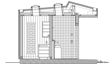
Sezione trasversale sui servizi
