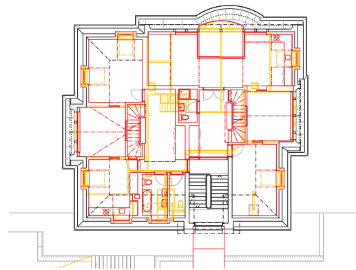
Grundriss Dachgeschoss, untere Ebene
