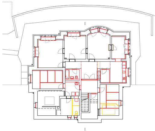
Grundriss 1. bis 3. OG
