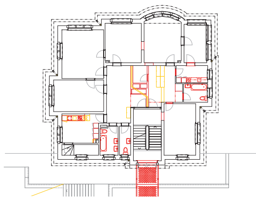
Grundriss Sockelgeschoss
