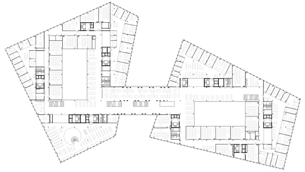
3. Obergeschoss
