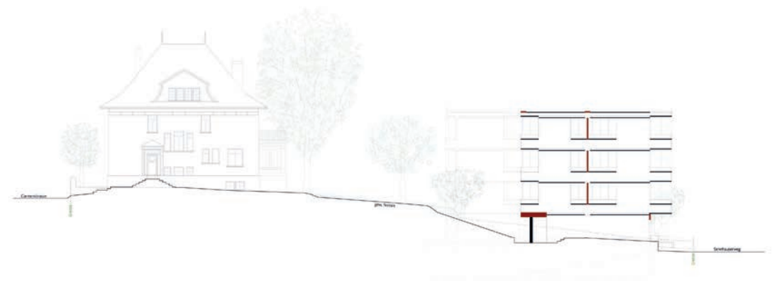
Ansicht 1:500
