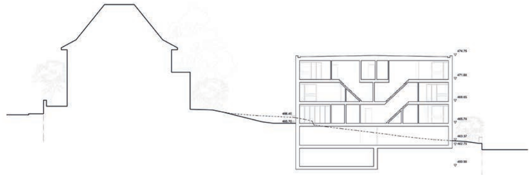
Schnitt 1:500
