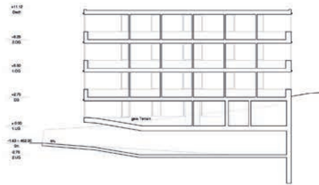
Schnitt und Ansicht 1:500
