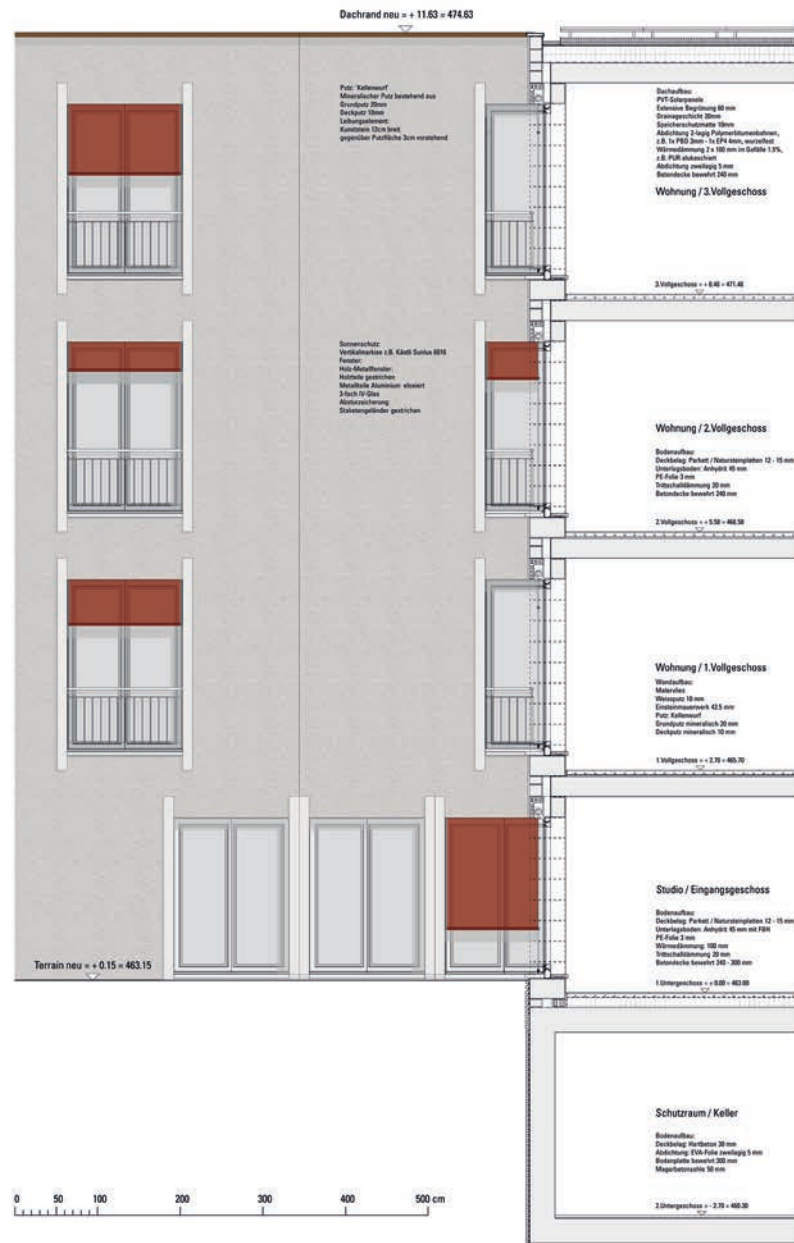
Detailschnitt und -ansicht 1:100
