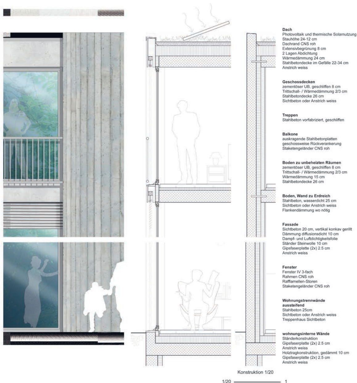
Detailschnitt und -ansicht 1:100
