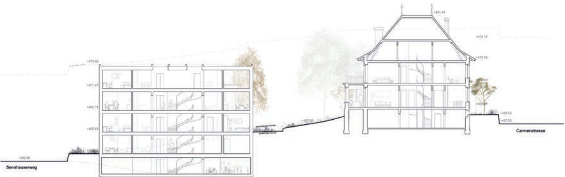
Schnitt 1:500
