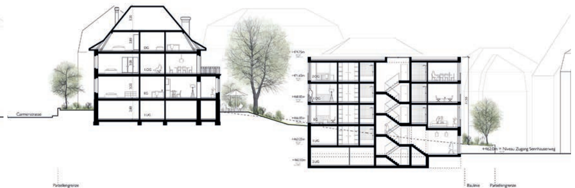
Schnitt 1:500
