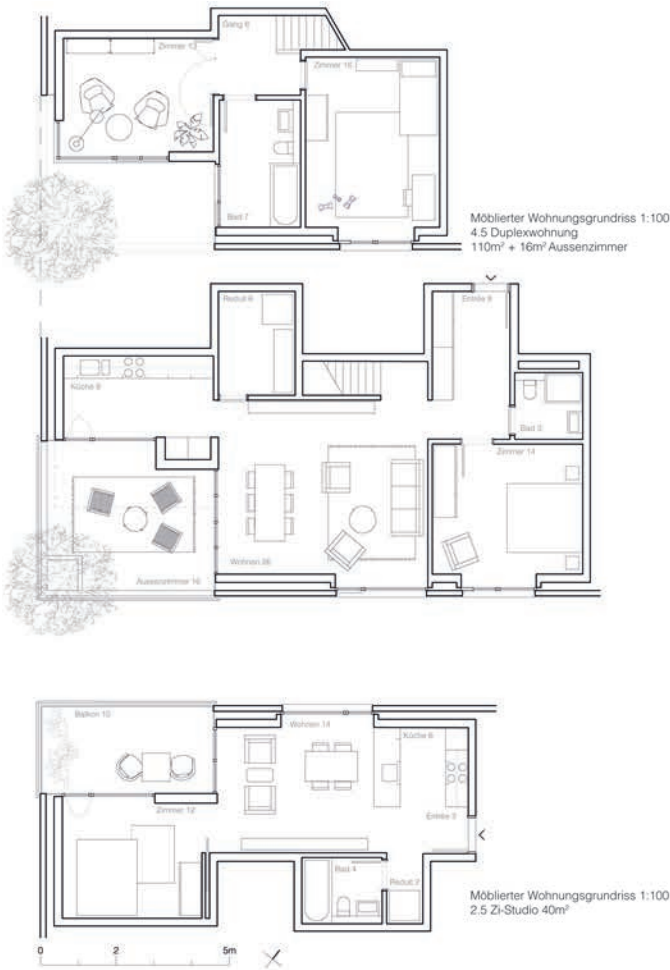
Grundriss Wohnungstypen 1:200
