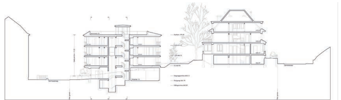
Schnitt 1:500
