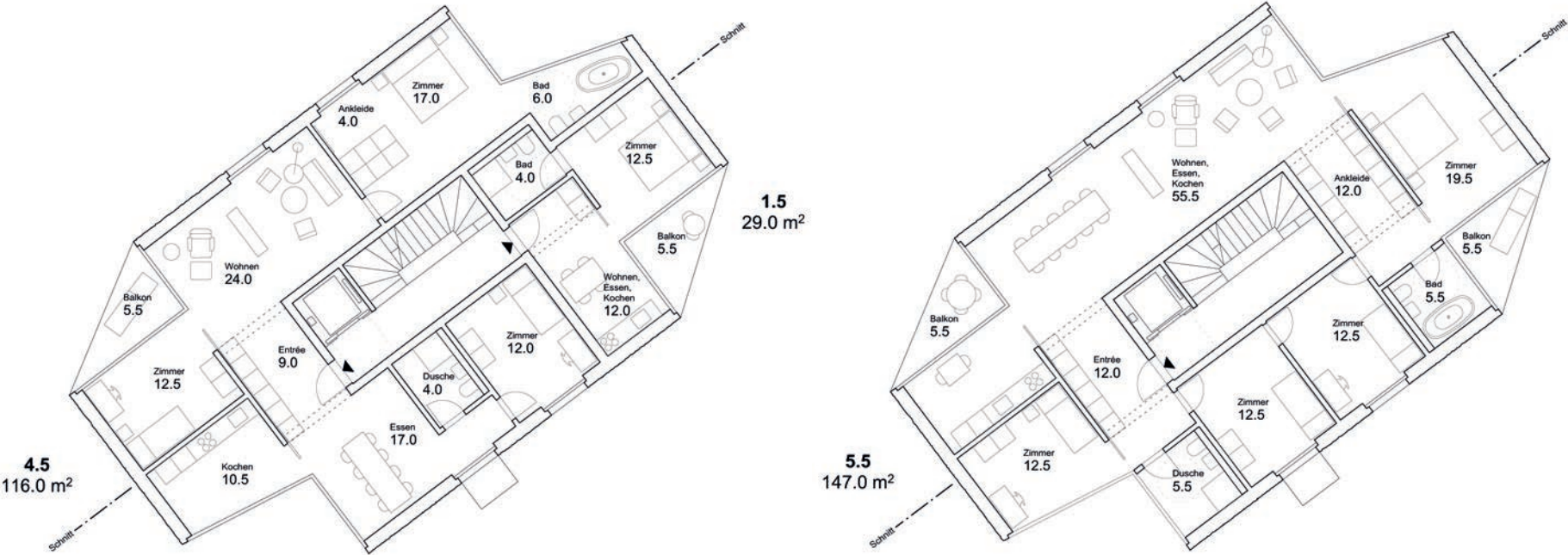
Grundrisse 1:200
