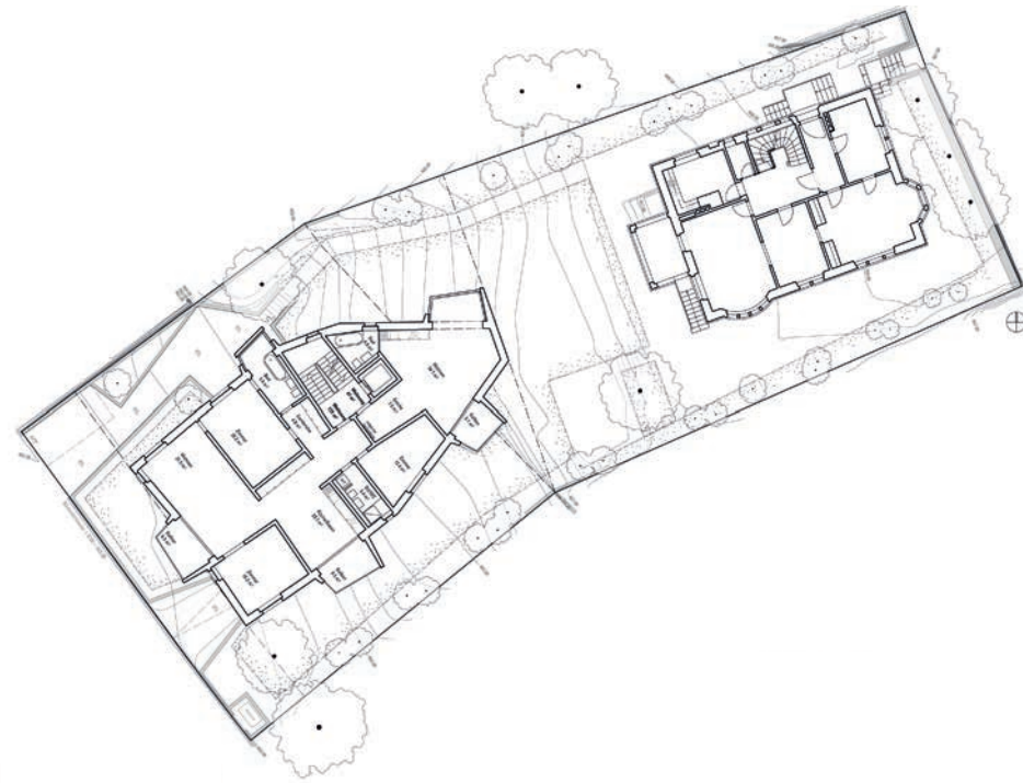
Erdgeschoss 1:500
