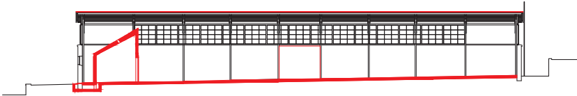
Sezione longitudinale
