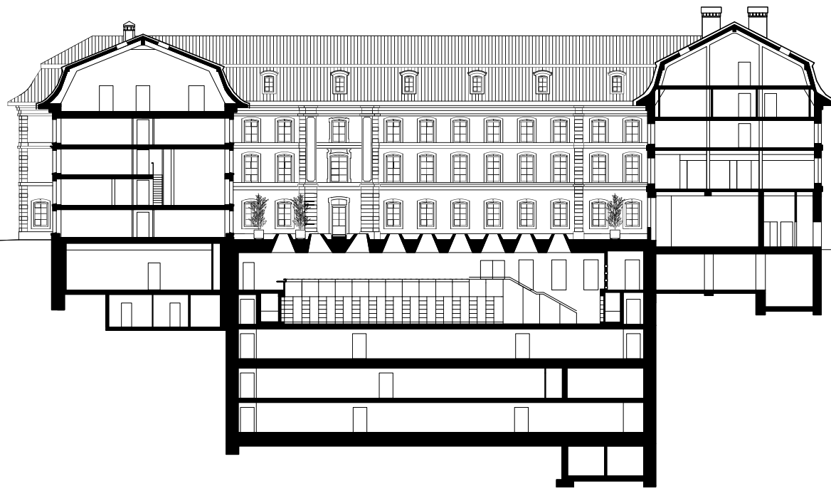
Längsschnitt Seitenflügel und Hof
