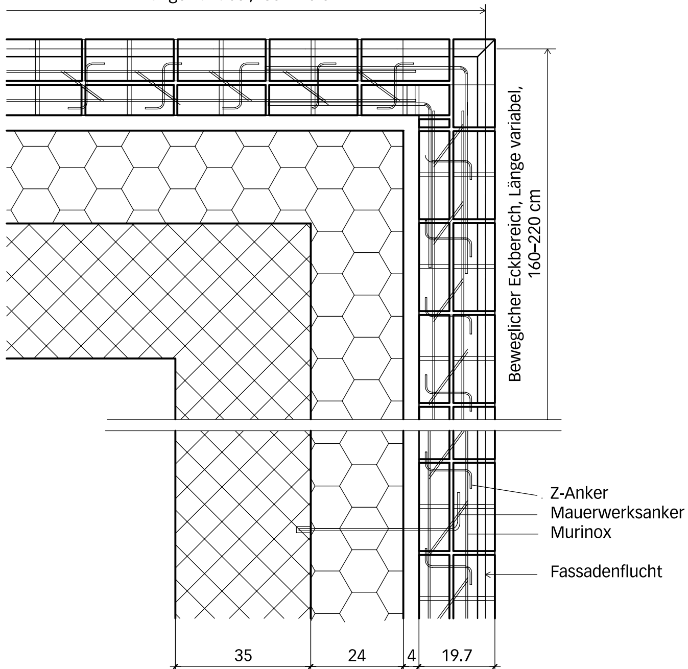
Beweglicher Eckbereich ohne Mauerwerksanker, Länge variabel, 160–220 cm
