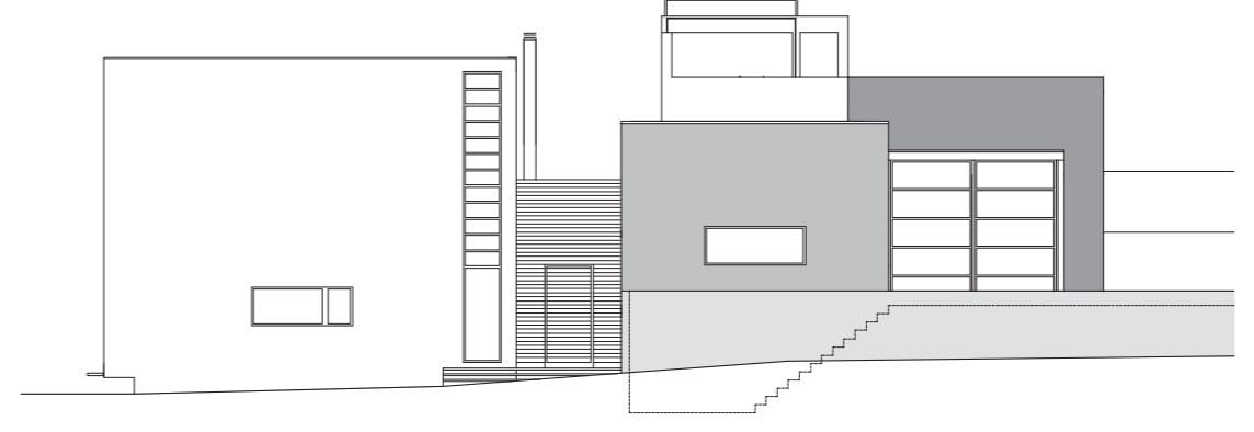
PROSPETTO SUD
