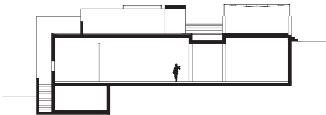
SEZIONE LONGITUDINALE
