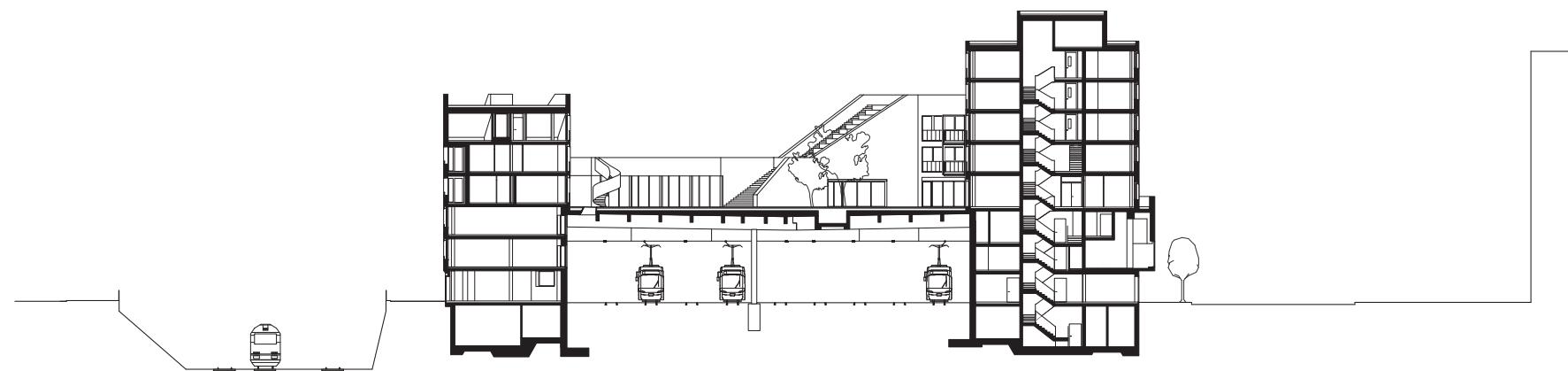
QUERSCHNITT TRAMHALLE 1:400
