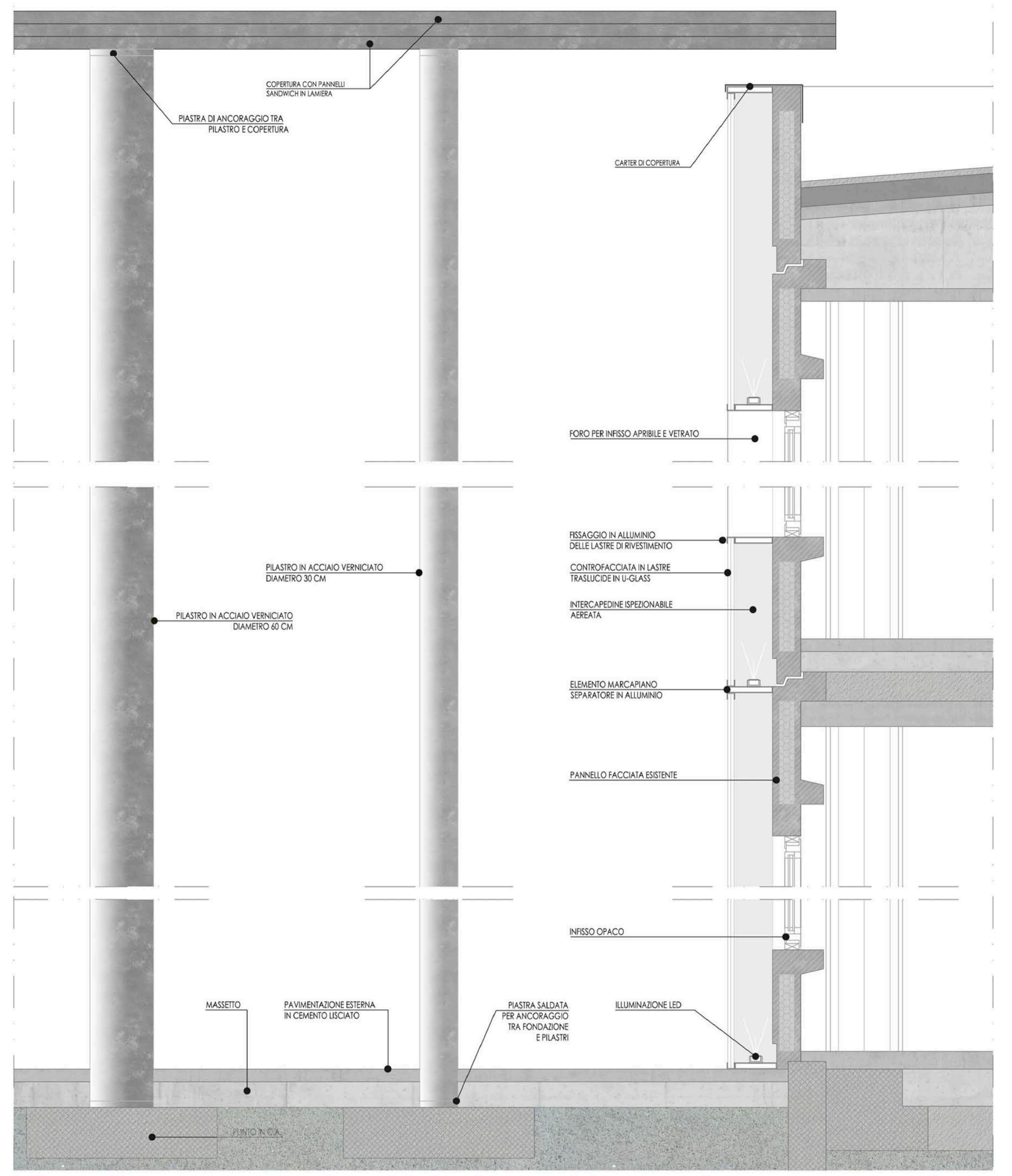
dettaglio 1:20
