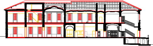
SEZIONE 1-1
