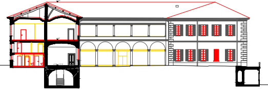
SEZIONE 2-2
