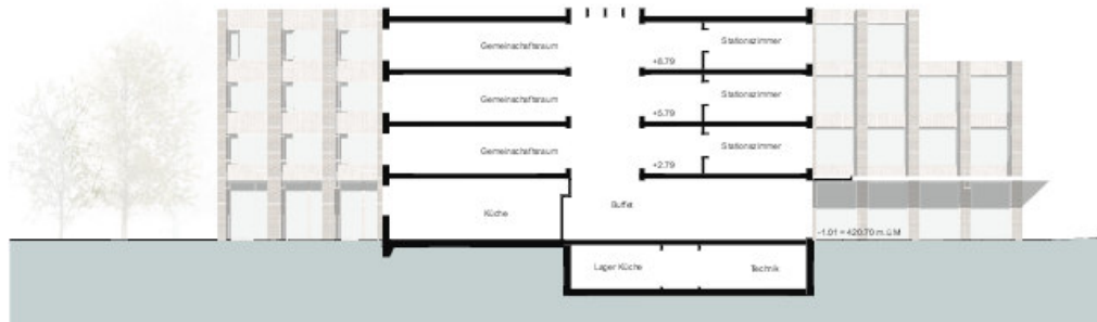
Schnitt A
