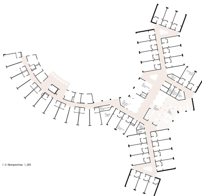
1. - 3. Obergeschoss
