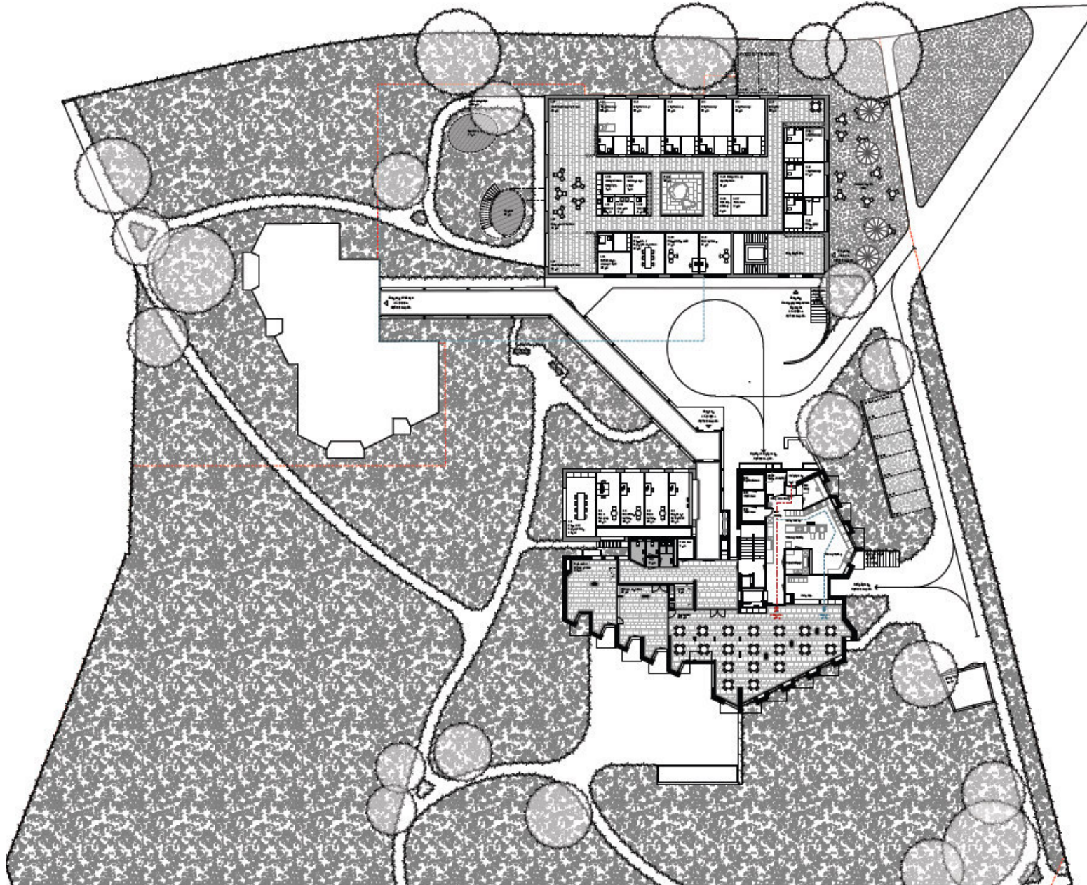
Erdgeschoss
