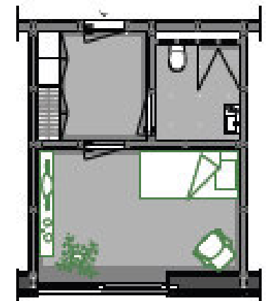
Grundriss Einbettzimmer
