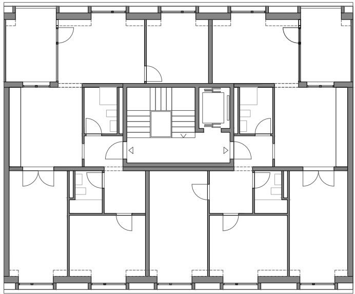
plan de l'attique, 1:200
