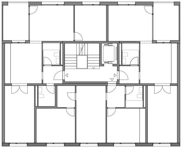
plan de surélévation, 1:200
