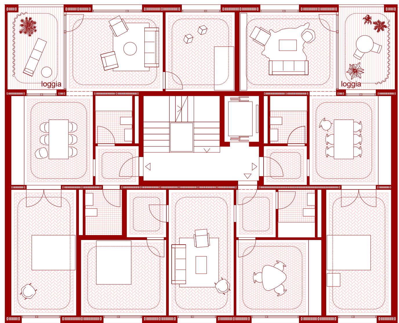
plan du niveau 5-6, 1:100
