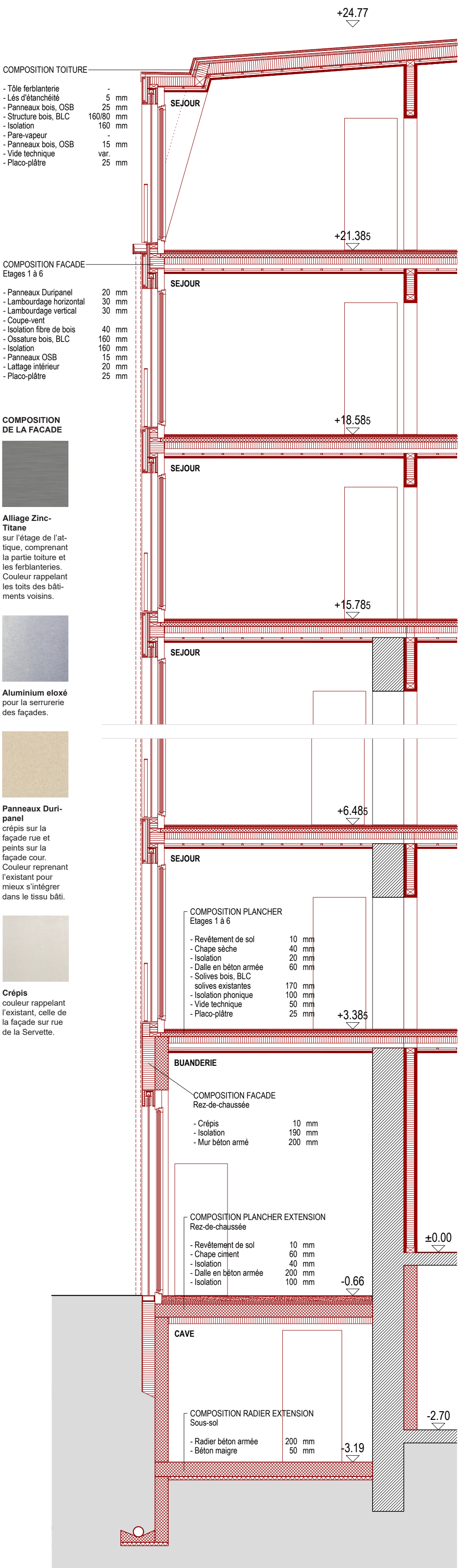
coupe détail constructif, 1:50
