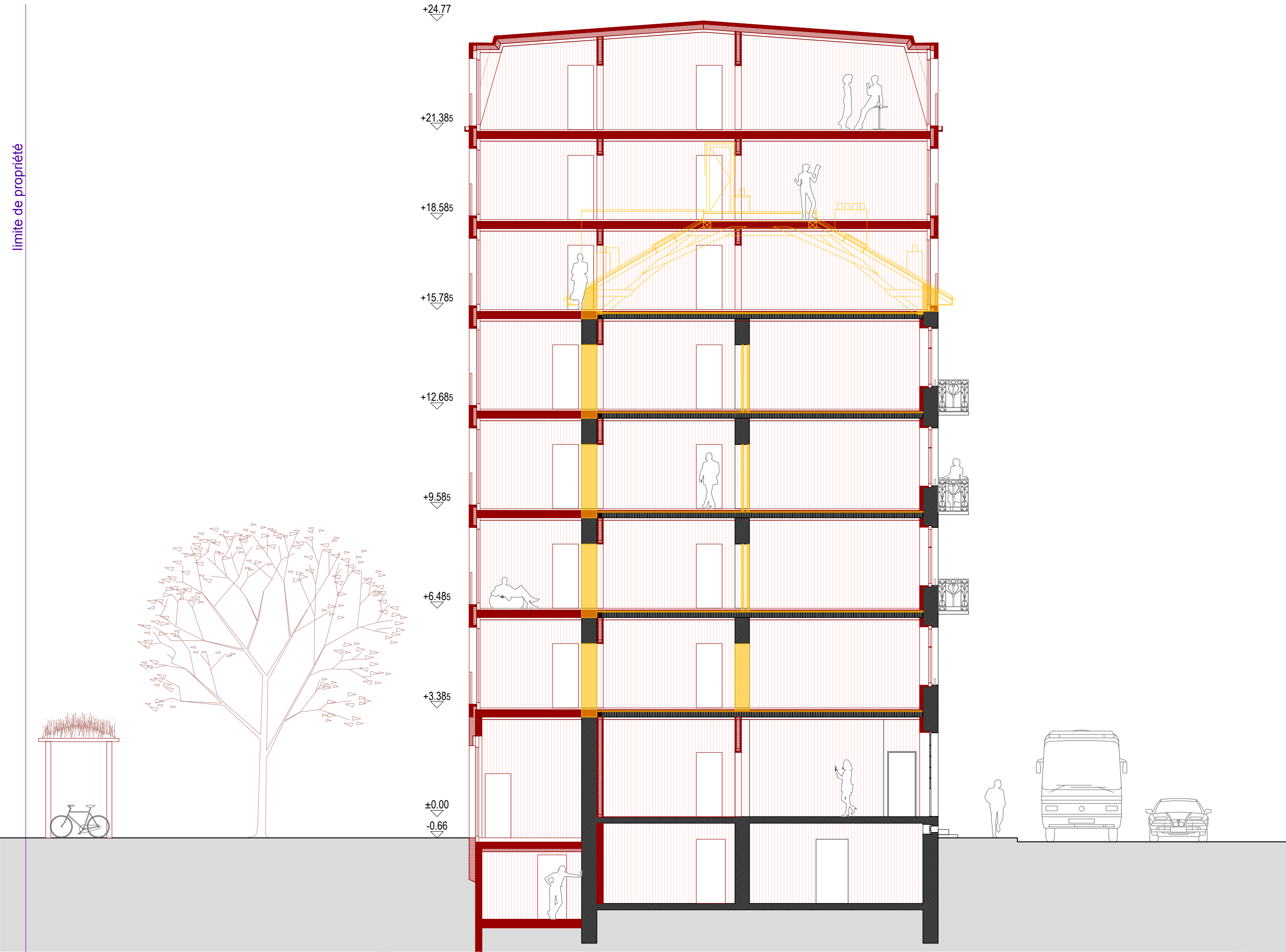
coupe transversale, 1:100
