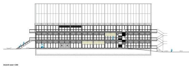
Ansicht west 1:200
