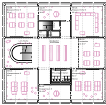
2. Obergeschoss 1.200, Mittelschule
