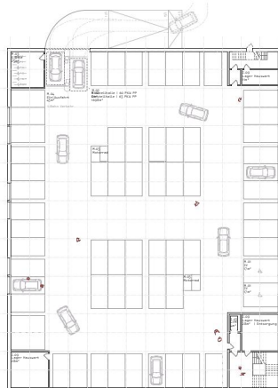
UNTERGESCHOSS
