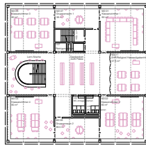
3. Obergeschoss 1.200, Mittelschule
