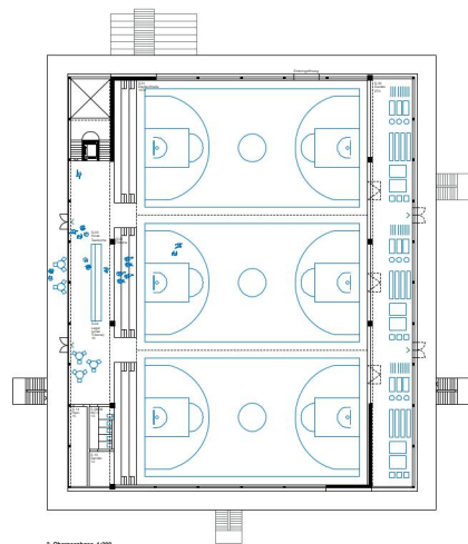
2. Obergeschoss 1:200
