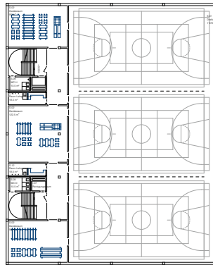
2. Obergeschoss 1.200
