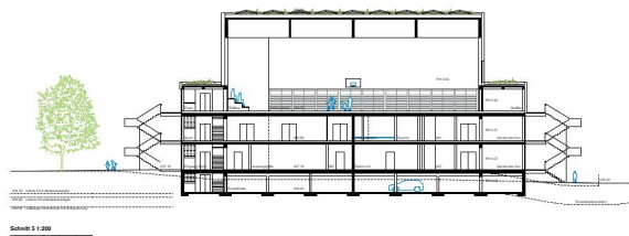
Schnitt 1:1:200
