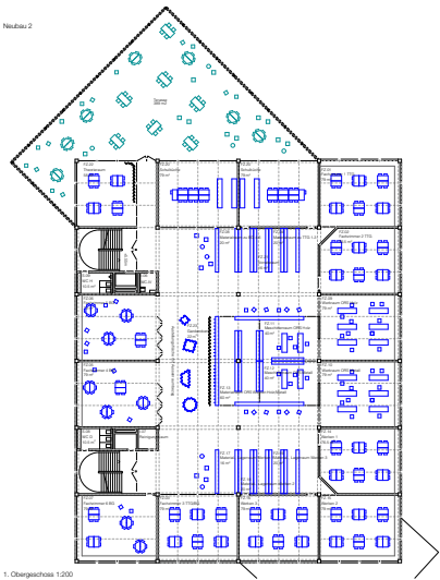
1. Obergeschoss 1.200
