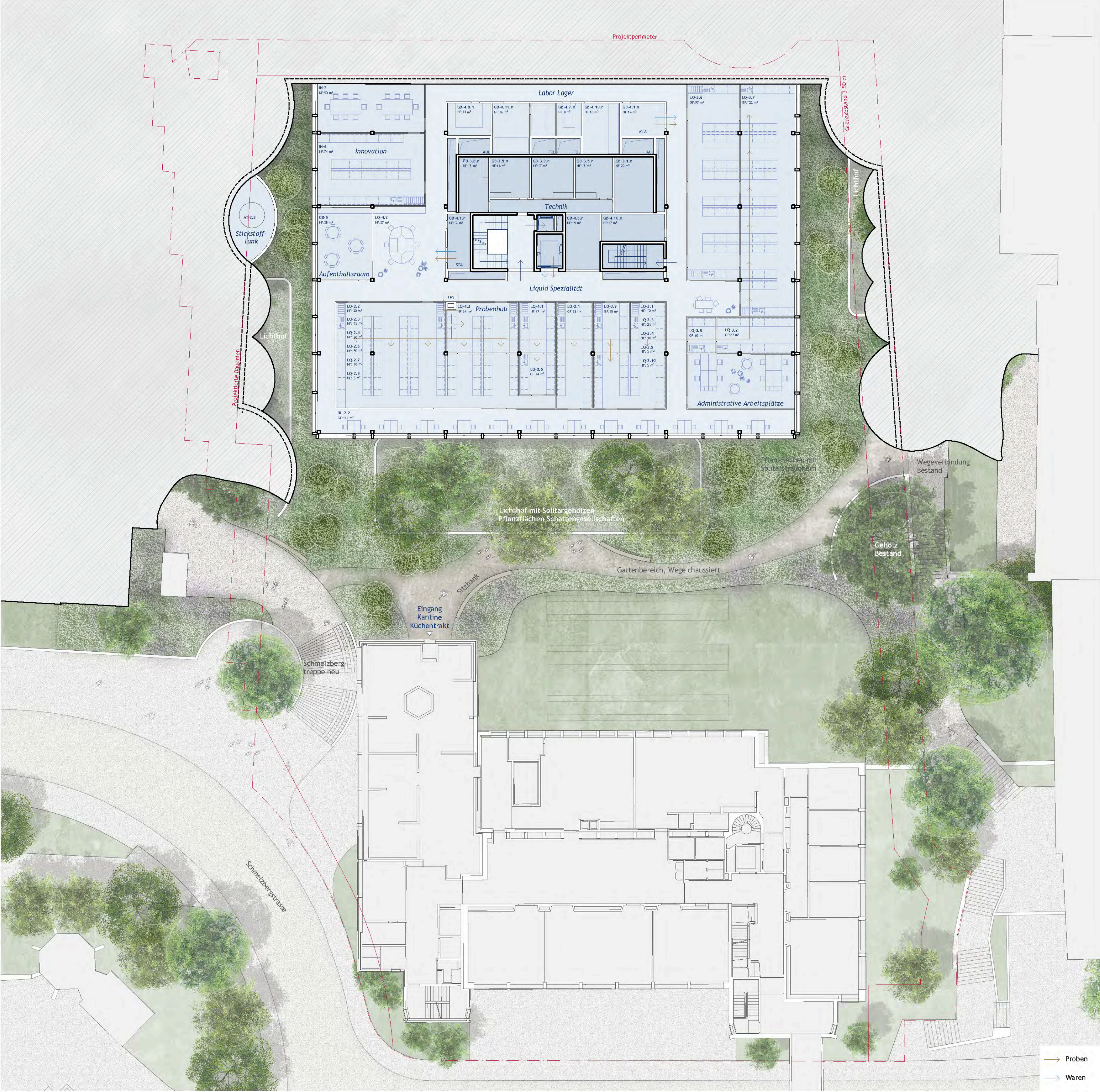
Geschoß B, Met. 1:200
