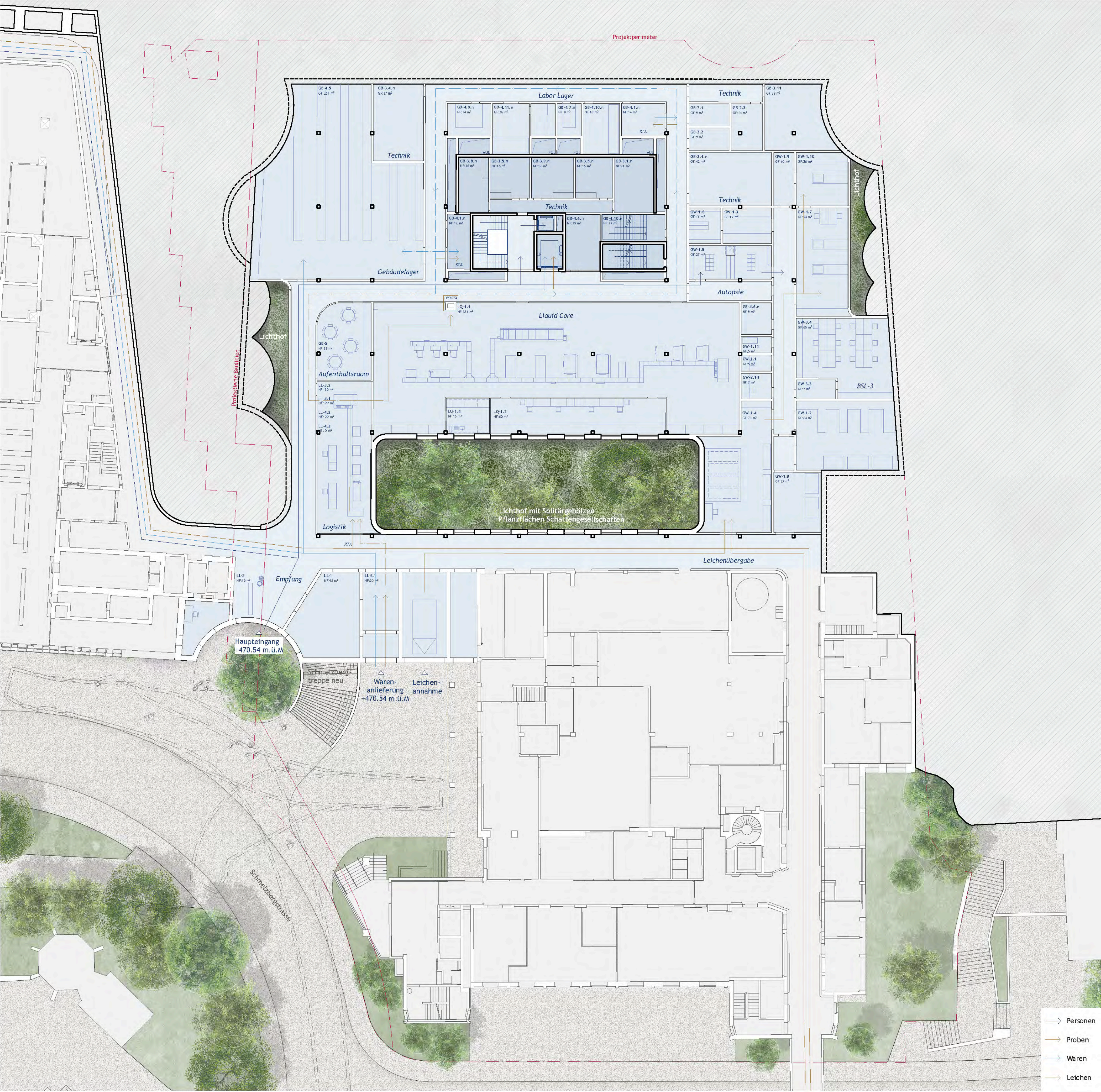
Geschoß A, Met. 1:200
