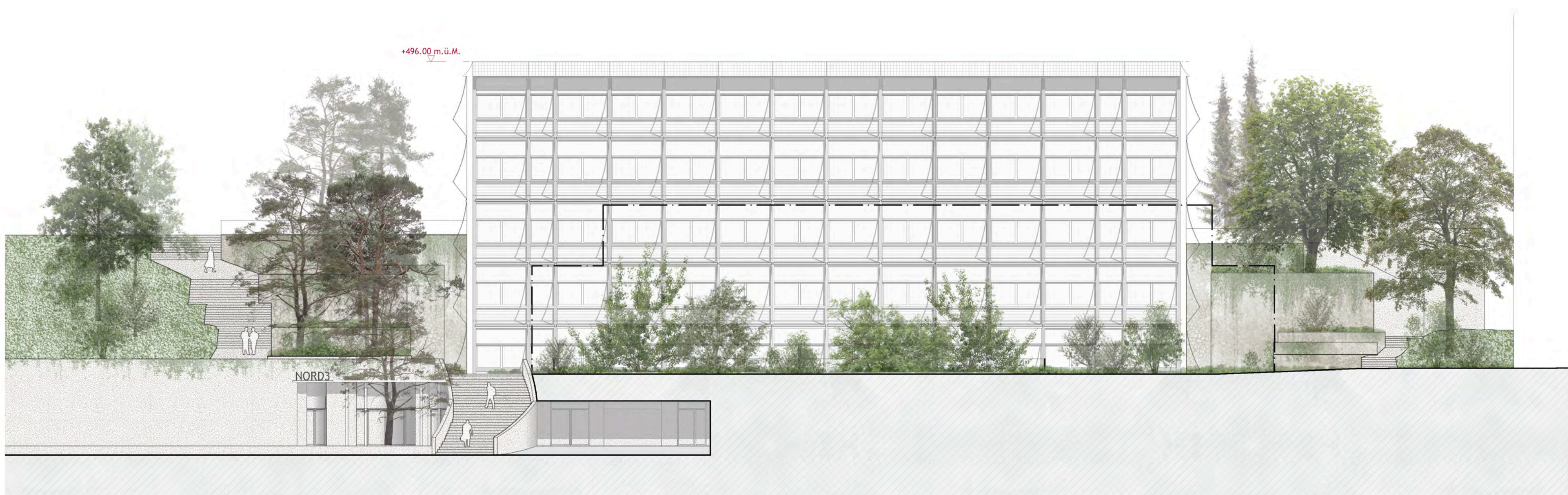
Ansicht Süd, Mst. 1:200
