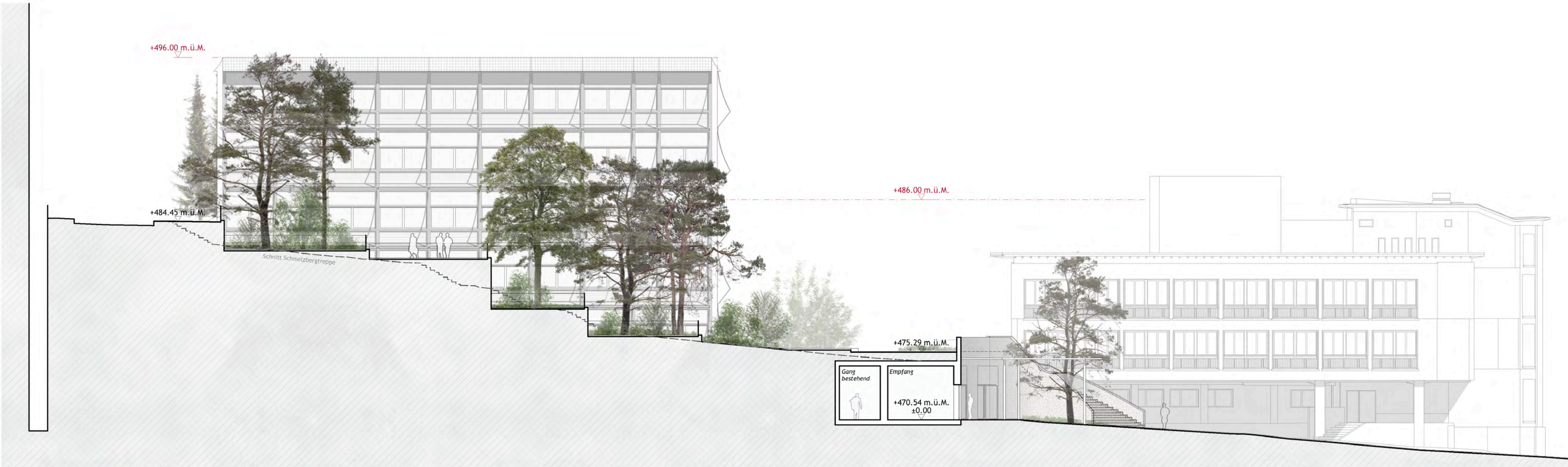
Schnitt Schmelzbergstrasse, Mst. 1:200
