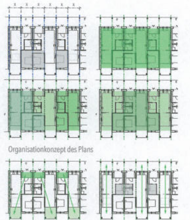
Flexibilität durch Schlafzimmern / von 1.5-Zimmer bis 4.5-Zimmer Wohnungen
