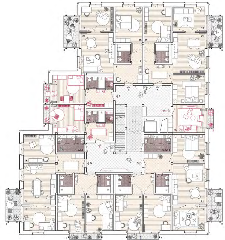
Regelgeschoss – Einteilung A
