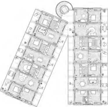
Regelgeschoss
