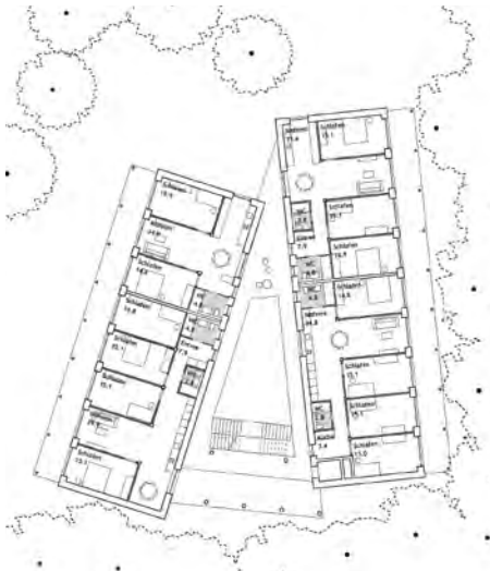
2. Obergeschoss
