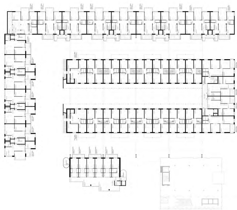
1. Obergeschoss 1:200
