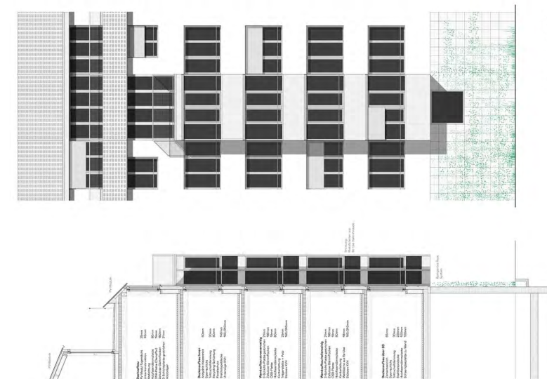
Konstruktionscheit Winkelbau Ansicht Isenstraße 150
