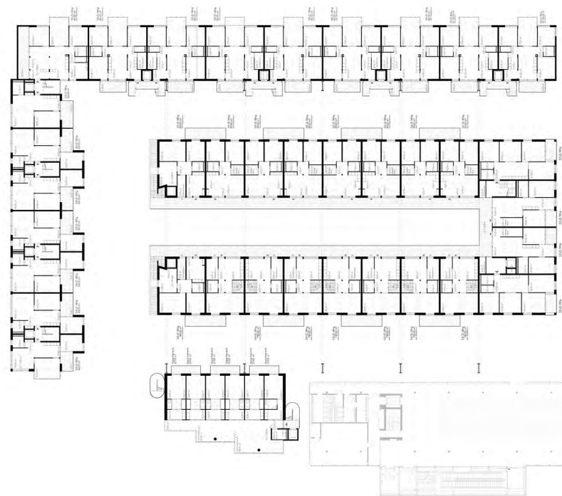
2. Obergeschoss 1:200
