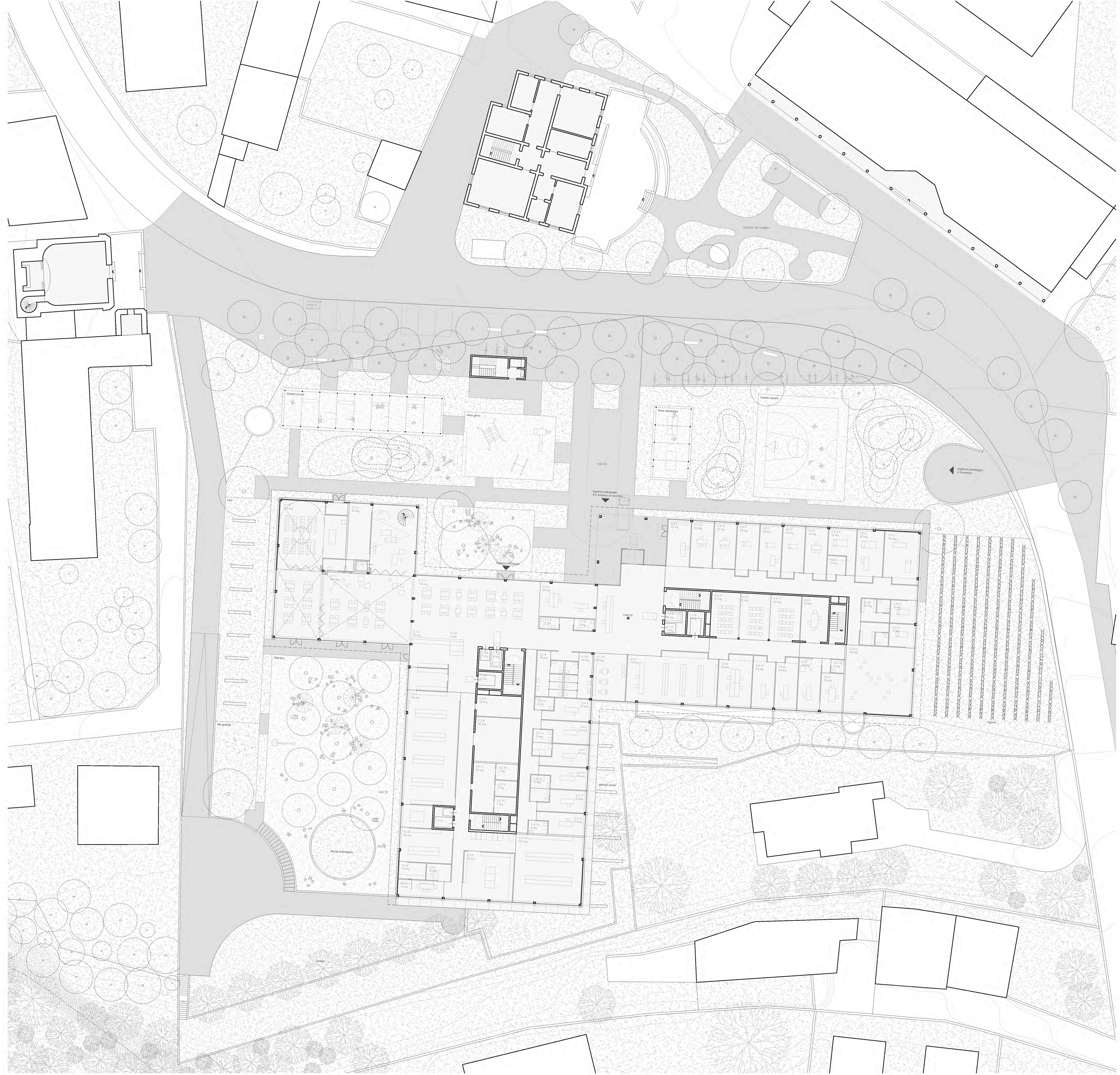
Pianta del piano terra, scala 1:200
