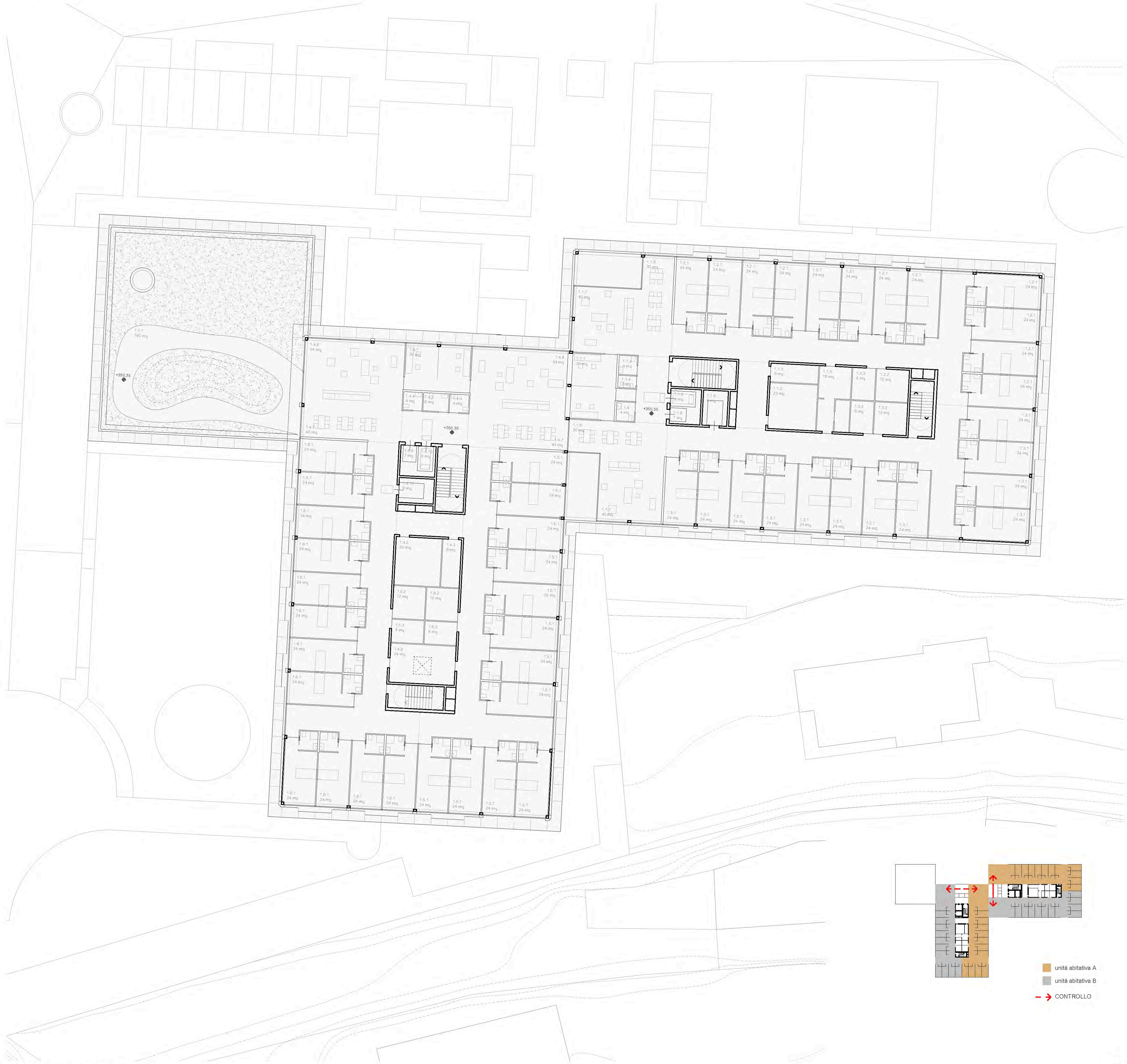
Pianta secondo piano, scala 1:200
