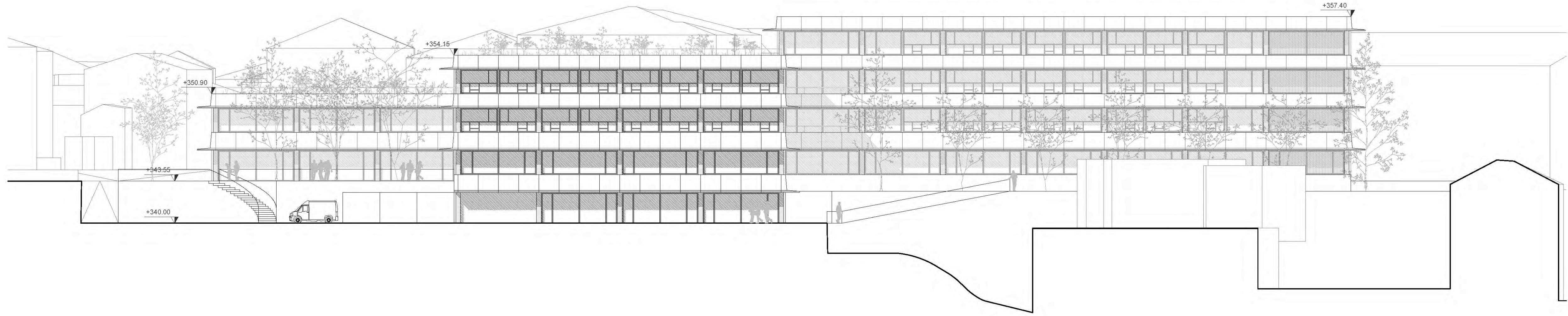
Vista sud-ovest, scala 1:200
