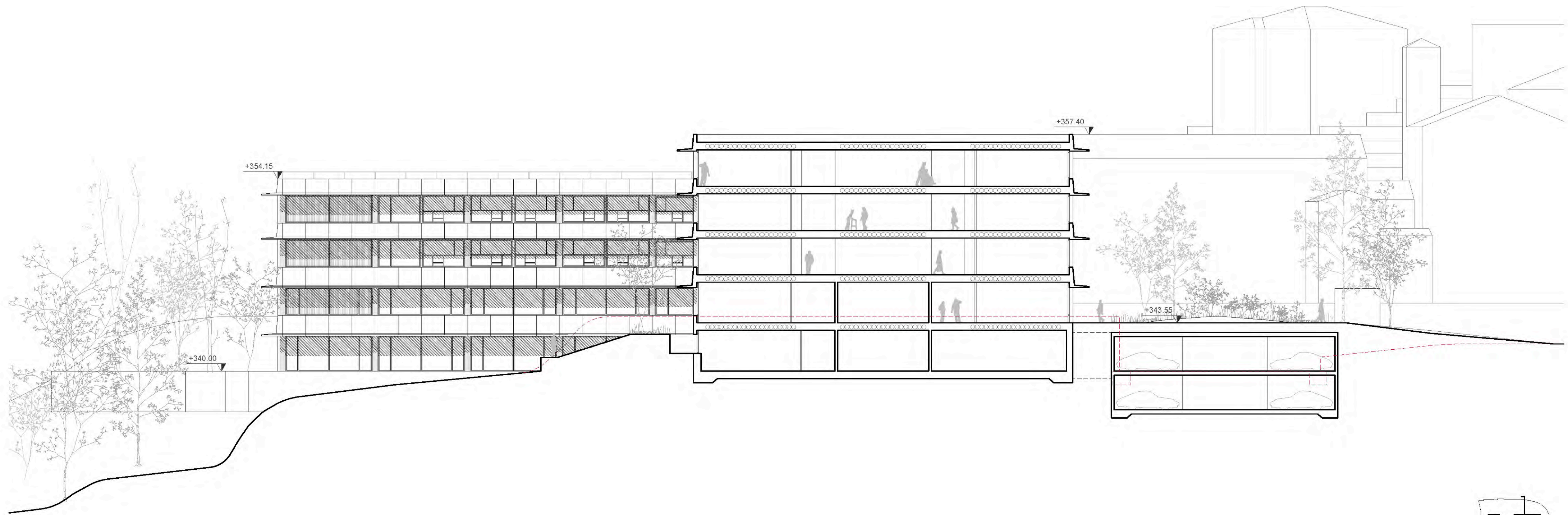
Sezione CC', scala 1:200
