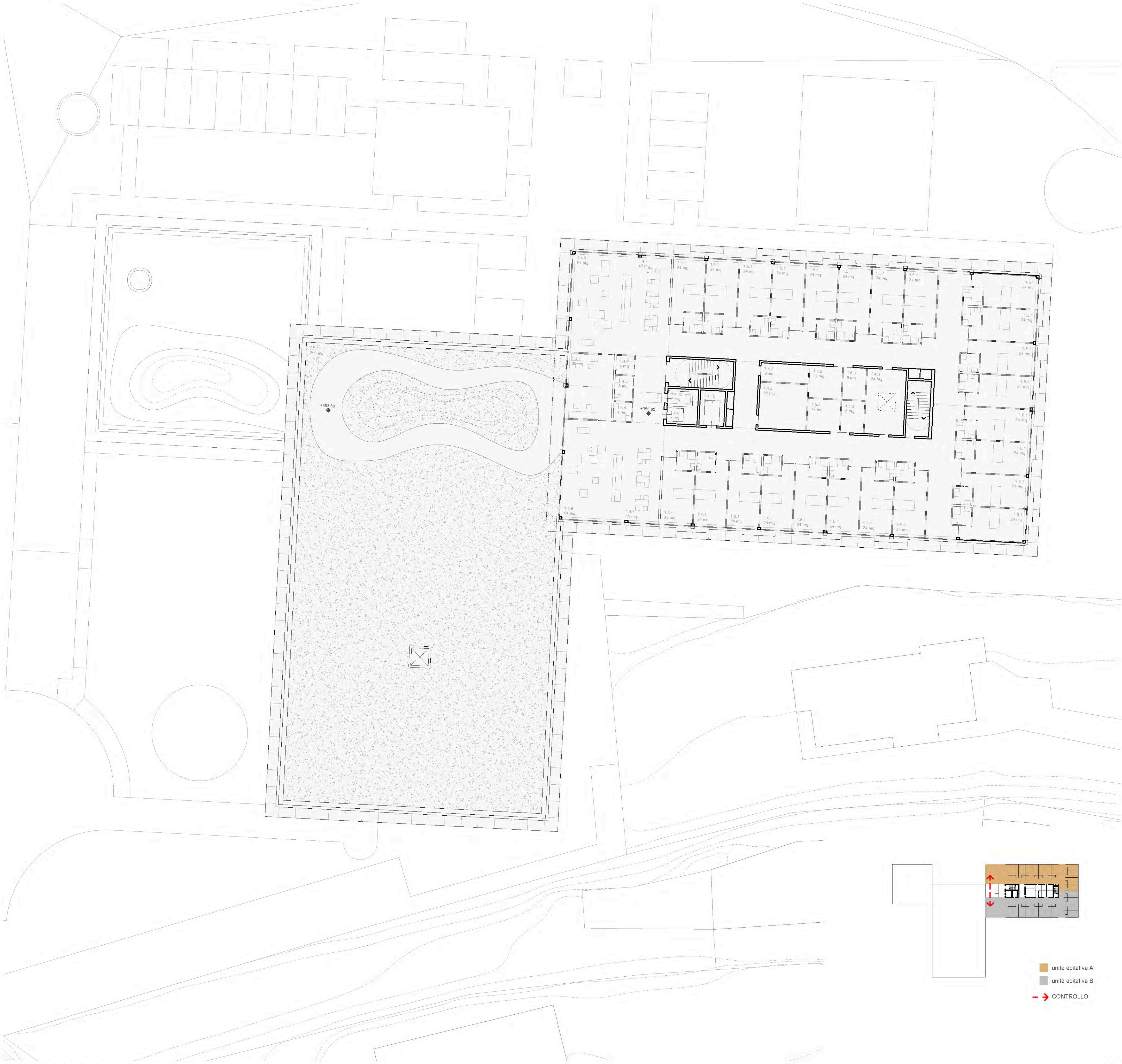
Pianta terzo piano, scala 1:200
