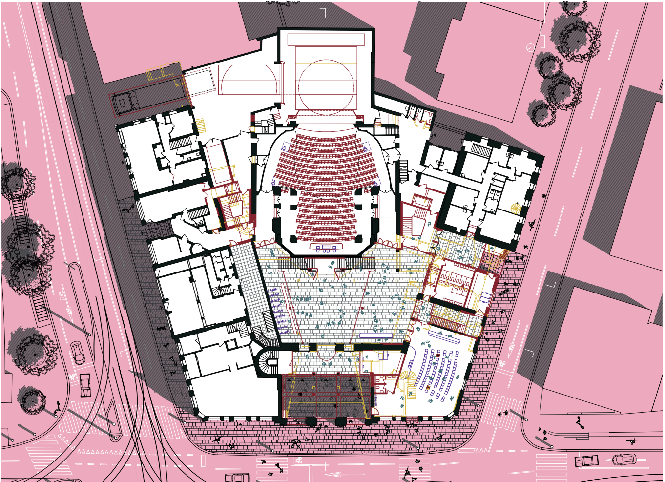
Grundriss Erdgeschoss 1:600
