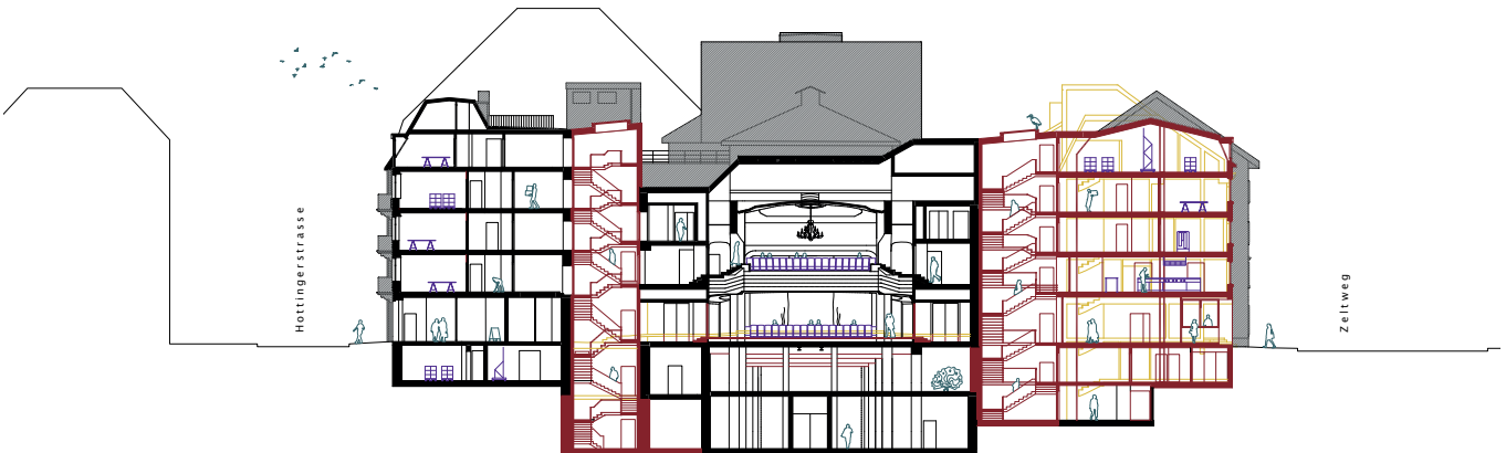
Schnitt 1:600
