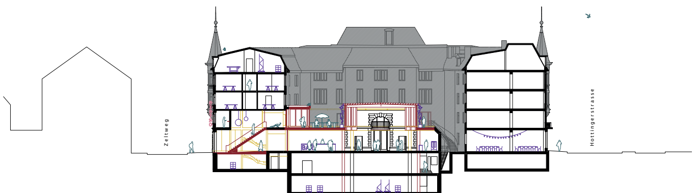
Schnitt 1:600
