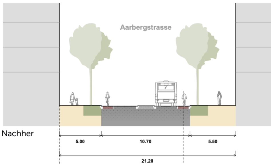
Schnitt Aarbergstrasse
