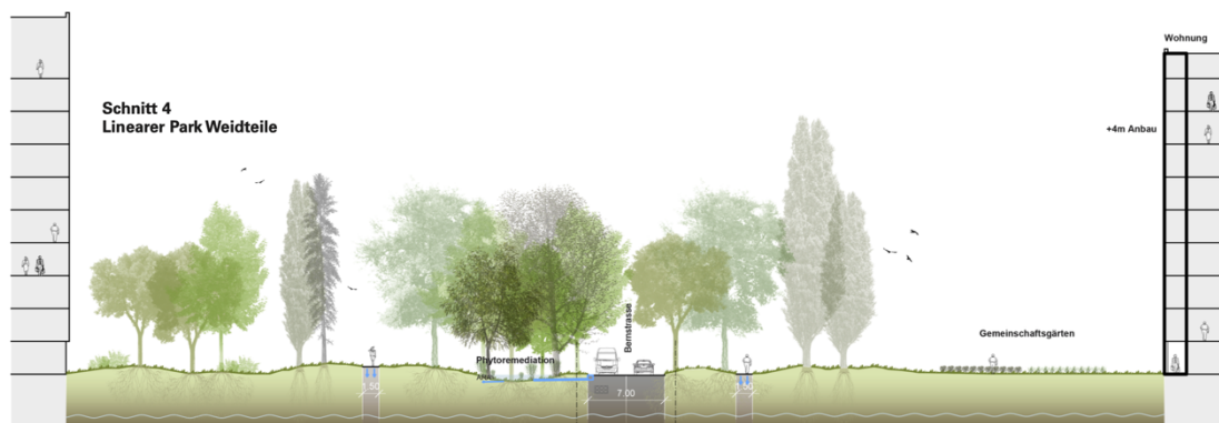
Schnitt Bernstrasse
