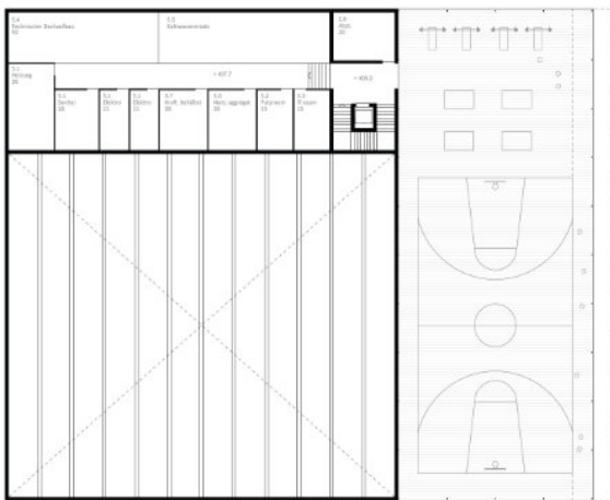
2. Obergeschoss
