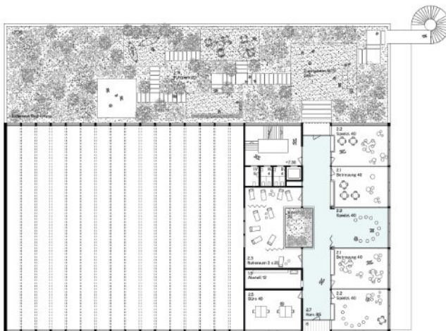
2. Obergeschoss
