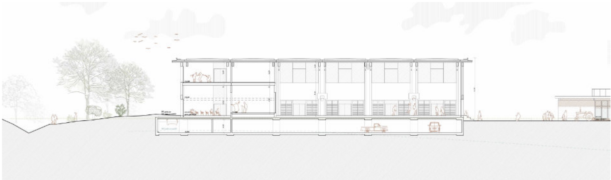
Längsschnitt MZH
