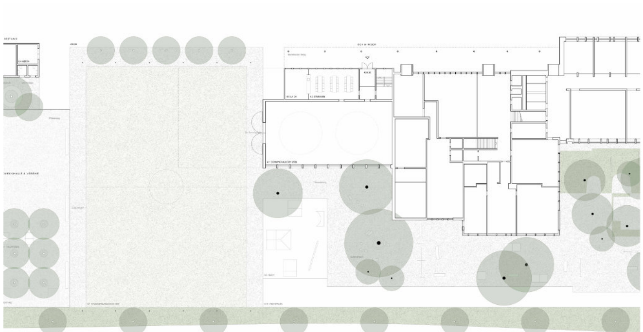
Erdgeschoss Schwinghalle
