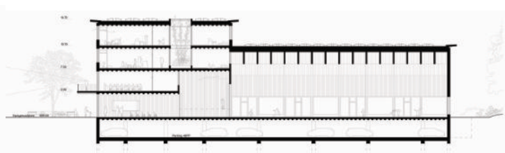
Längsschnitt Erweiterung
