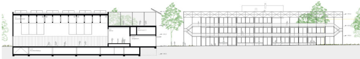
Schnitt A (Mehrzweckhalle)
