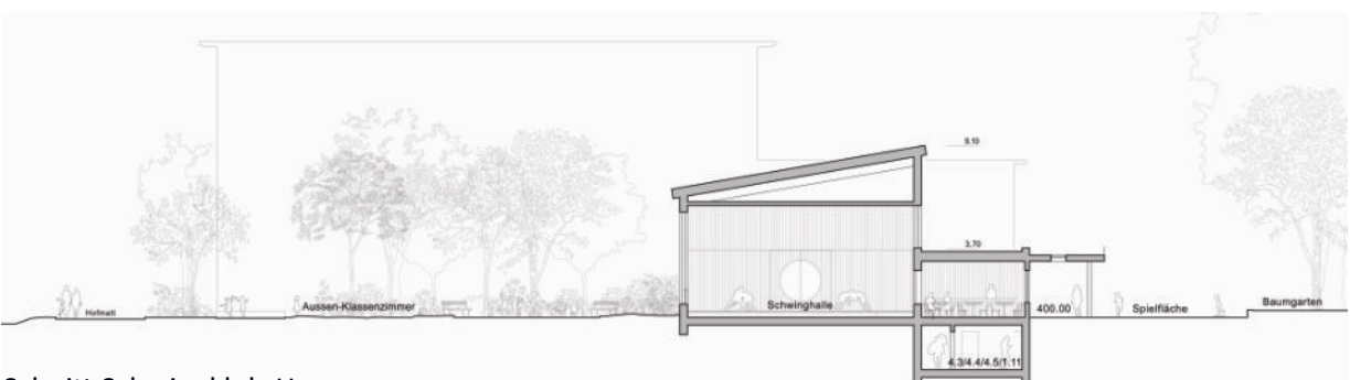
Schnitt Schwingklub-Haus
