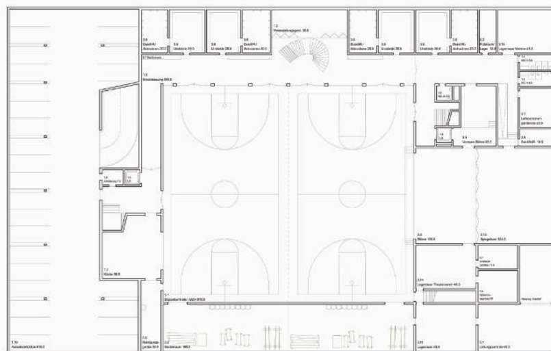
Untergeschoss MZH
