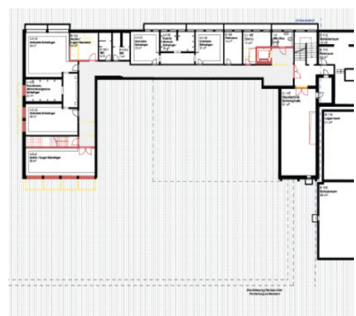
Untergeschoss Trakt 2
