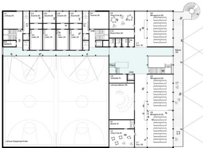
1. Obergeschoss
