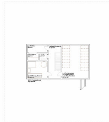
Untergeschoss MTS
