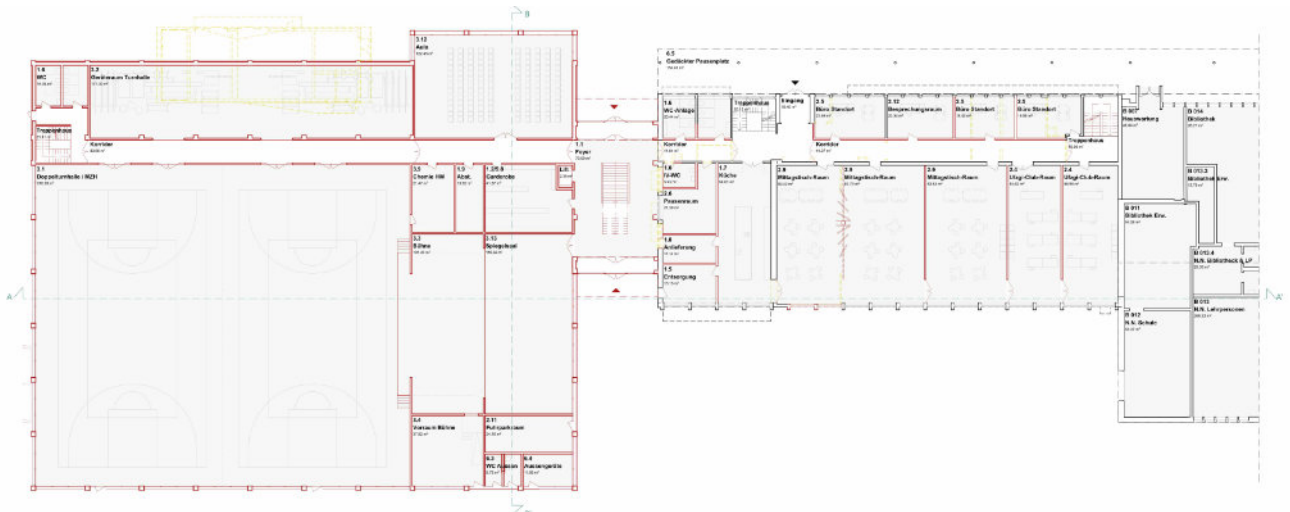
Erdgeschoss
