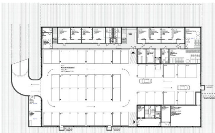
Untergeschoss Neubau
