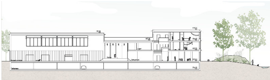
Schnitt 1
