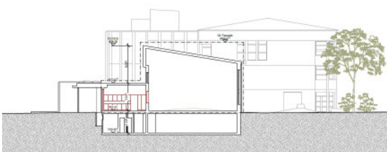
Schnitt B
