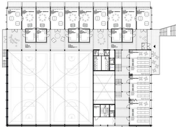
1. Obergeschoss
