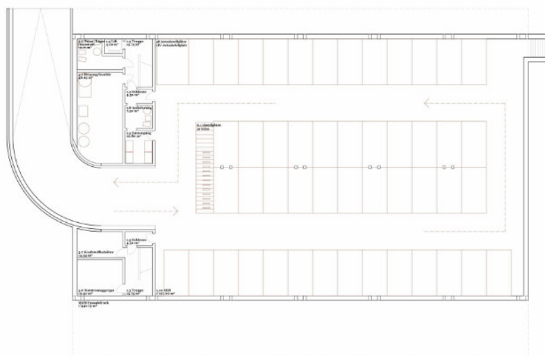
Untergeschoss MZH
