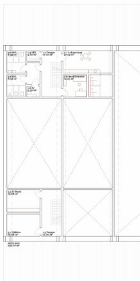
Obergeschoss MZH
