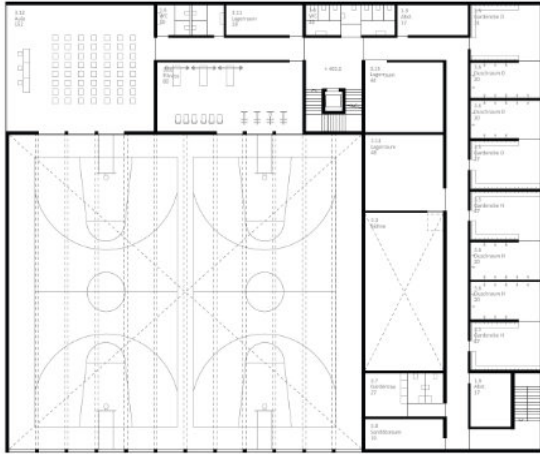
1. Obergeschoss
