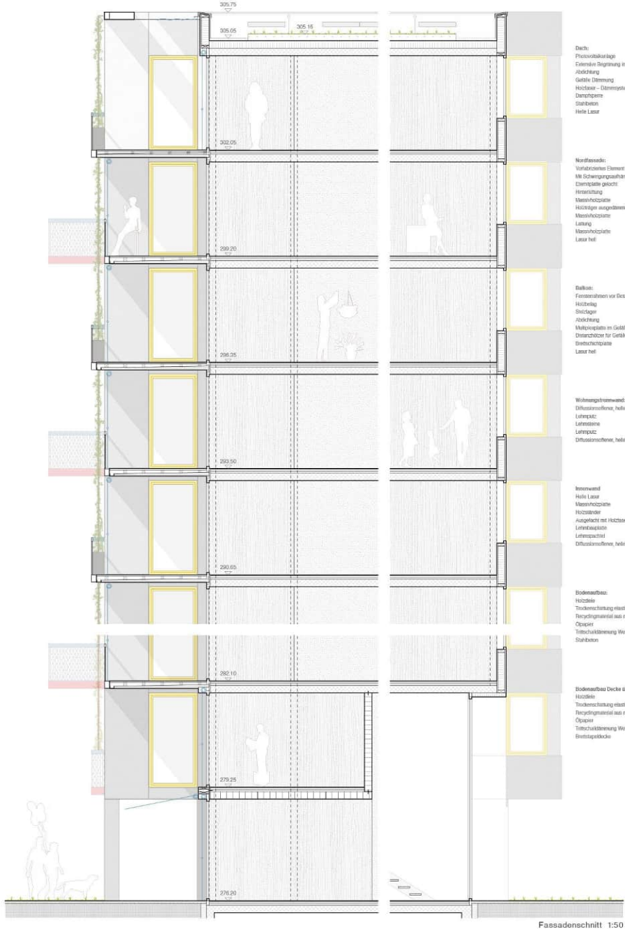
Fassadenschnitt 1:50
