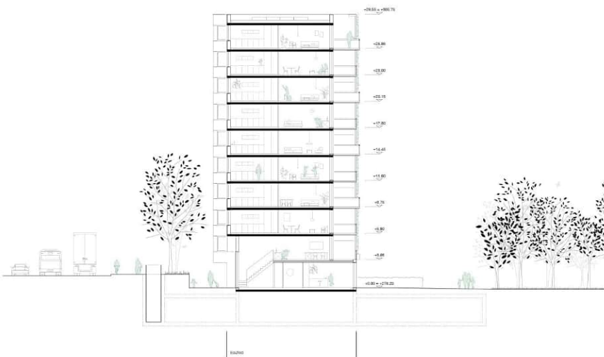
Schnitt CC 1:200
