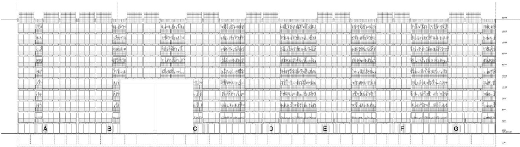
Südfassade 1:200
