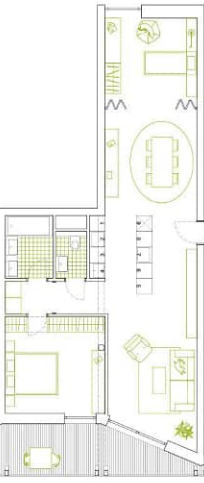
Wohnungstyp 3.5g ZL-WHG 1:100
