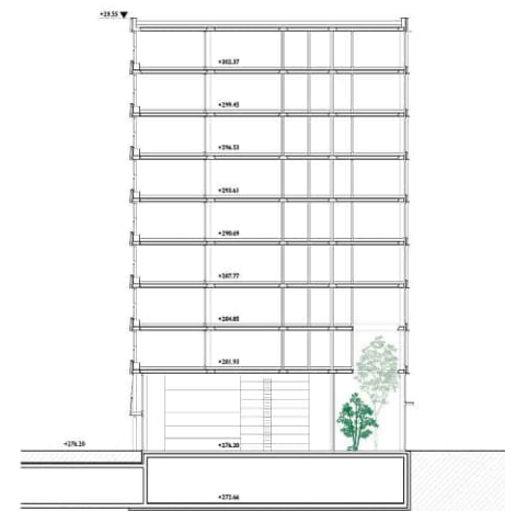
Querschnitt A - 1:200
