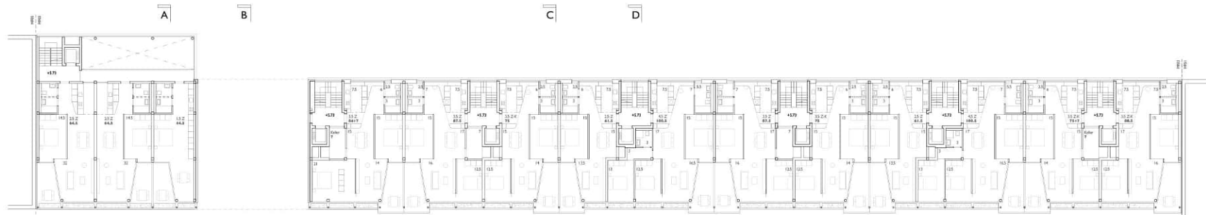
2.OG - 4.OG - 1:200
