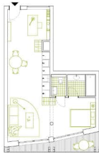
Wohnungstyp 2.5 ZL-WHG 1:100
