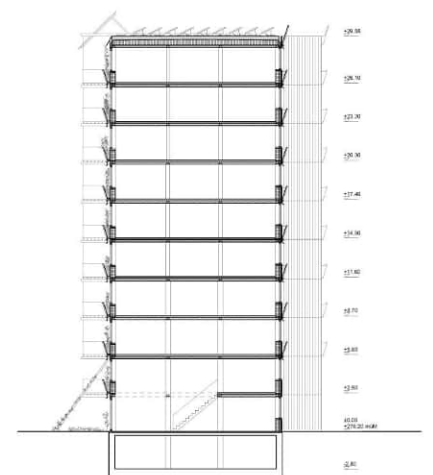
Querschnitt Gewerbe EG 1:200
