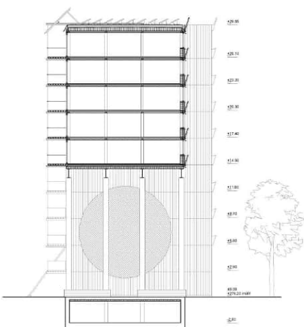
Querschnitt 2 1:200
