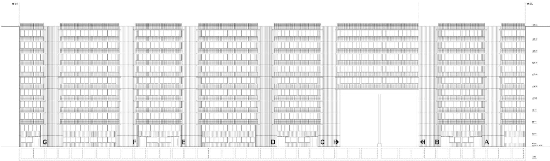
Nordfassade 1:200
