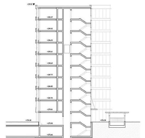
Querschnitt D - 1:200
