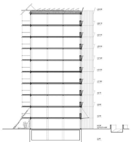
Querschnitt 3 1:200
