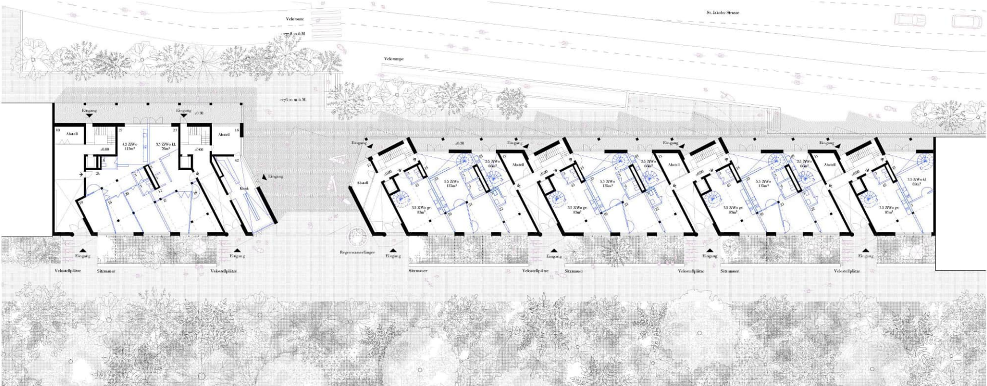
Situation, Erdgeschoss mit Ausbau 1: 200
