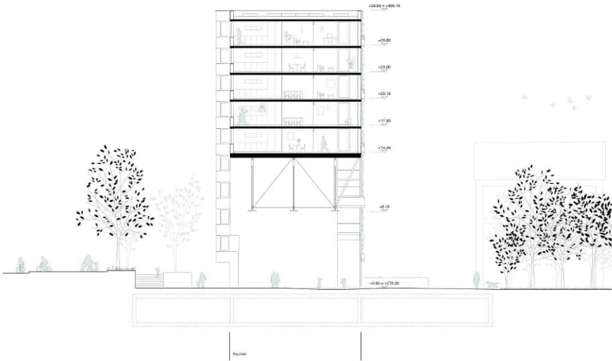
Schnitt BB 1:200
