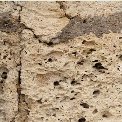
Porosität als Lebensgrundlage für Vegetation: Tuffstein
