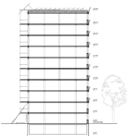
Querschnitt 1 1:200
