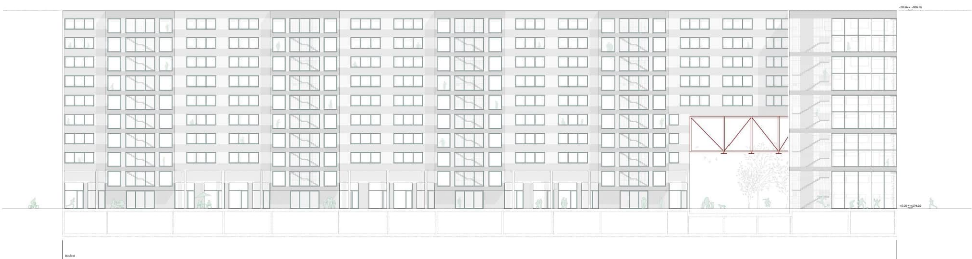
Ansicht Nord 1:200
