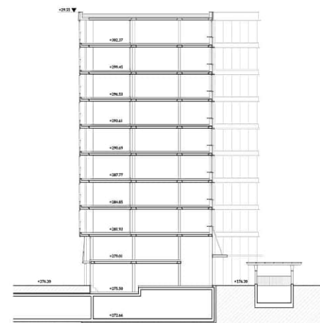
Querschnitt C - 1:200
