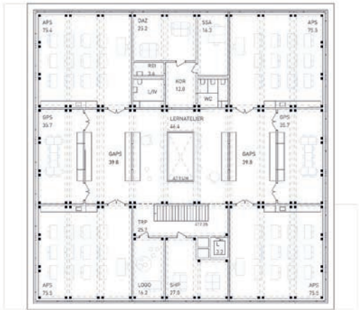
Grundriss 2. Obergeschoss 1:500
