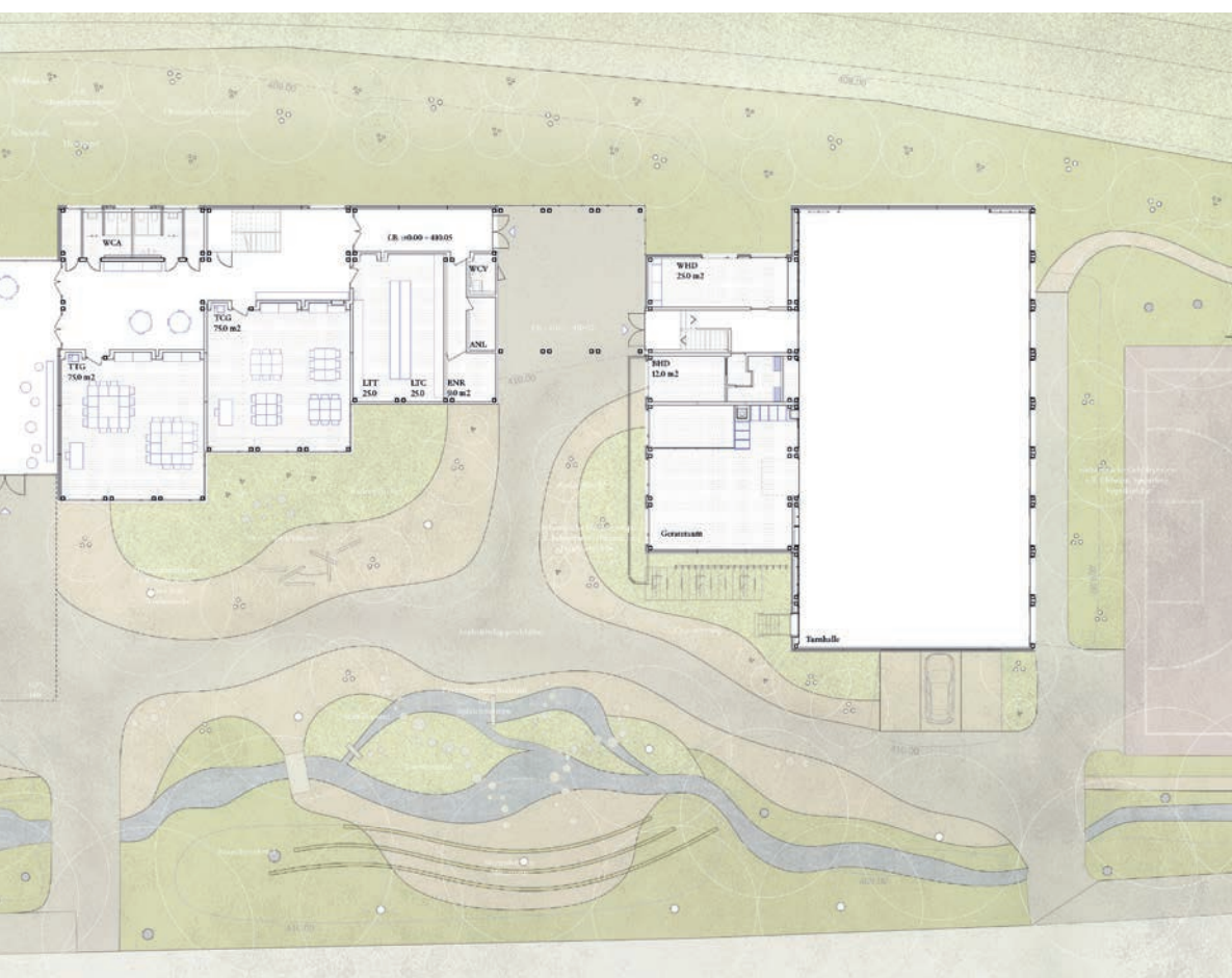
Grundriss Erdgeschoss 1:500
