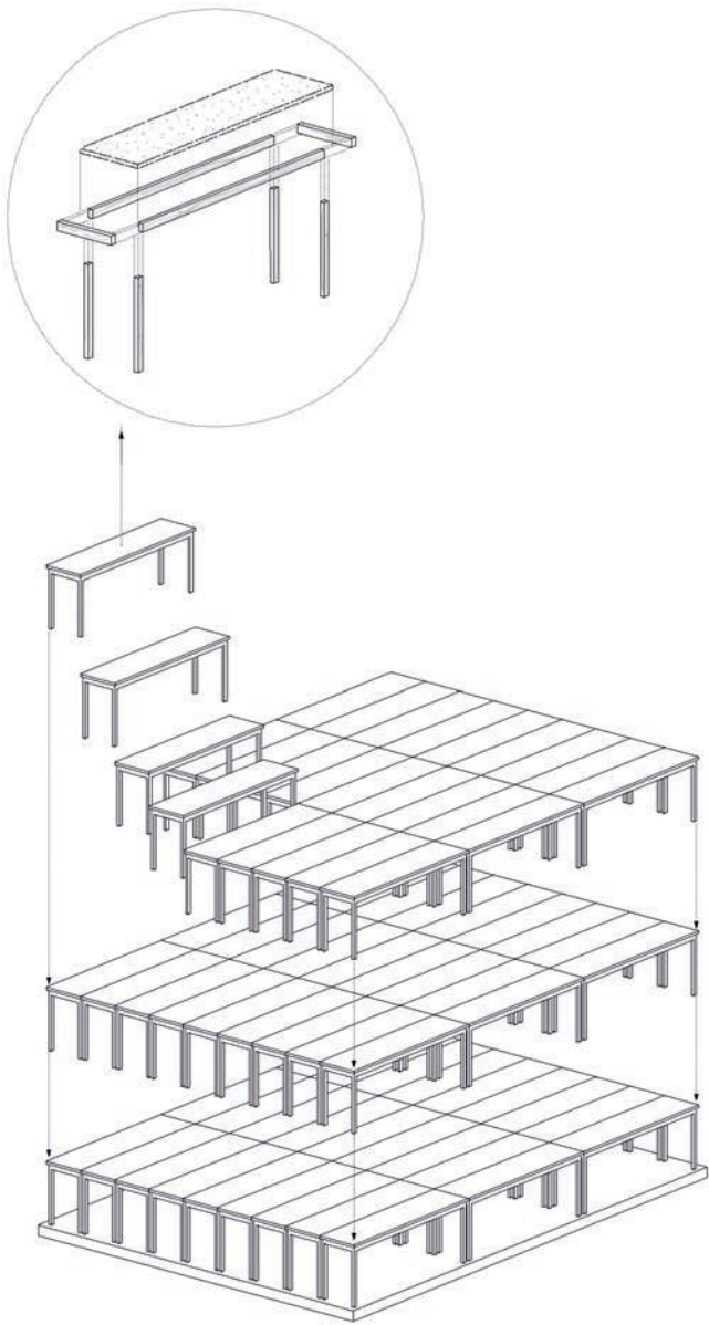
Axonometrie Statik
