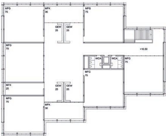
Erweiterung Grundriss 3.Obergeschoss 1:500
