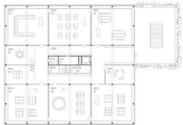
Erweiterung Grundriss 3.Obergeschoss 1:500
