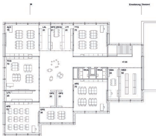
Grundriss 2.Obergeschoss 1:500
