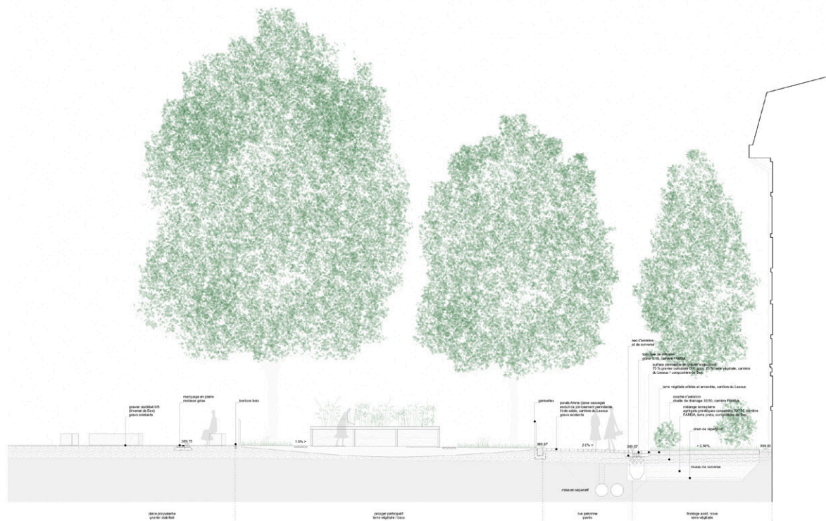
Coupe de détail, frontage passif - potager, 1:50
