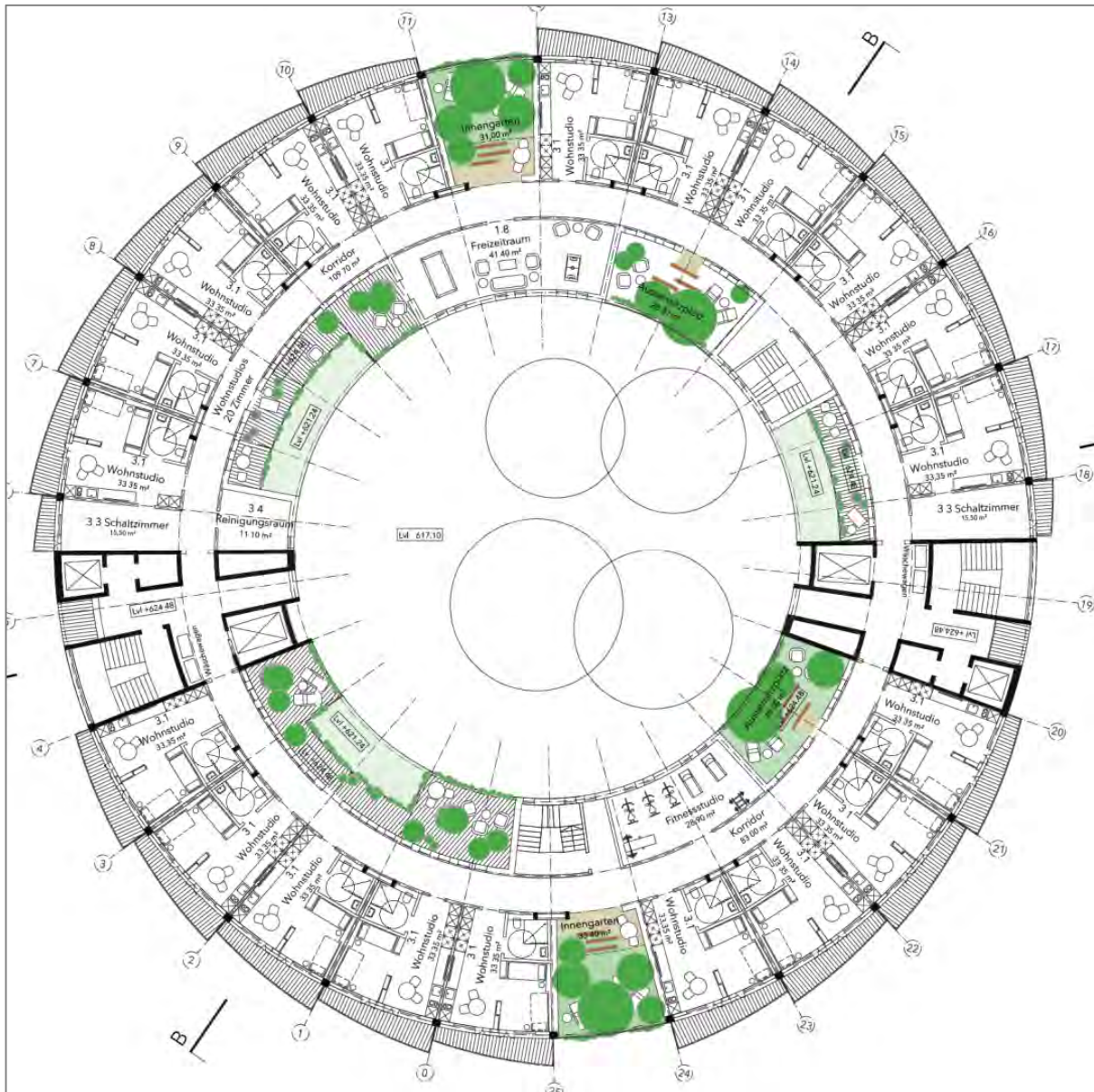
Grundriss 2. Obergeschoss
