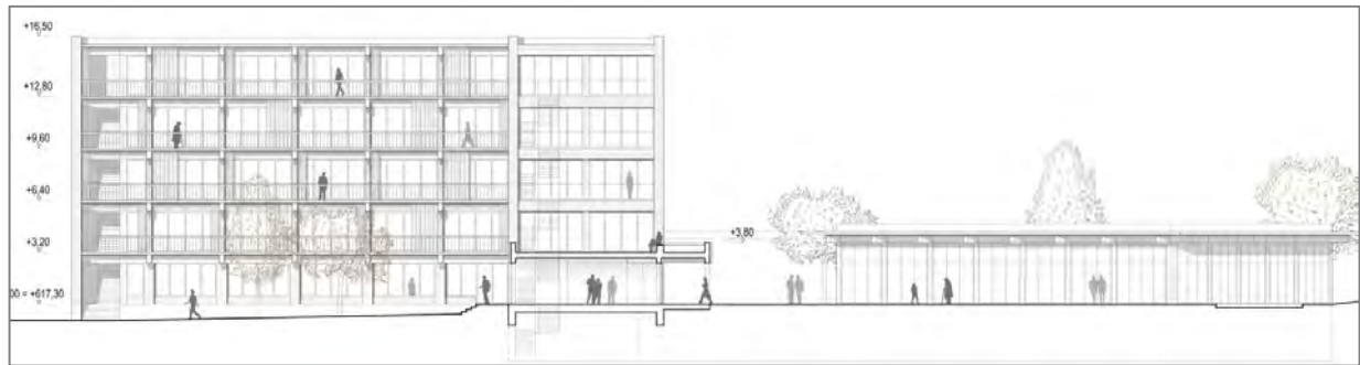
Ansicht Nord-Ost
