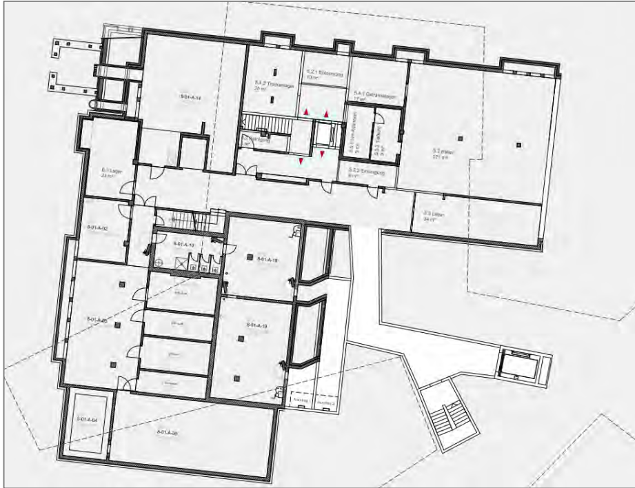
Grundriss Untergeschoss
