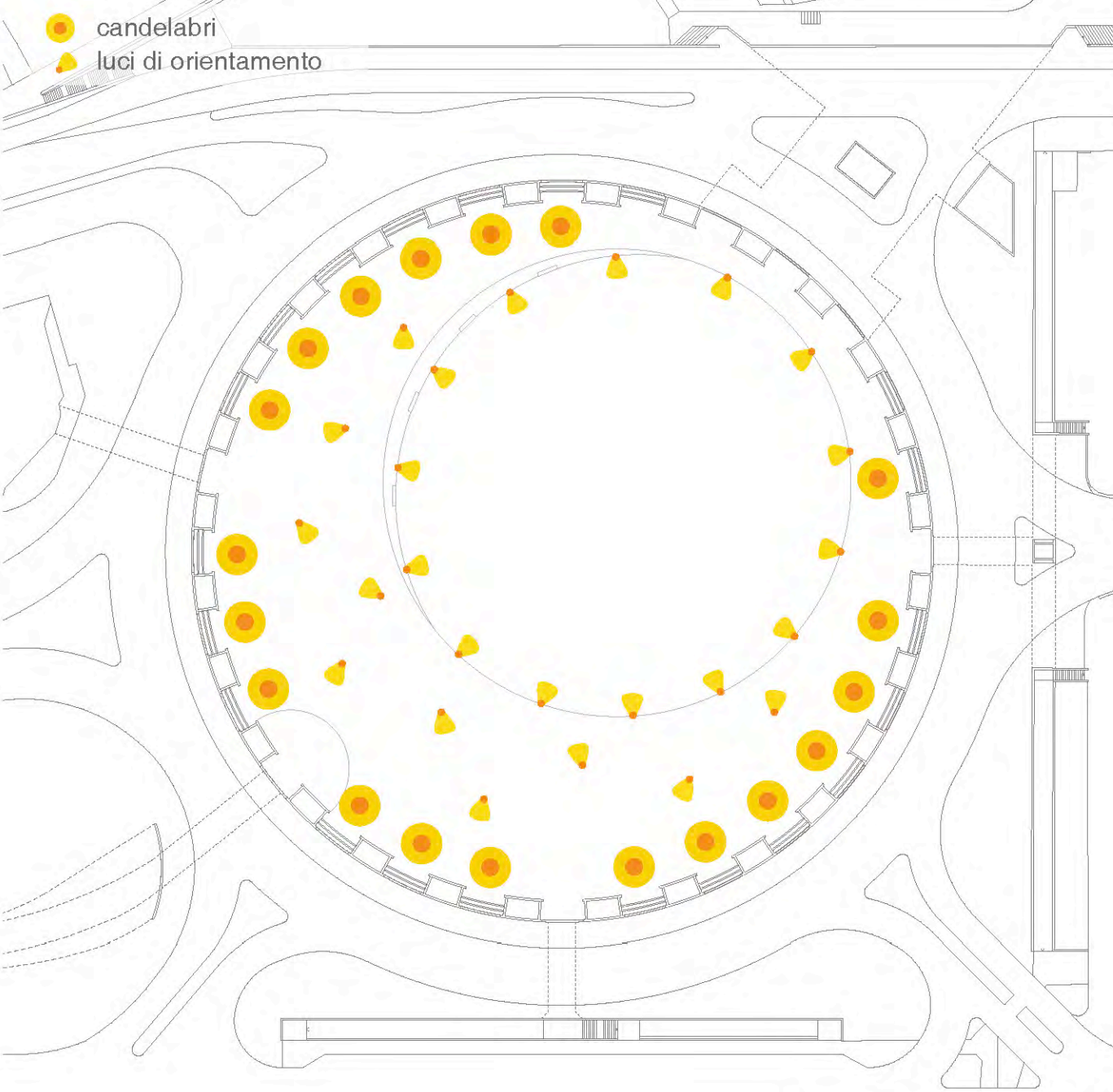
schema illuminotecnico
