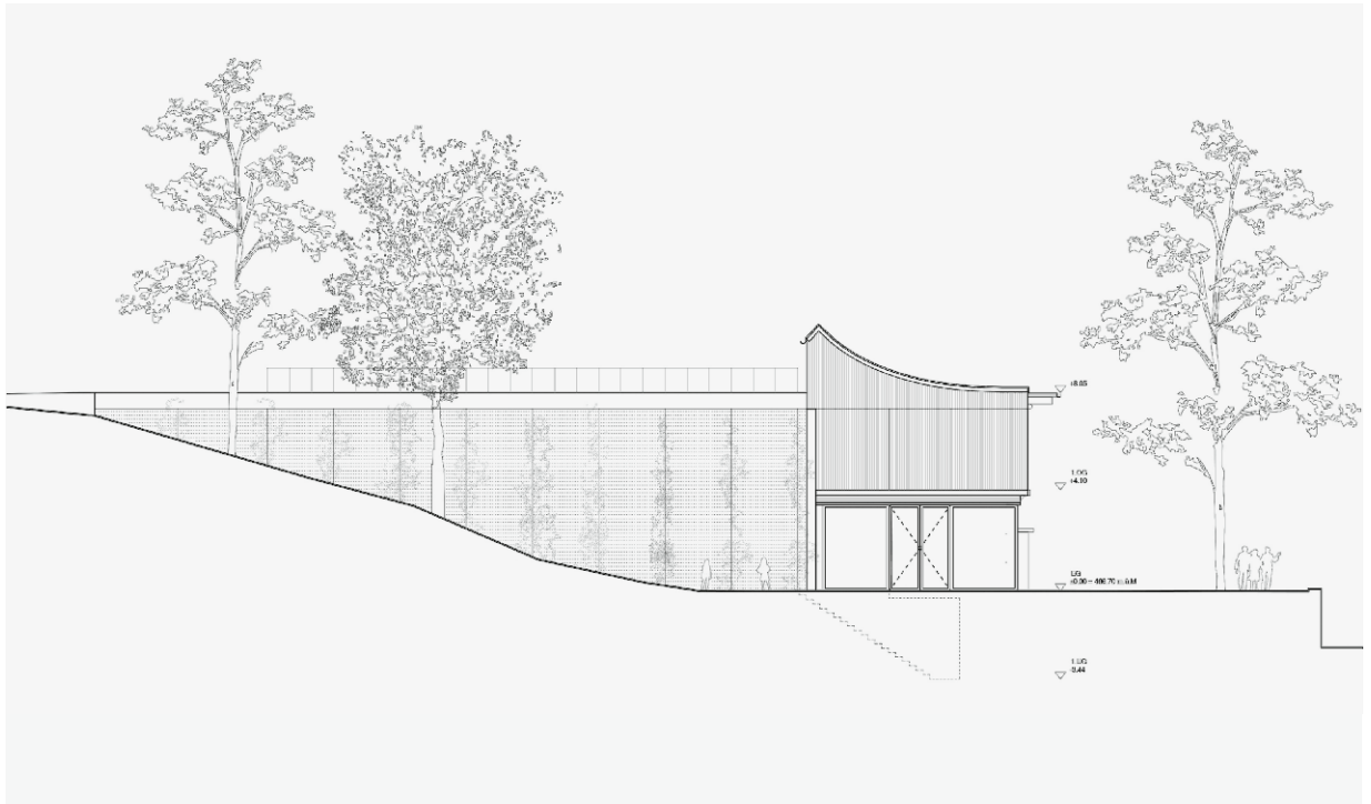
Ansicht Ost
