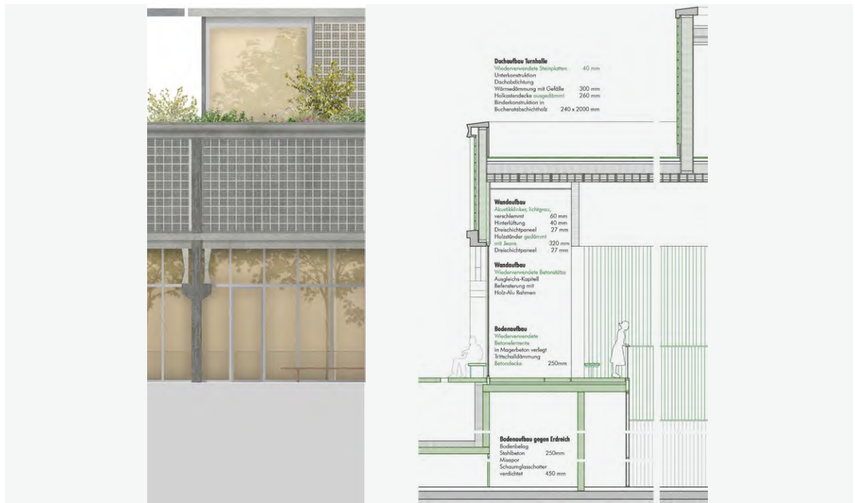
Fassadenschnitt und Fassadeansicht
