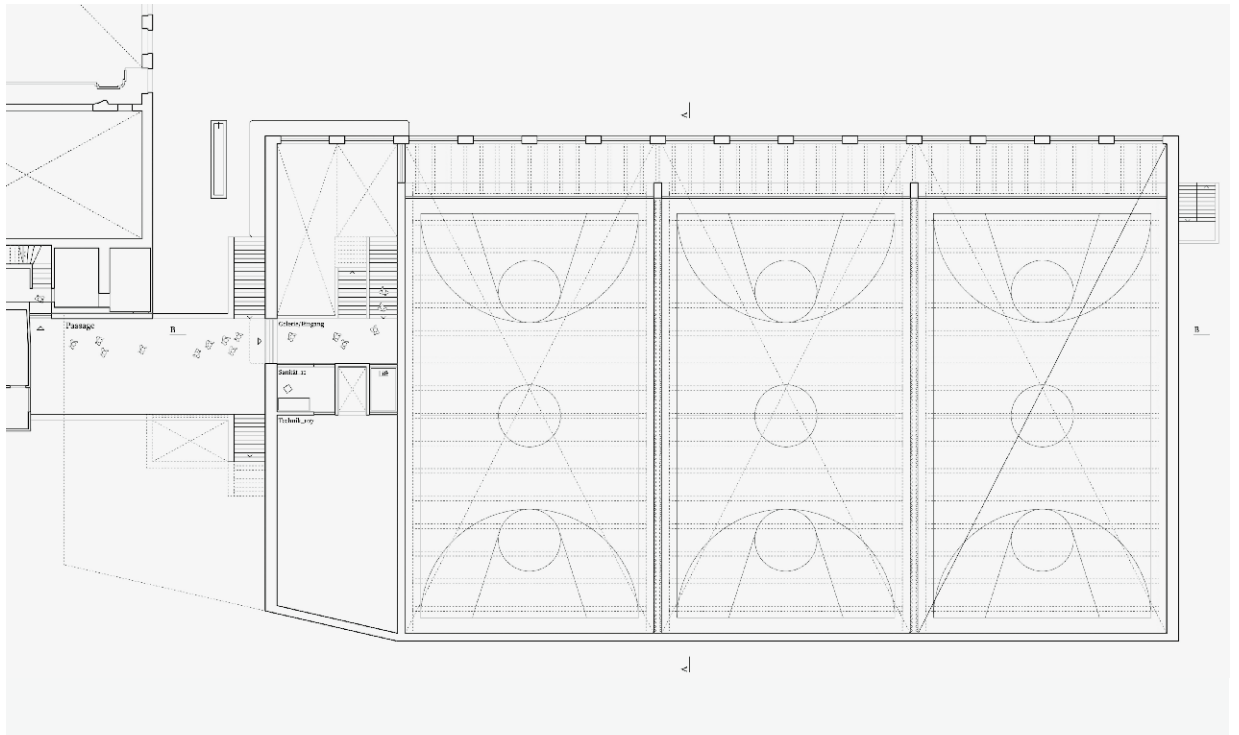
Grundriss Ebene 2
