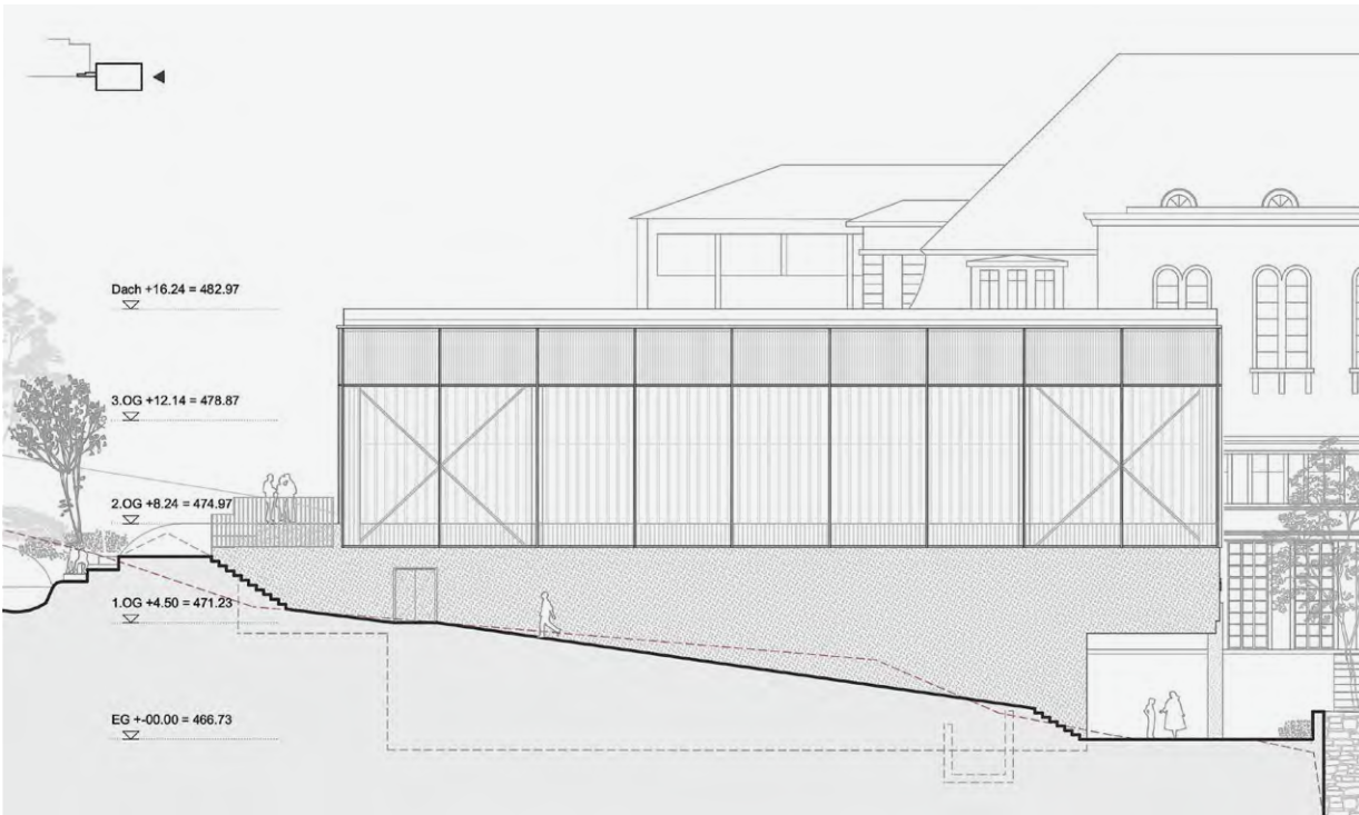
Ansicht Nord-Ost
