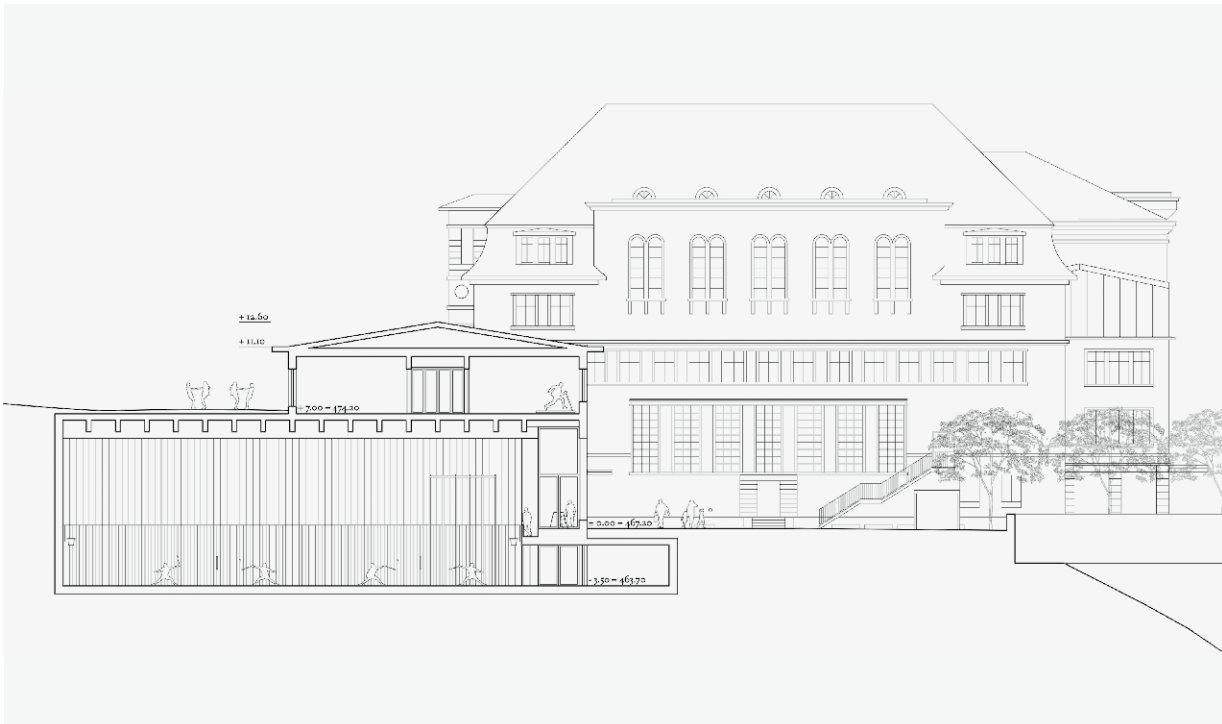
Querschnitt
