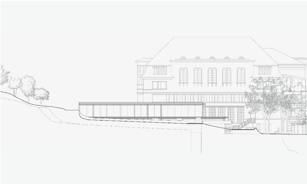
Ansicht Ost
