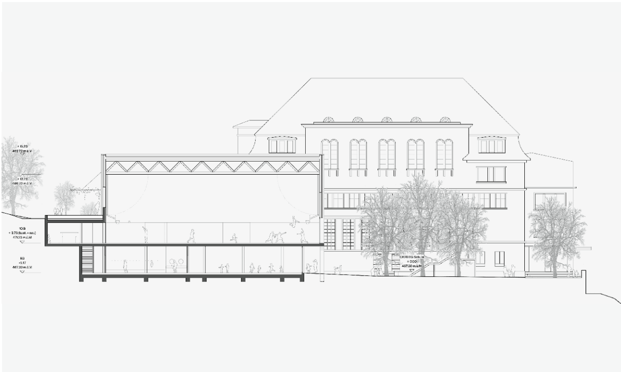
Querschnitt
