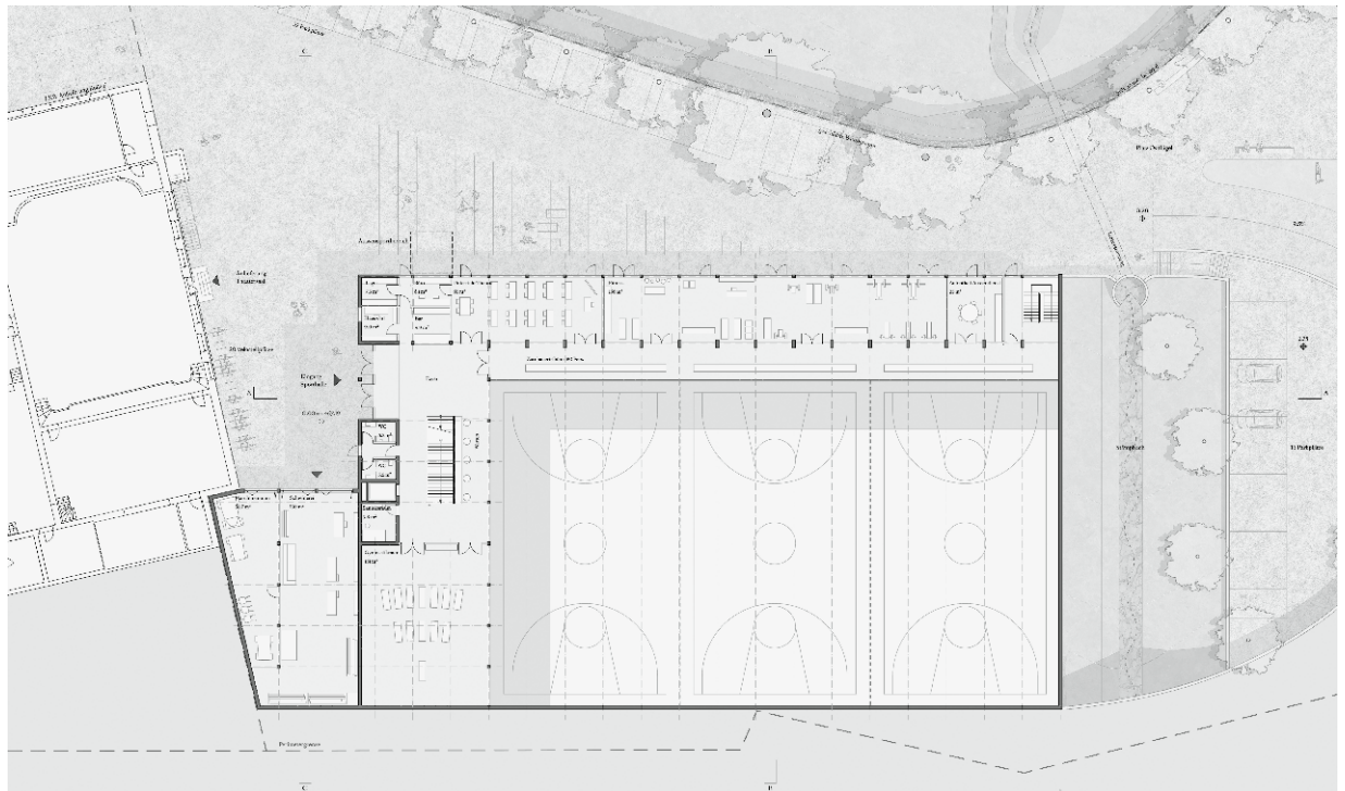
Grundriss Erdgeschoss
