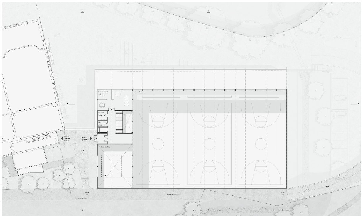
Grundriss Obergeschoss
