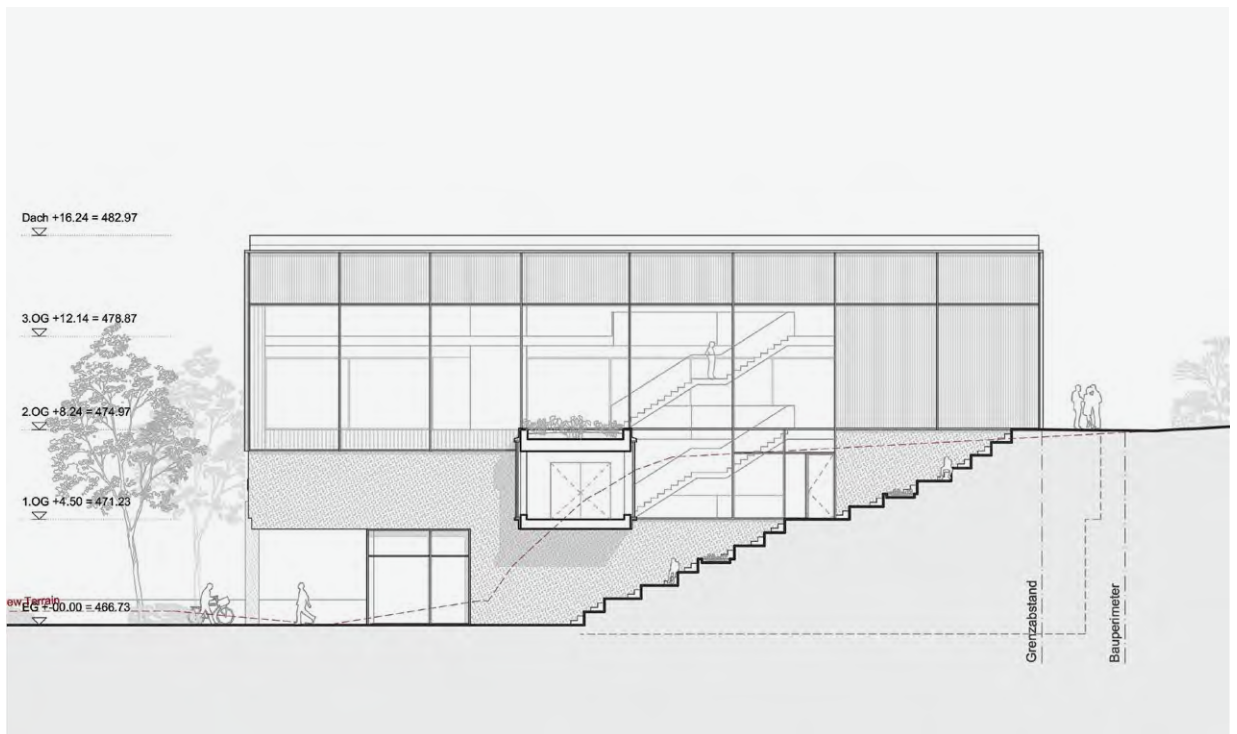
Ansicht Süd-West
