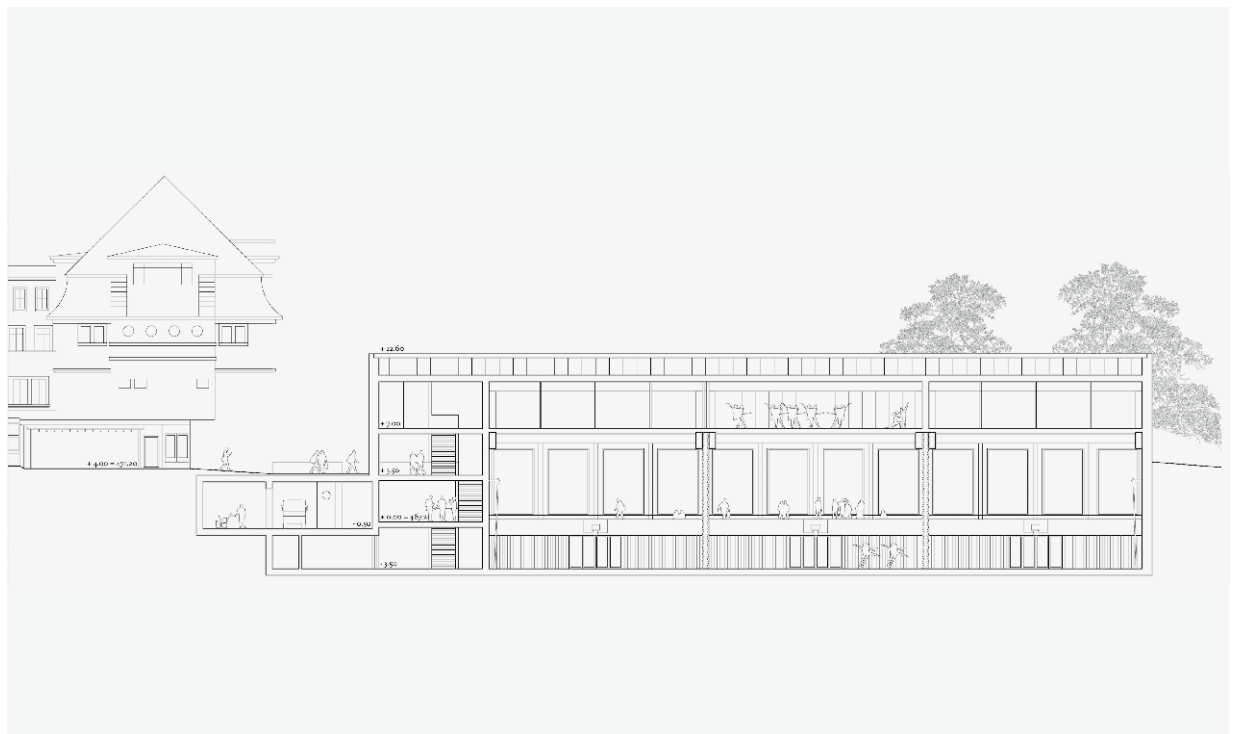
Längsschnitt B-B
