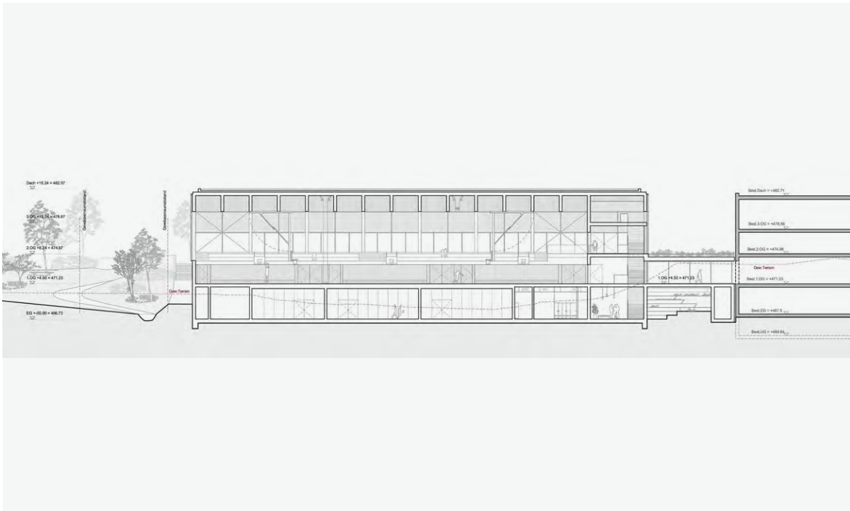
Längsschnitt
