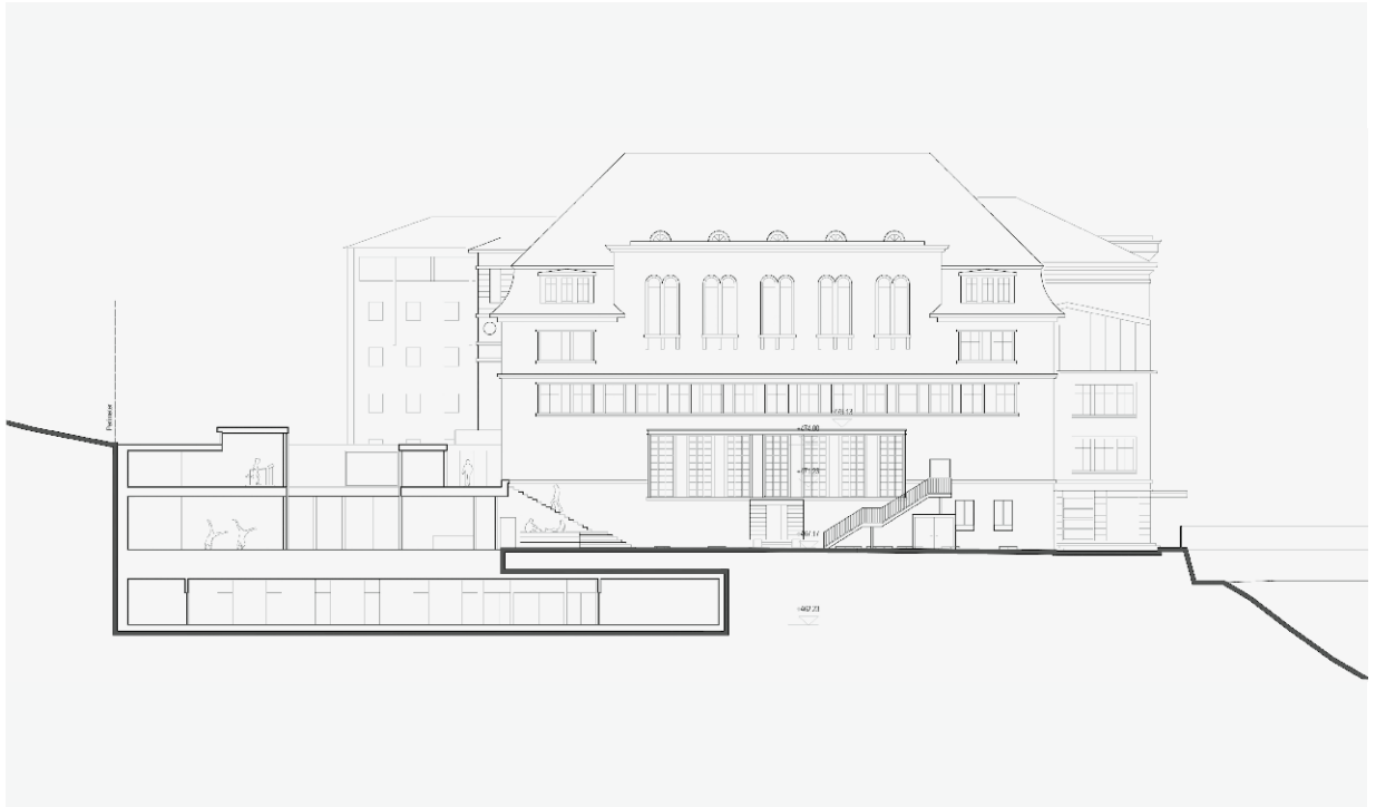
Querschnitt
