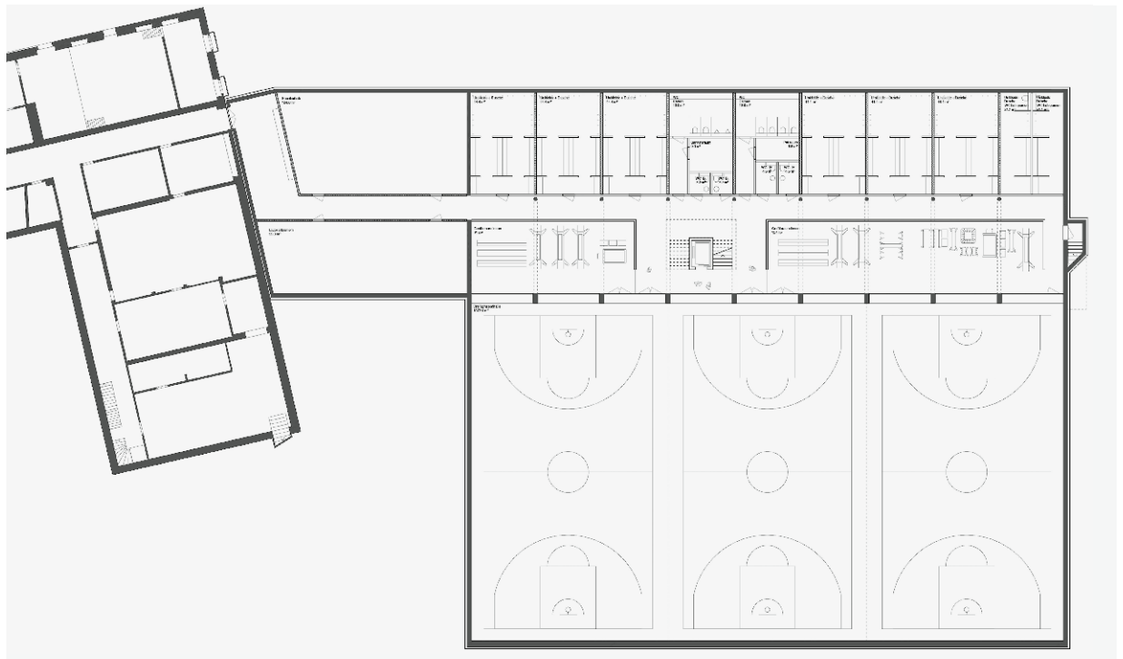
Grundriss Untergeschoss
