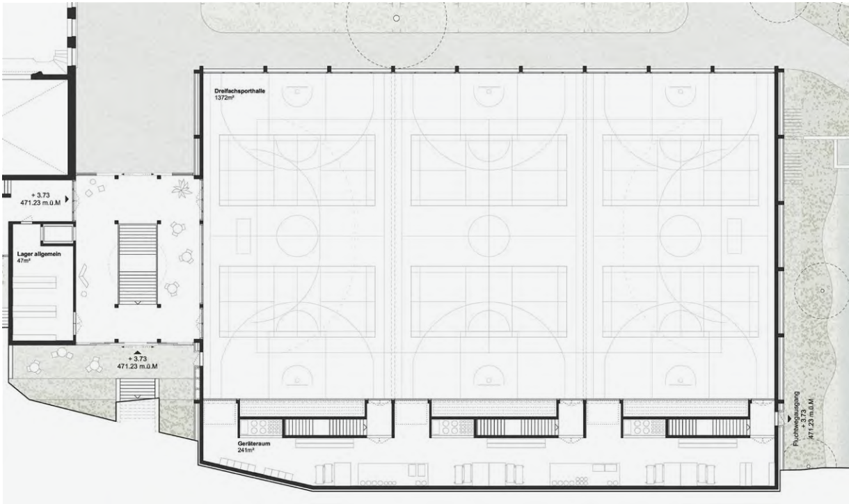
Grundriss 1. Obergeschoss
