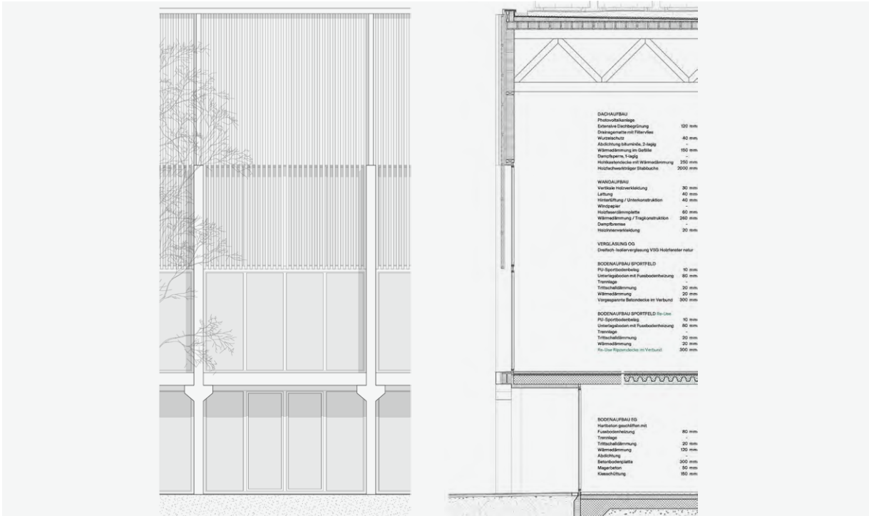
Fassadenansicht und Detailschnitt
