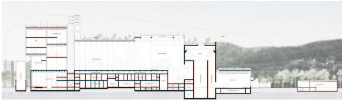
Längsschnitt
