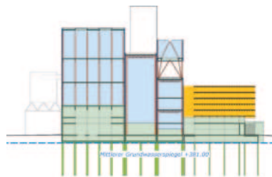
Querschnitt Vollausbau - Tragwerk KVA
