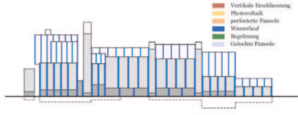
Wasserkaskade Ein Gebäude als Wasserfall. Die Dächer sind leicht geneigt und sammeln das Wasser und leiten dieses über die Kaskaden geordnet über die vertikale Fugen in der Fassade nach unten.
