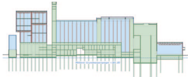
Längsschnitt Vollausbau - Tragwerk KVA
