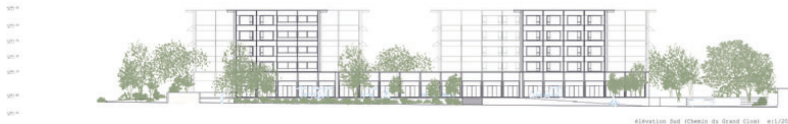
élévation Sud (Chemin du Grand Clos) en 1/200
