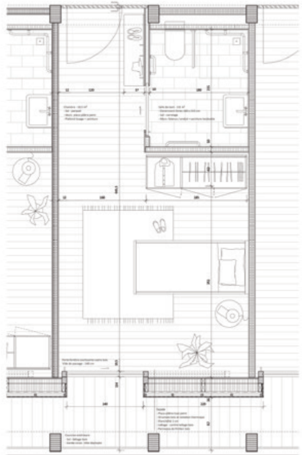
Plan de chambre 3.30
