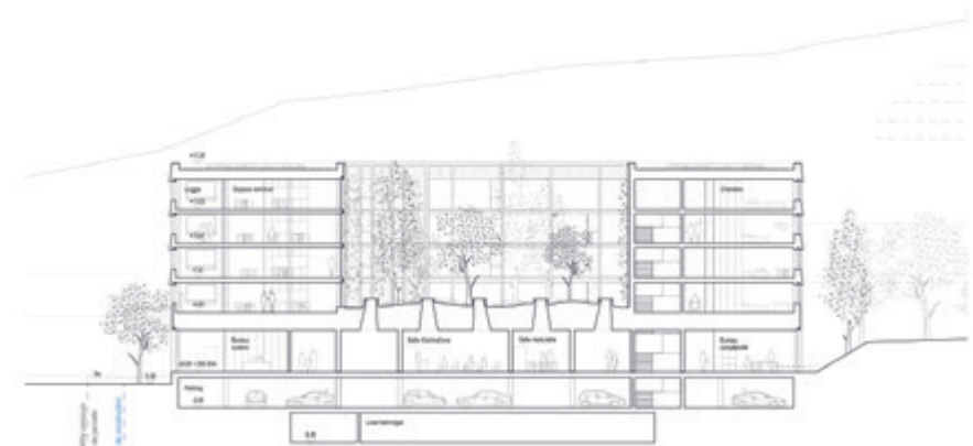
FAÇADE EST 1:200
