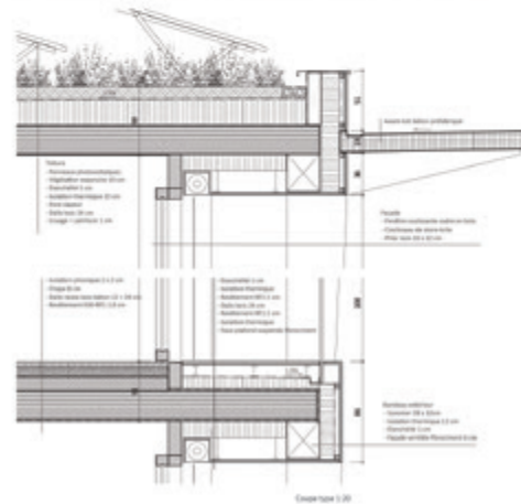
Coupe type 3.30
