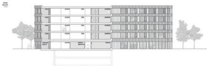
FACADE OUEST 1:200
