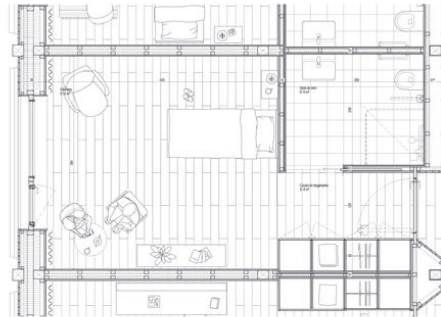
PLAN CHAMBRE TYPE 1:20
