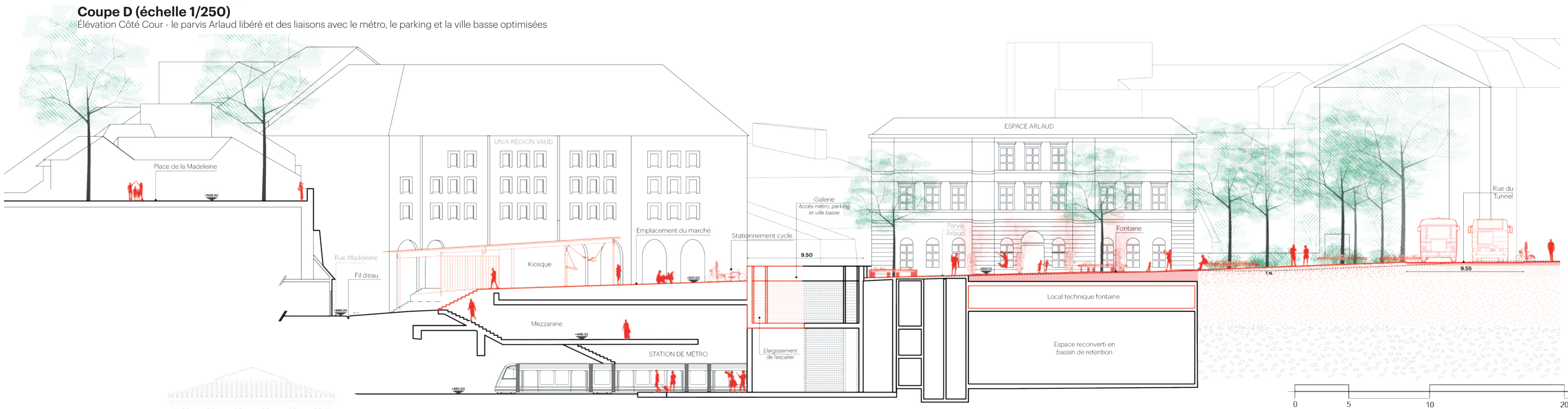
Coupe D (échelle 1/250) Élévation Côte Cour - le parvis Airlaud libéré et des liaisons avec le métro, le parking et la ville basse optimisées
