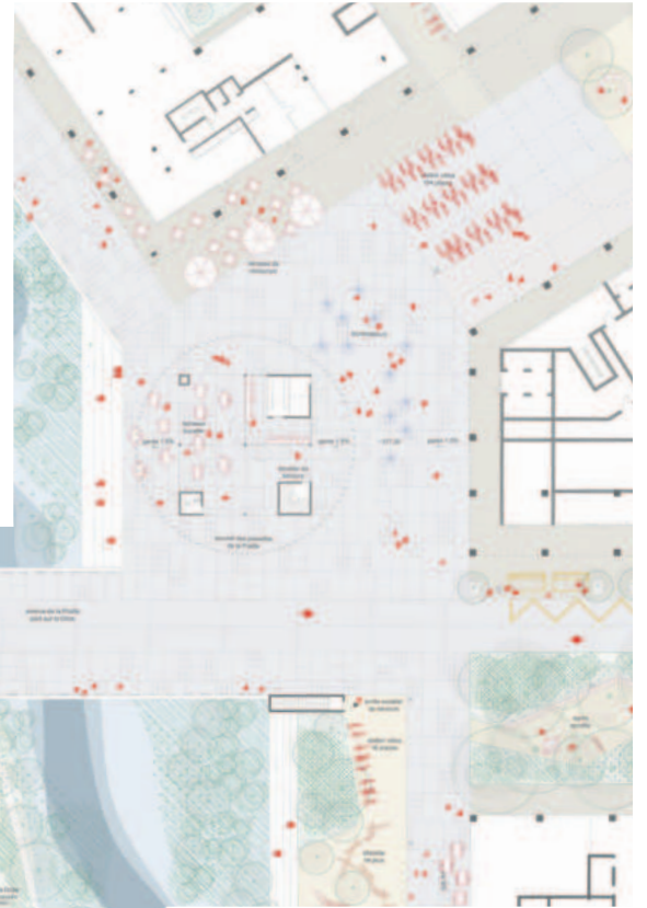
PLACETTES DE LA PRAILLE _ PLAN 1:250
