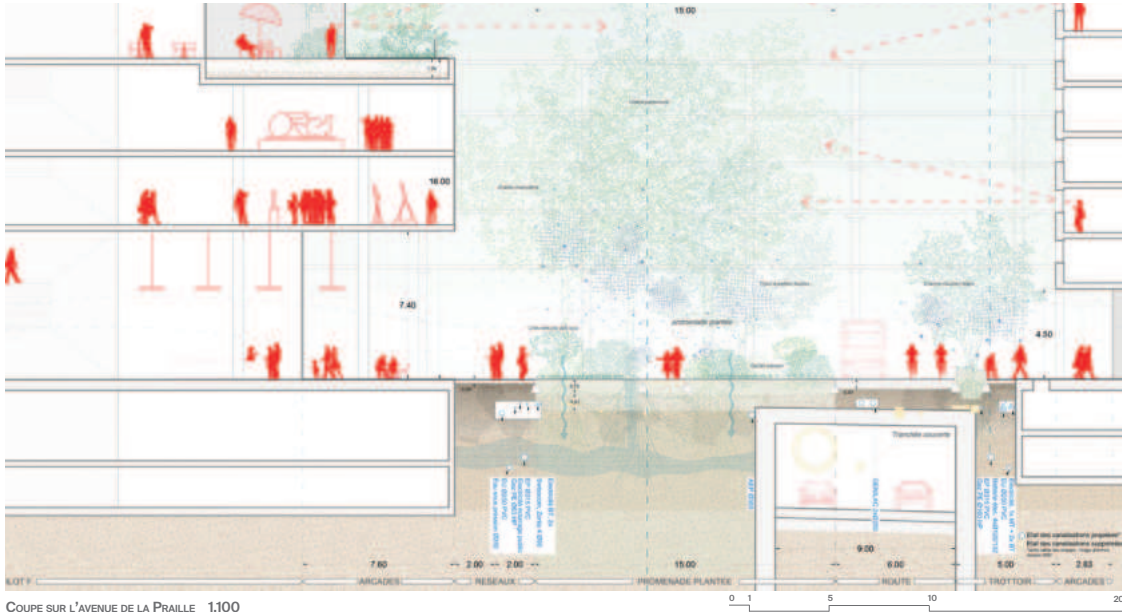
COUPE SUR L'AVENUE DE LA PRAILLE _ 1:100
