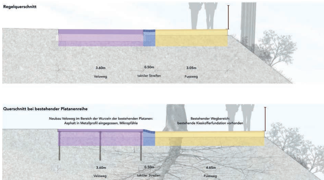
Schemaschnitte zum Umgang mit dem Baumbestand
