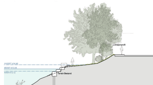
Schnitt Liegewiese 1:500
