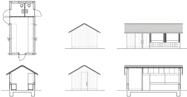
Pläne Buvette 1:250
