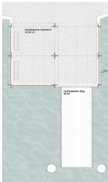
Grundriss Schiffflände 1:250
