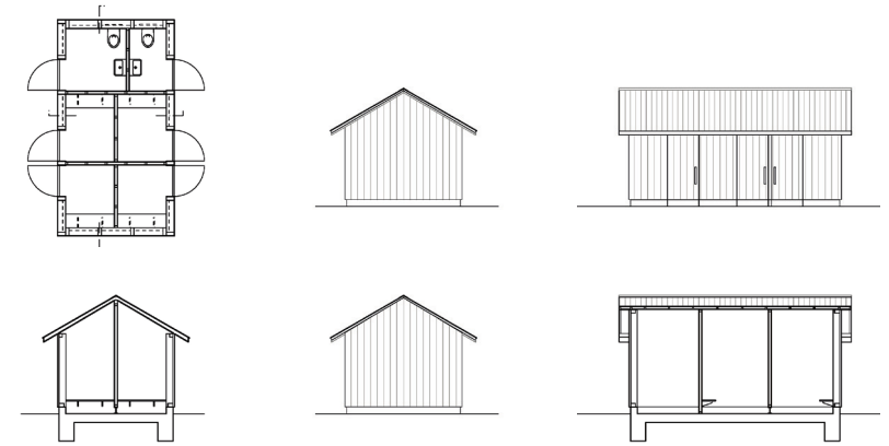
Pläne Umkleide 1:250
