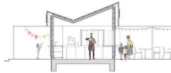
Schnitt, Buvette 1:250
