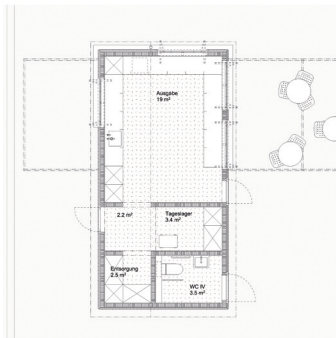
Grundriss Buvette 1:250
