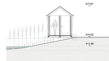
Schnitt Umkleide 1:250
