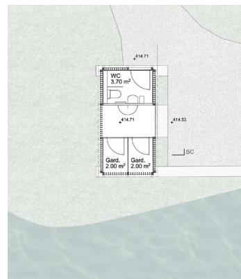
Grundriss Umkleide 1:250
