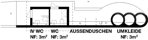
Grundriss Umkleide 1:250
