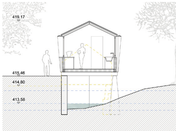
Schnitt Buvette 1:250
