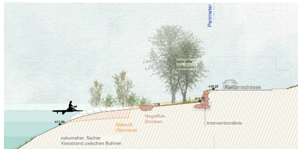
Schnitt J-J', Chäppeli 1:500
