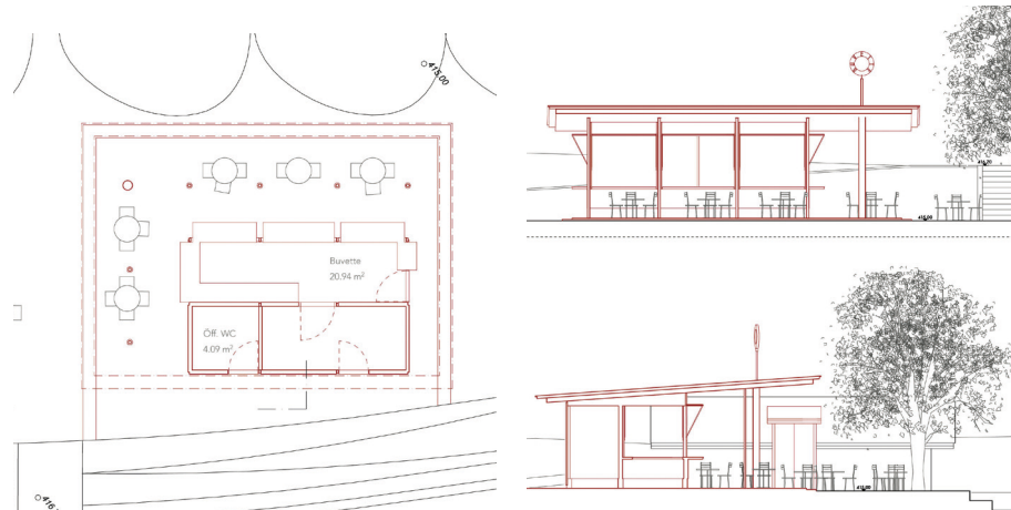
Grundriss Buvette 1:250
