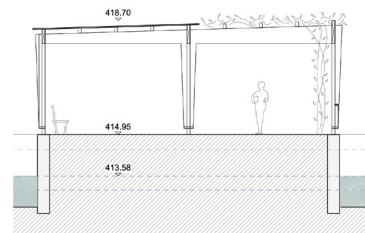
Schnitt Schiffflände 1:250
