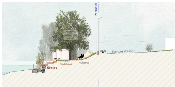
Schnitt B-B', Brüzigen 1:500
