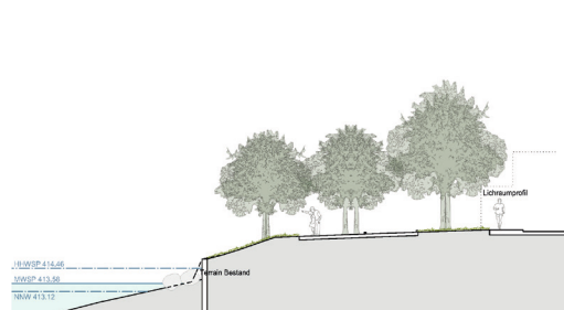
Schnitt Grillplatz 1:500
