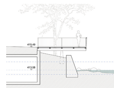
Schnitt Bellevue 1:250
