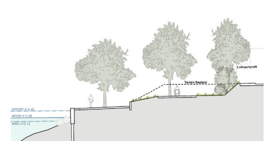
Schnitt Promenade 1:500
