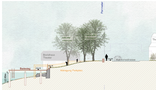
Schnitt C-C', Naber 1:500
