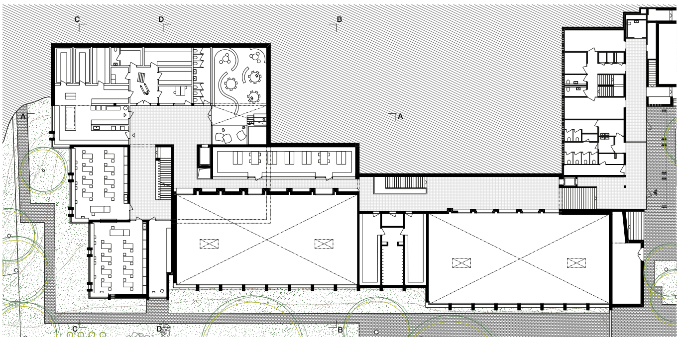
Grundriss 1. Untergeschoss 1:500
