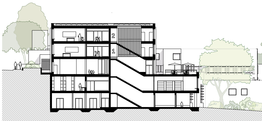
Schnitt D-D 1:500
