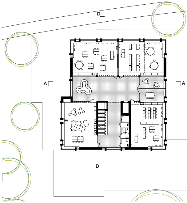
Grundriss 1./2. Obergeschoss 1:500
