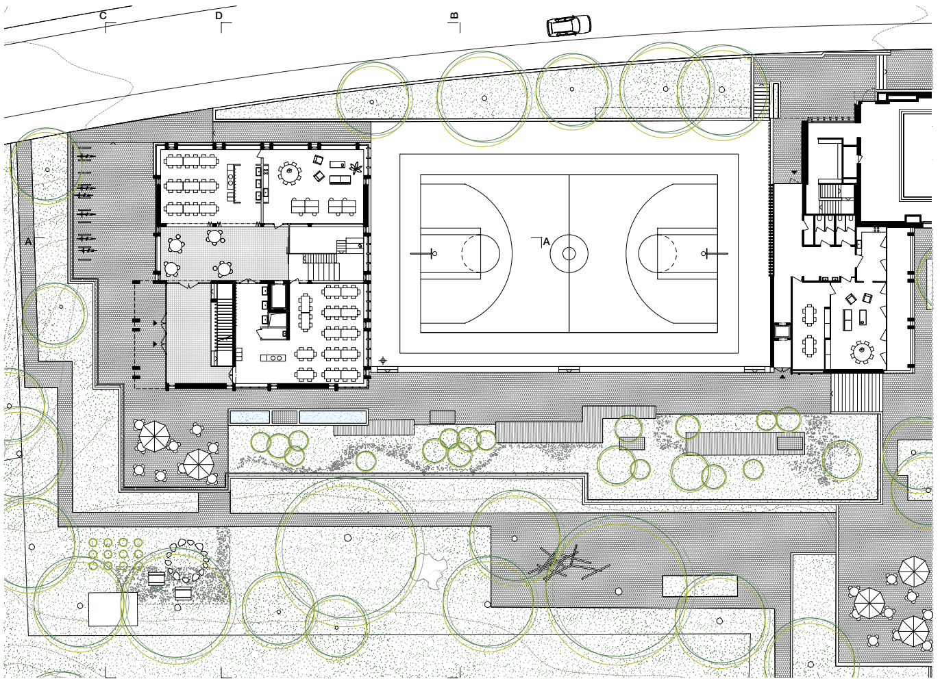
Gundriss Erdgeschoss 1:500
