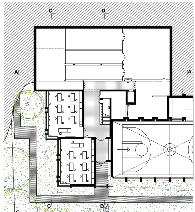
Grundriss 2. Untergeschoss 1:500
