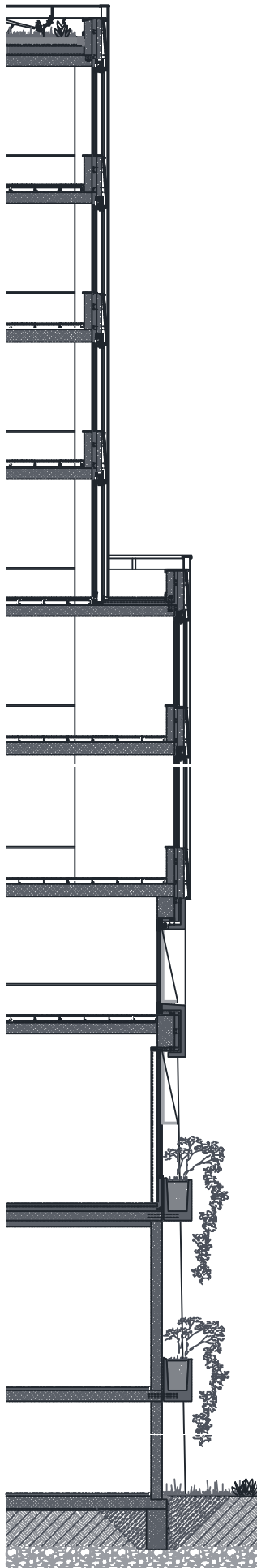
Fassadenschnitt
