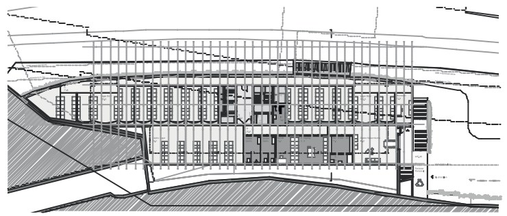
Grundriss 1. Obergeschoss
