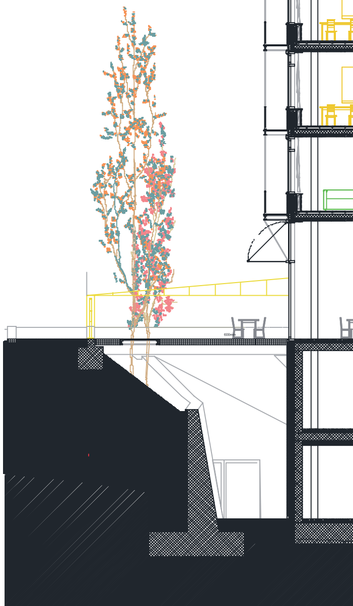
Fassadenschnitt
