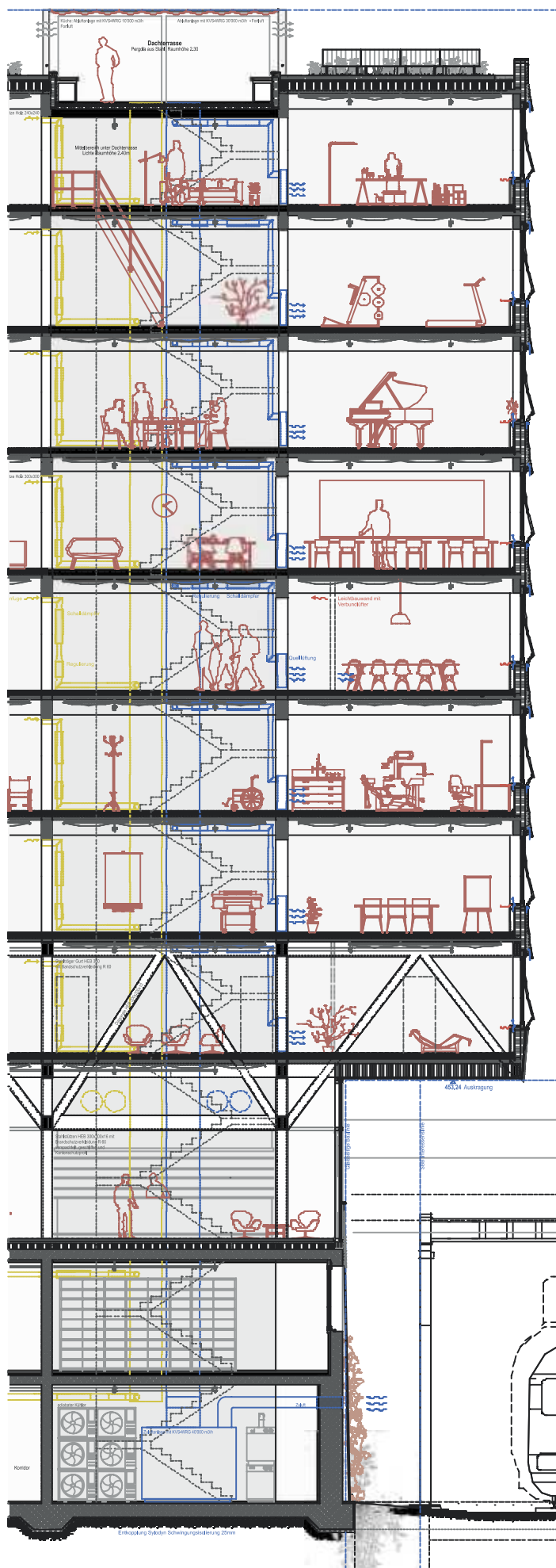
Fassadenschnitt
