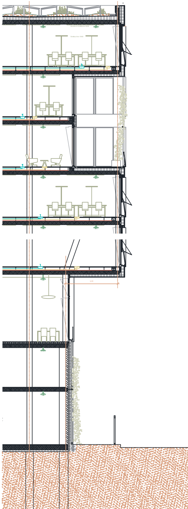
Fassadenschnitt
