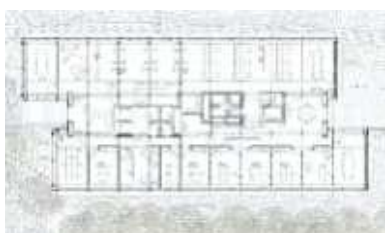
Regelgeschoss - Szenario Büro
