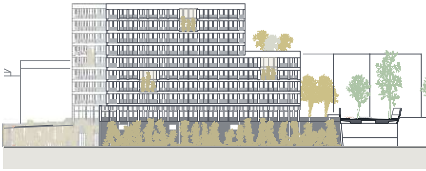
70 Ansicht Nordwest
