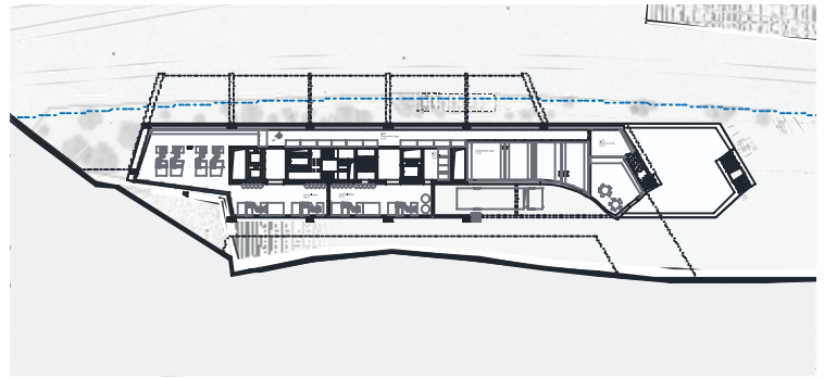
Grundriss 1. Obergeschoss
