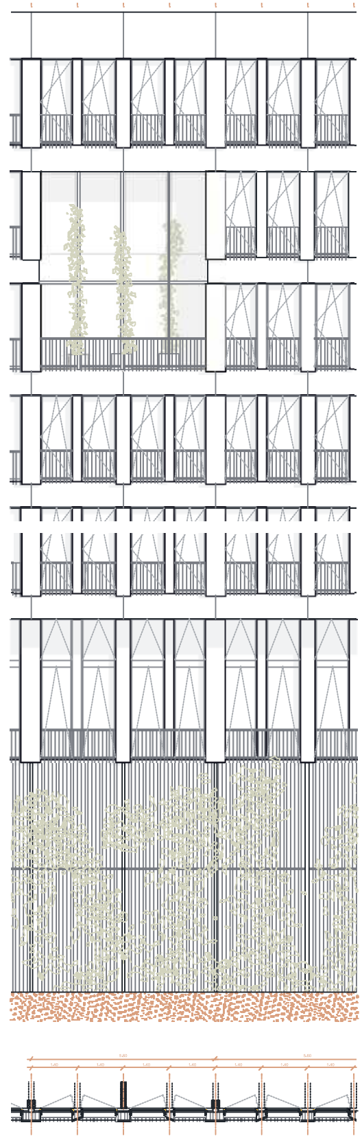
Fassadenansicht
