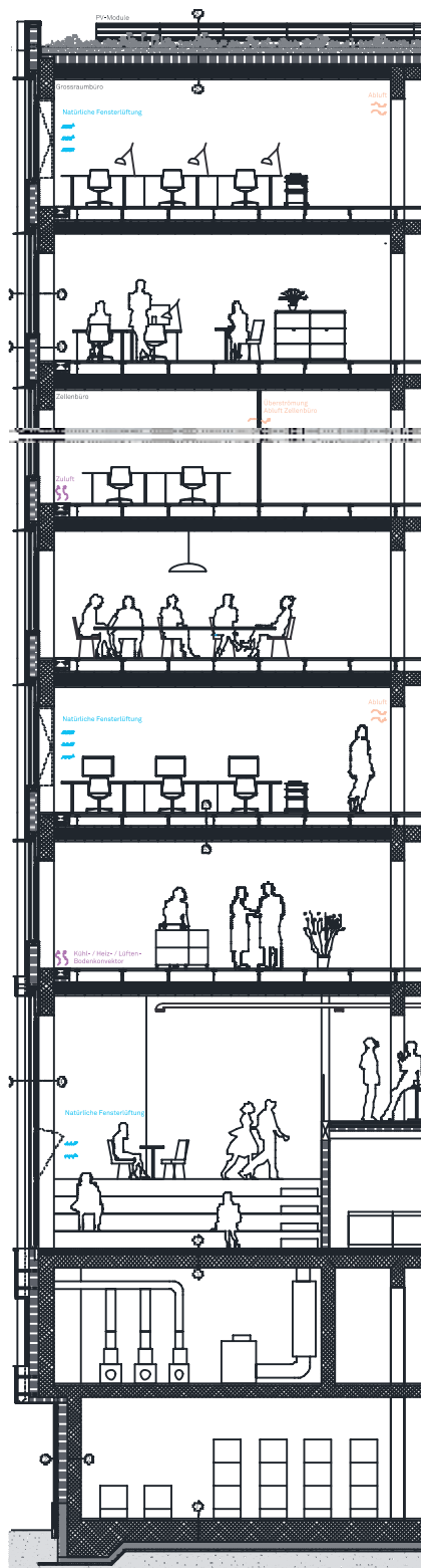
Fassadenschnitt
