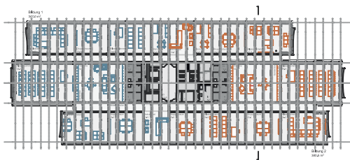
Regelgeschoss - Szenario Bildung
