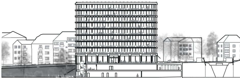
Längsschnitt
