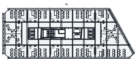
Regelgeschoss - Szenario Bildung
