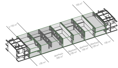
Produktionsgeschosse
