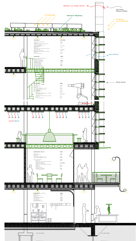
Konstruktionsschnitt
