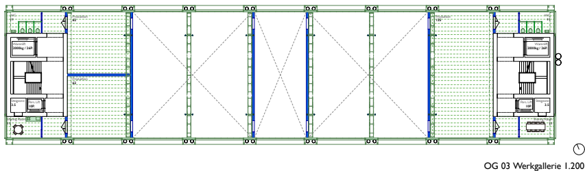
OG 03 Werkgalerie 1.200
