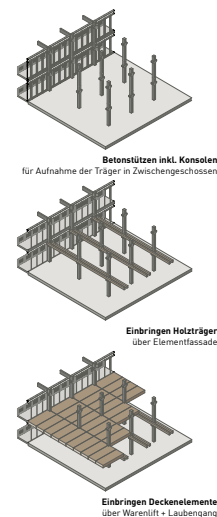
Konstruktionsprinzipien und Vergleich Deckensysteme
