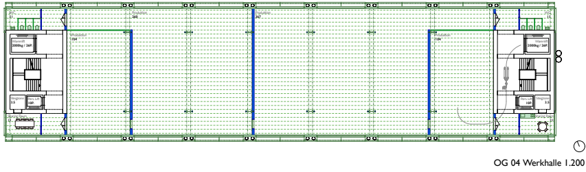
OG 04 Werkhalle 1.200
