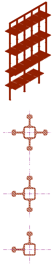
Aufbau Tragstruktur aus SBB-Schienenprofilen
