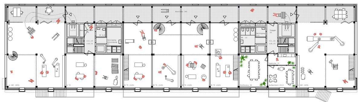
Grundriss 3./5. Obergeschoss
