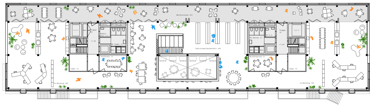
Grundriss 2. Obergeschoss
