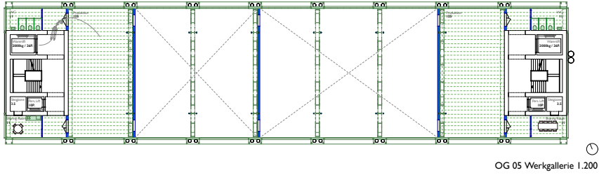
OG 05 Werkgalerie 1.200
