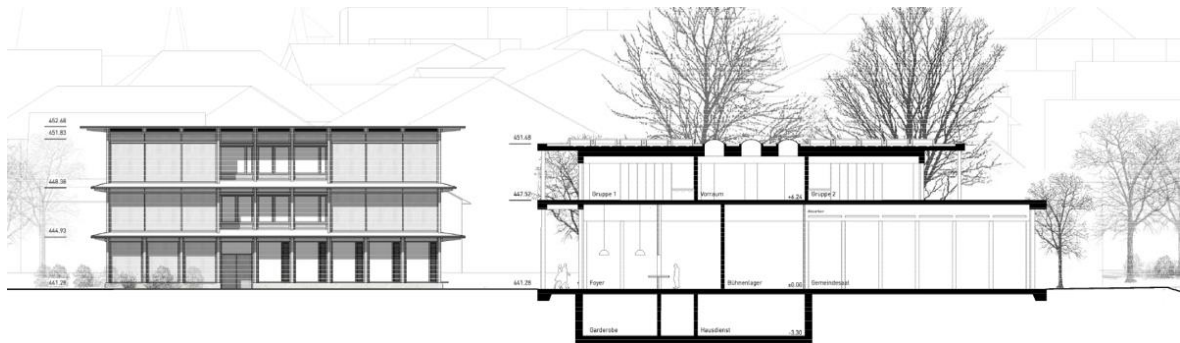
Abb. 40 Schnitt Gemeindesaal West
