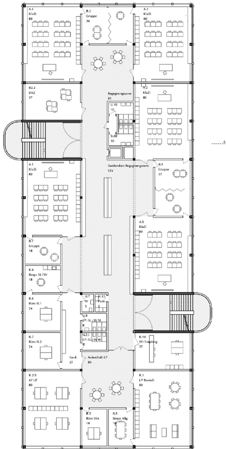
Abb. 6 Grundriss 1. Obergeschoss
