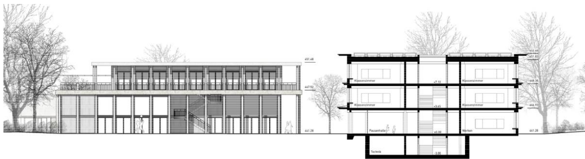
Abb. 39 Schnitt Schulhaus Ost
