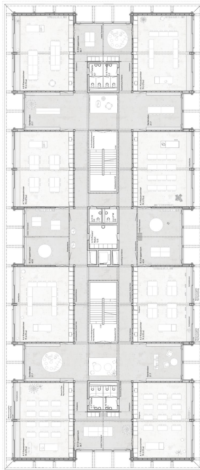
Abb. 35 Grundriss 1. Obergeschoss
