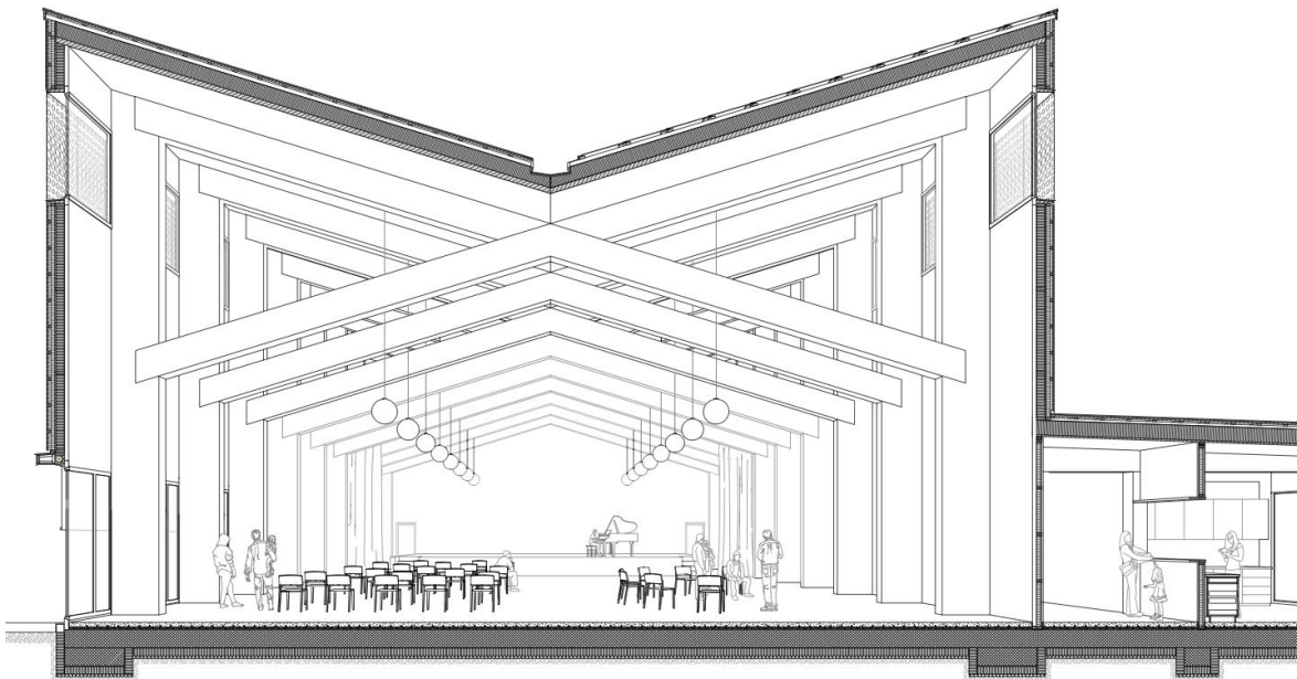
Abb. 22 Schnittperspektive Gemeindesaal
