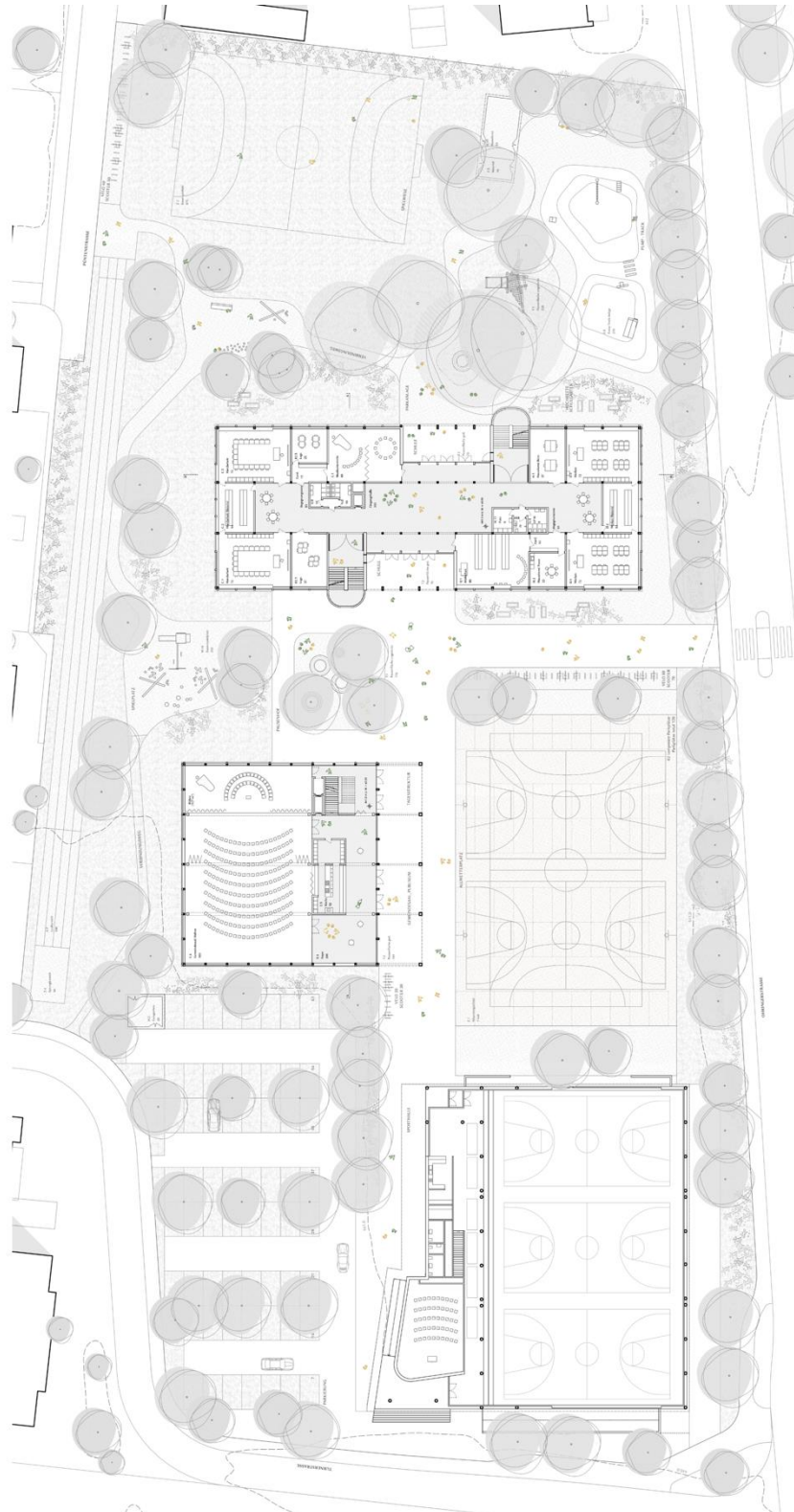
Abb. 5 Situation Erdgeschoss
