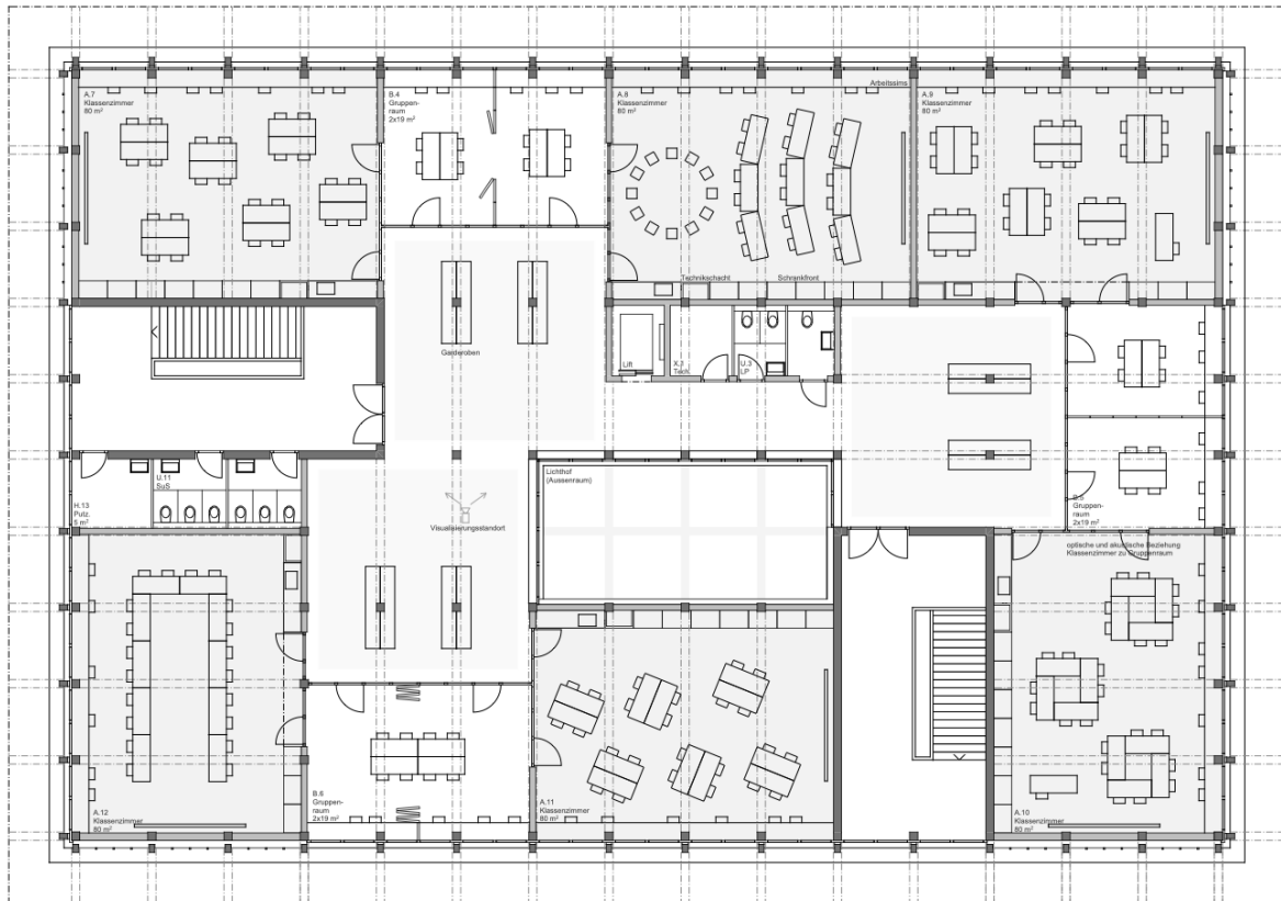
Abb. 46 Grundriss Schulhaus
