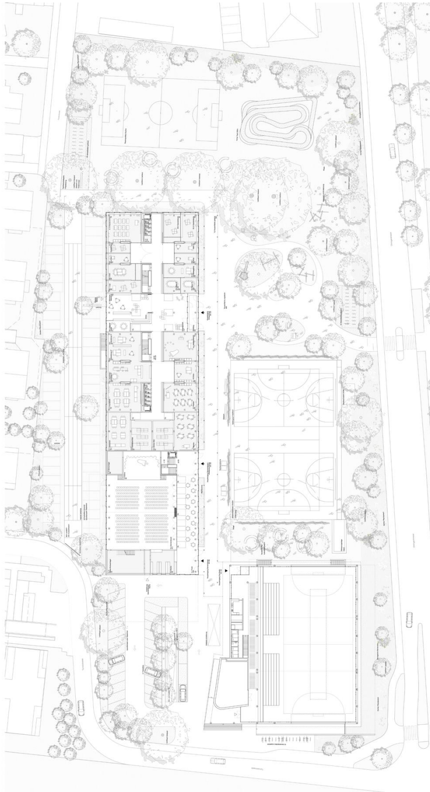
Abb. 52 Situation Erdgeschoss
