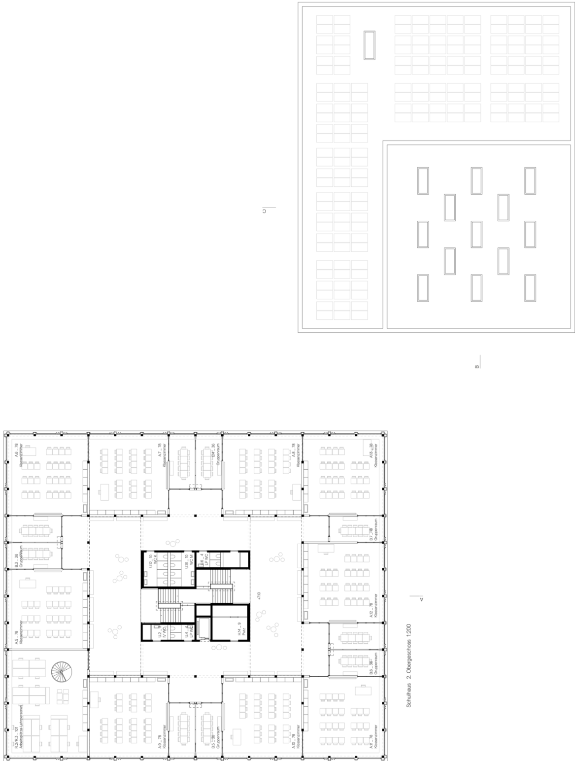
Abb. 27 Grundriss 2. Obergeschoss
