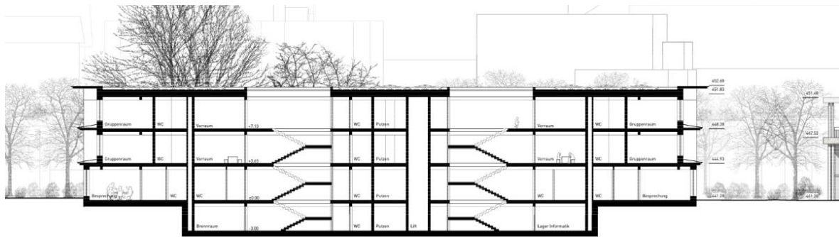
Abb. 38 Schnitt Schulhaus Süd
