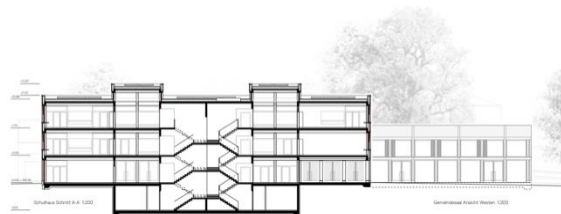
Abb. 31 Schnitt Schulhaus
