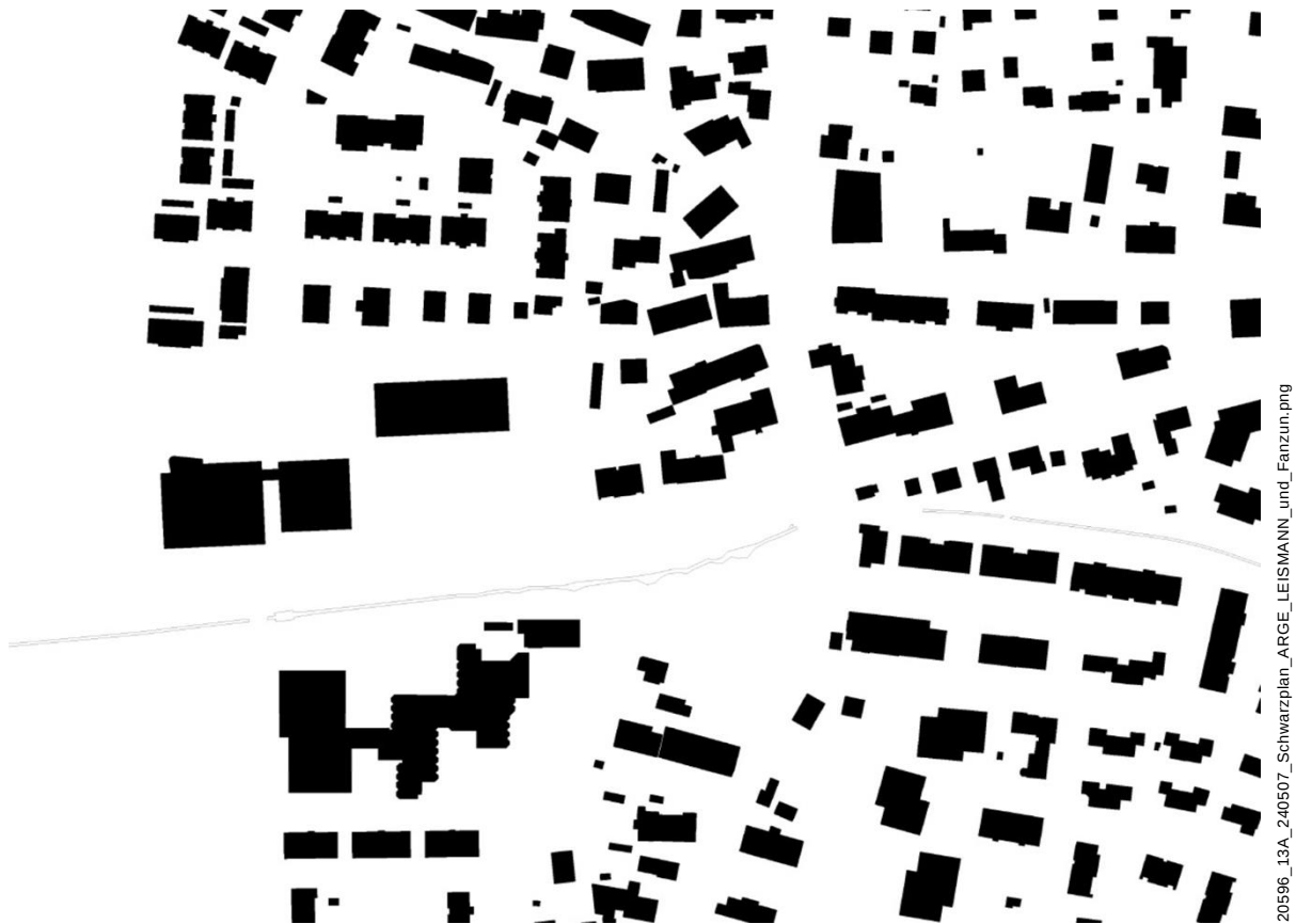
Abb. 32 Schwarzplan
