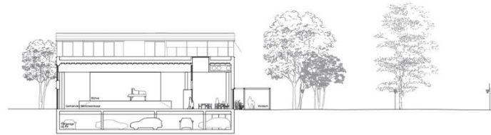
Abb. 57 Querschnitt
