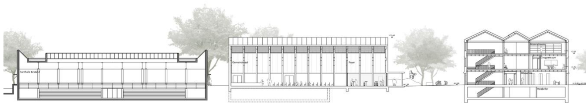
Abb. 18 Schnitt Ost-West
