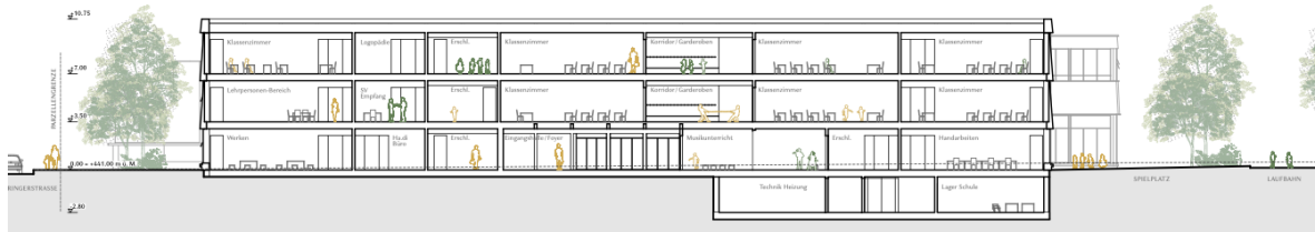
Abb. 11 Schnitt Nord - Süd
