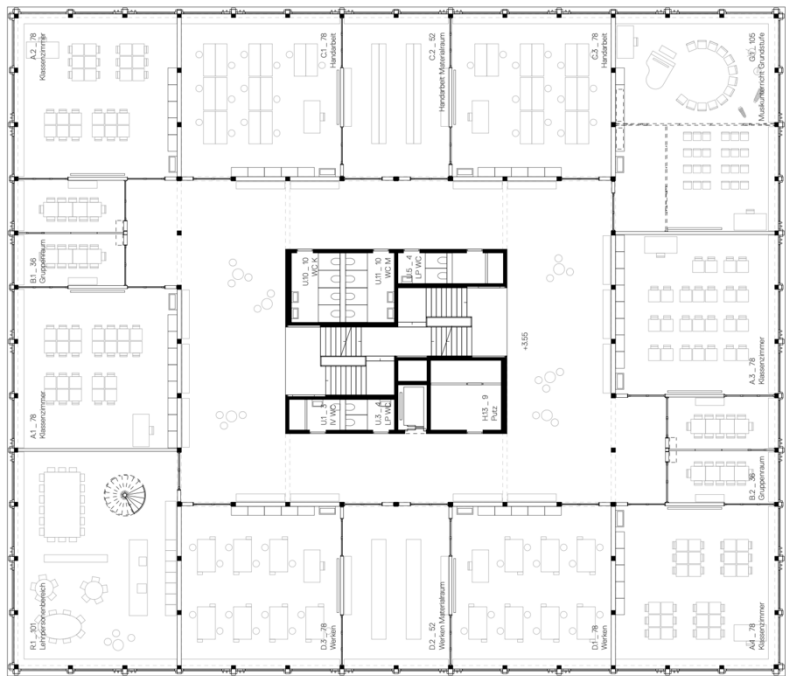
Abb. 26 Grundriss 1. Obergeschoss
