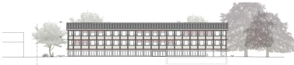
Abb. 20 Ansicht Schulhaus West
