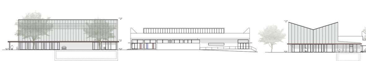
Abb. 19 Ansicht Gemeindesaal (links: Nord, Rechts: Ost)
