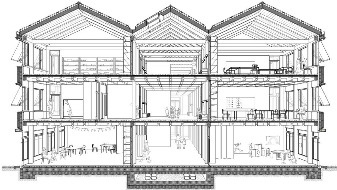
Abb. 21 Schnittperspektive Schulhaus
