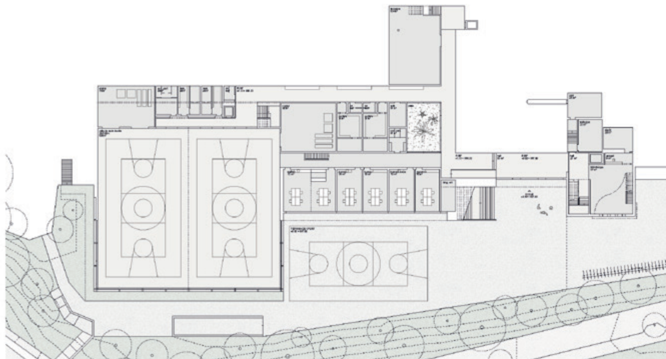
Plan de l'étage 1 : 1/200
