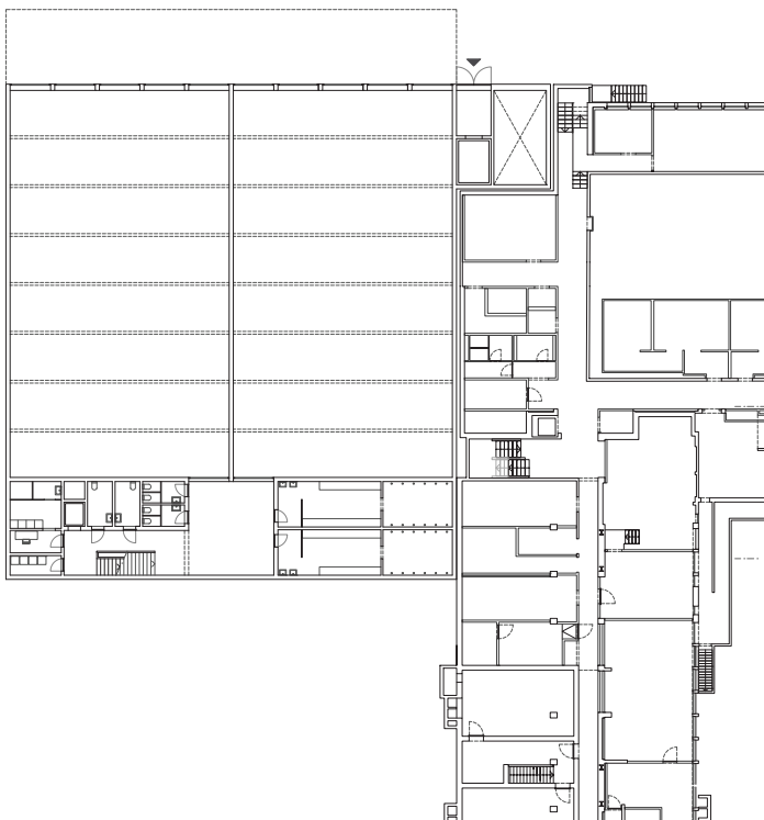
Grundriss 2. Untergeschoss 1:600
