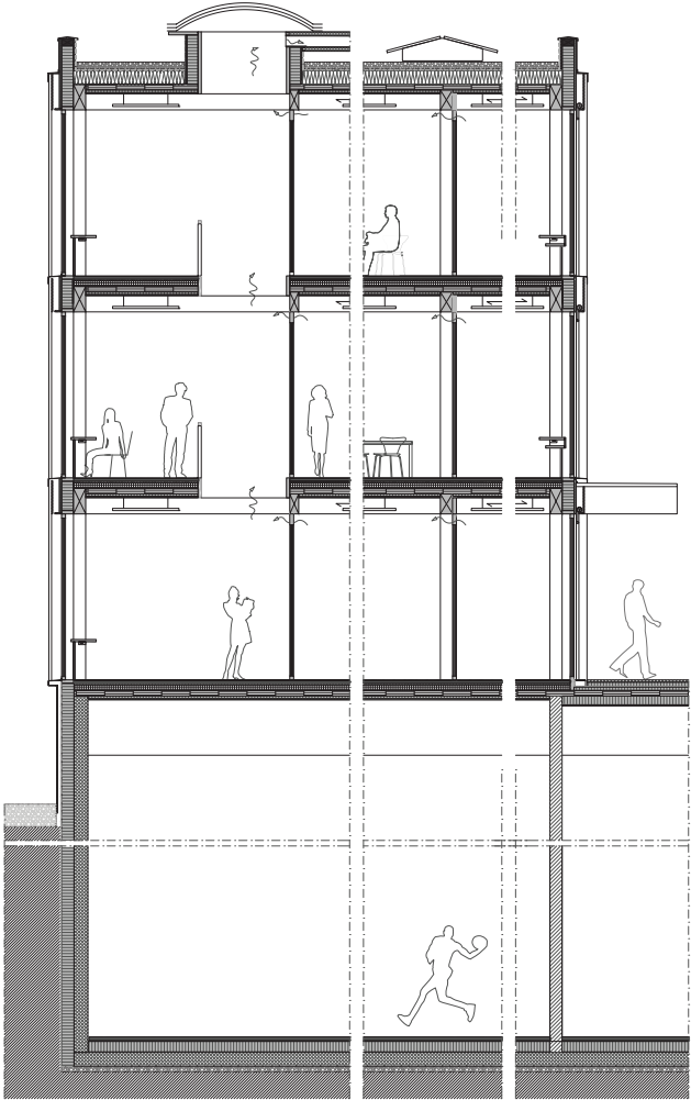
Konstruktionsschnitt und Ausschnitt Fassade 1:150
