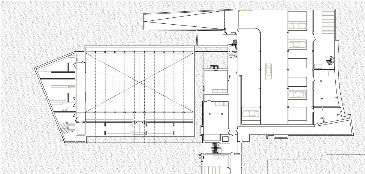
Grundriss 2. Untergeschoss 1:600
