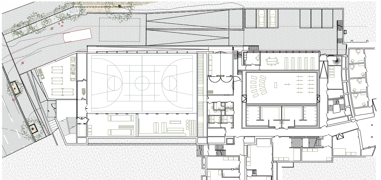
Grundriss 1. Untergeschoss 1:600
