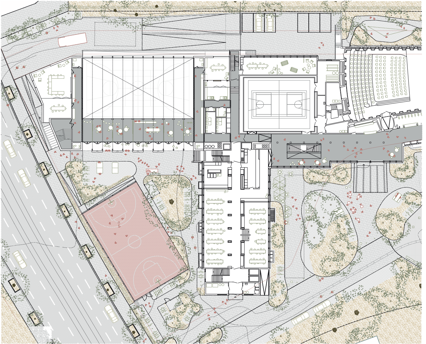
Grundriss Erdgeschoss 1:600
