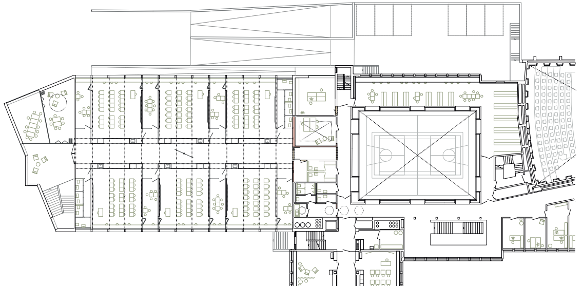
Grundriss 1. Obergeschoss 1:600
