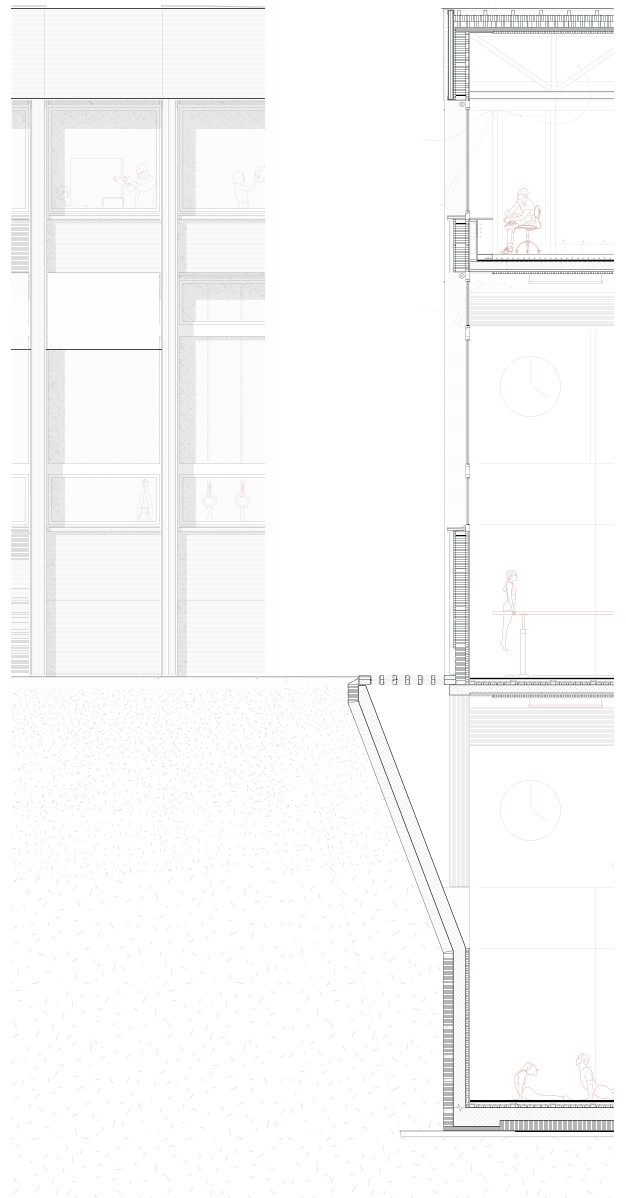
Konstruktionsschnitt und Ausschnitt Fassade 1:150
