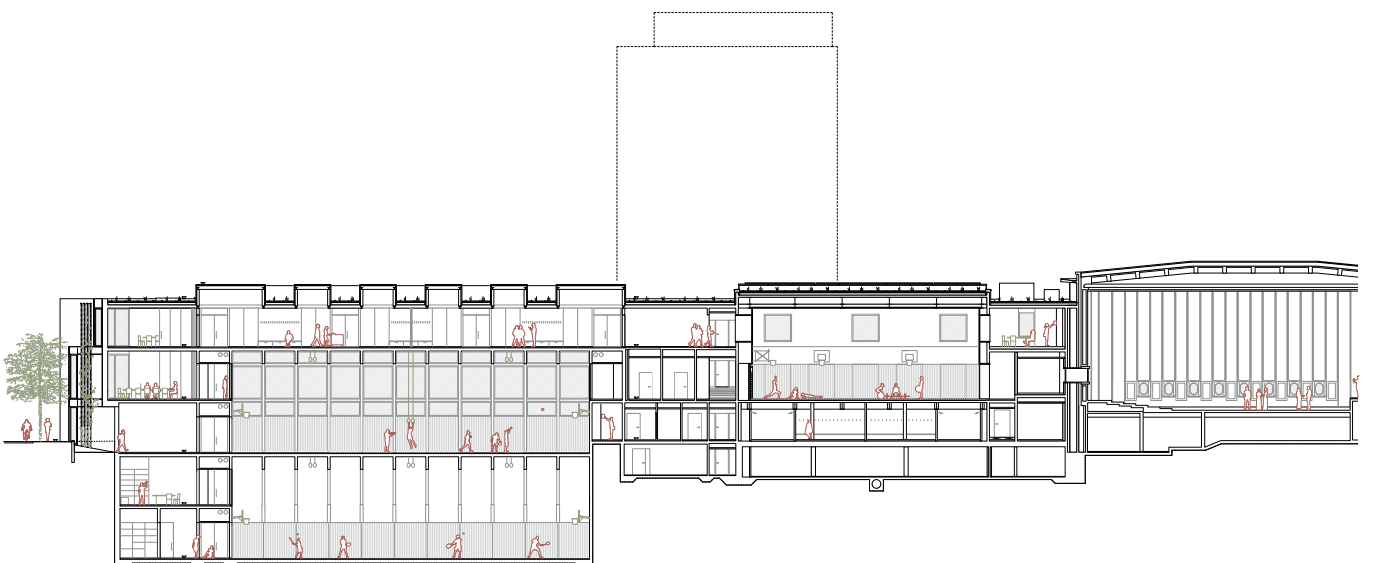
Längsschnitt 1:600
