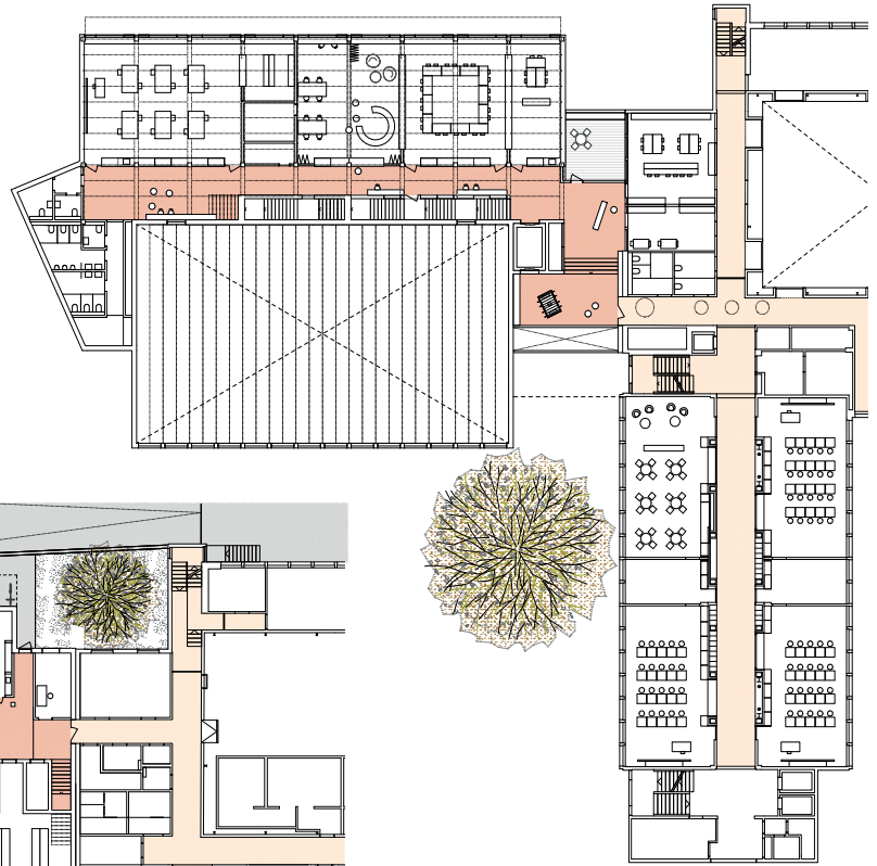
Grundriss 1. Obergeschoss 1:600
