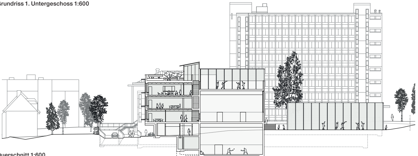
Querschnitt 1:600
