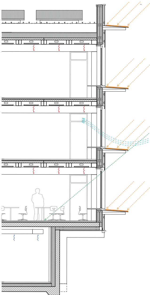
Konstruktionsschnitt und Ausschnitt Fassade 1:150
