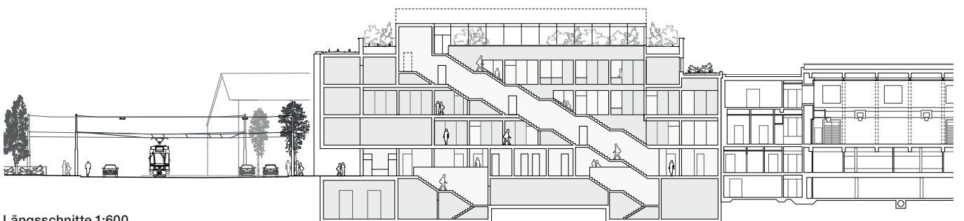
Längsschnitte 1:600
