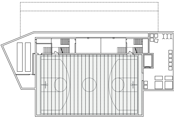
Grundriss 1. Untergeschoss 1:600
