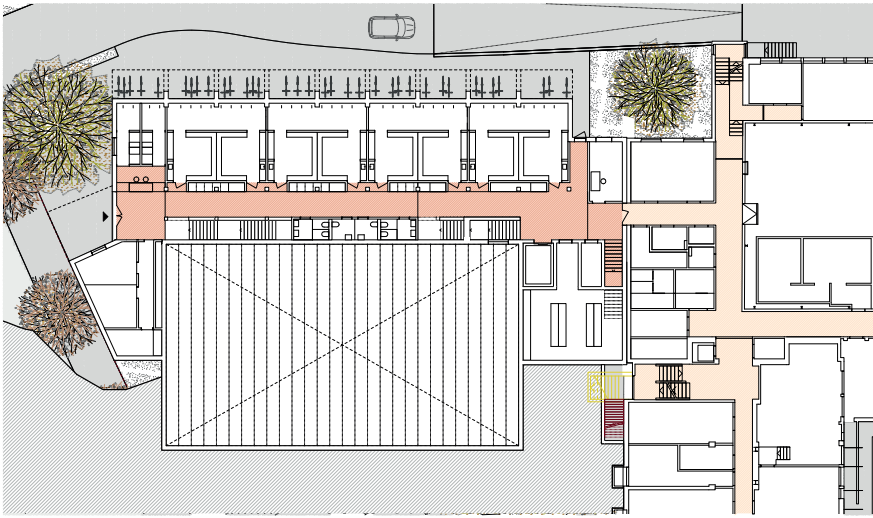
Grundriss Tiefparterre 1:600
