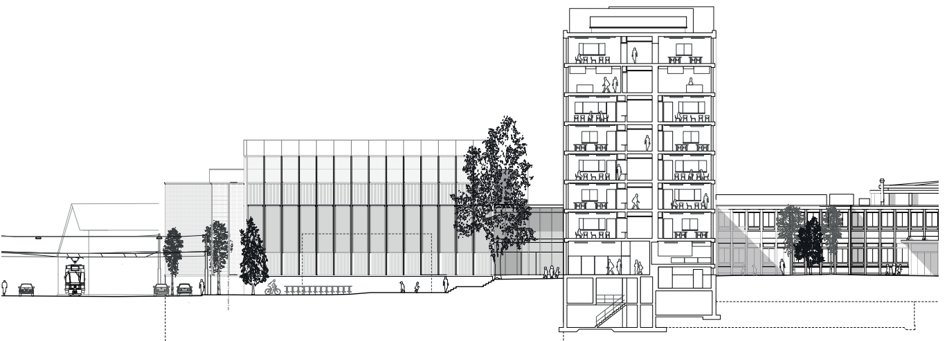
Ansicht Südwest 1:600
