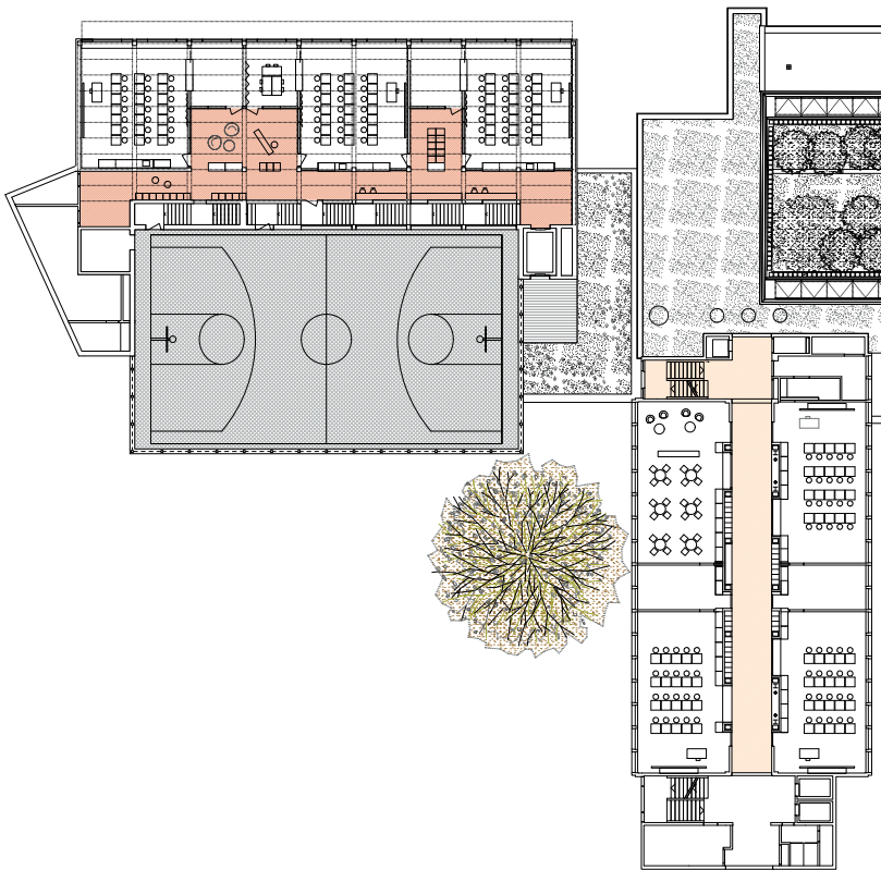
Grundriss 2. Obergeschoss 1:600
