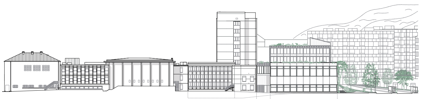
Ansicht Ost 1:1000
