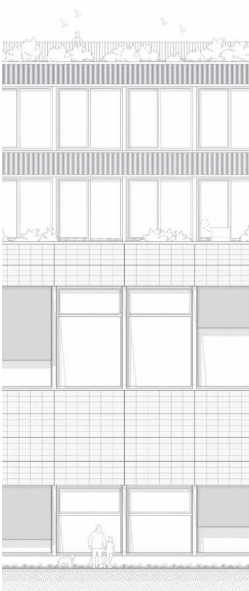
Konstruktionsschnitt und Ausschnitt Fassade 1:150
