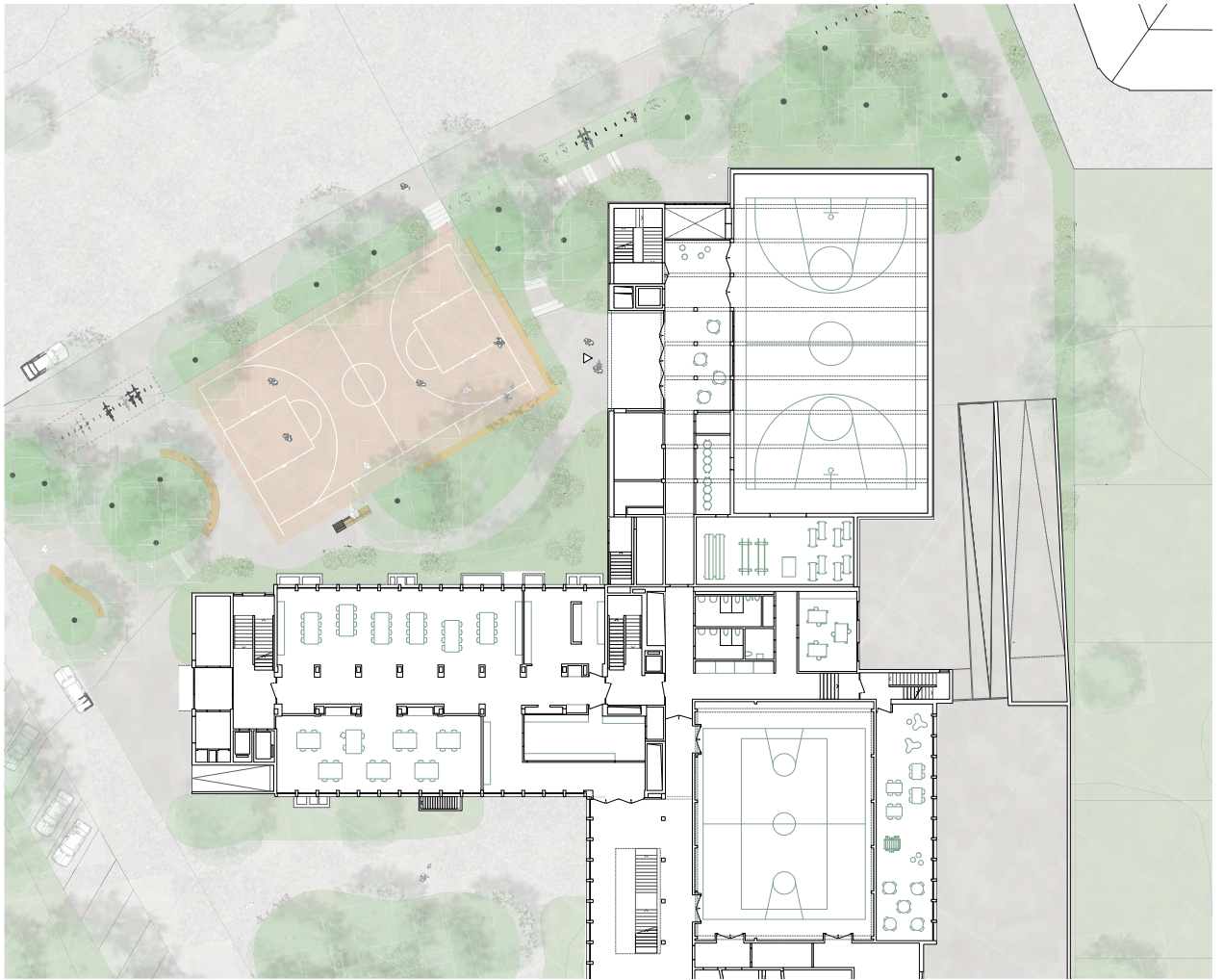
Grundriss Erdgeschoss 1:600
