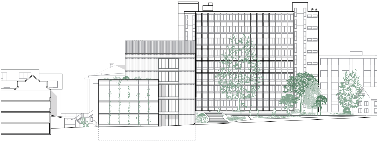
Ansicht Nord 1:600
