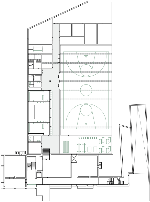
Grundriss 2. Untergeschoss 1:600
