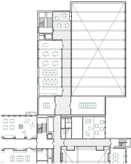
Grundriss 1. Obergeschoss 1:600
