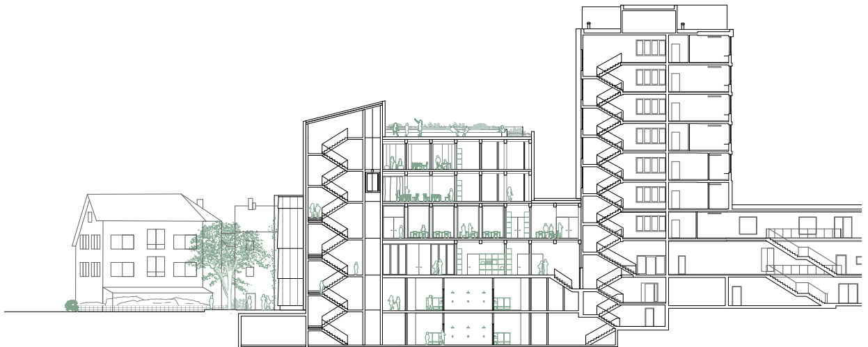
Längsschnitt 1:600
