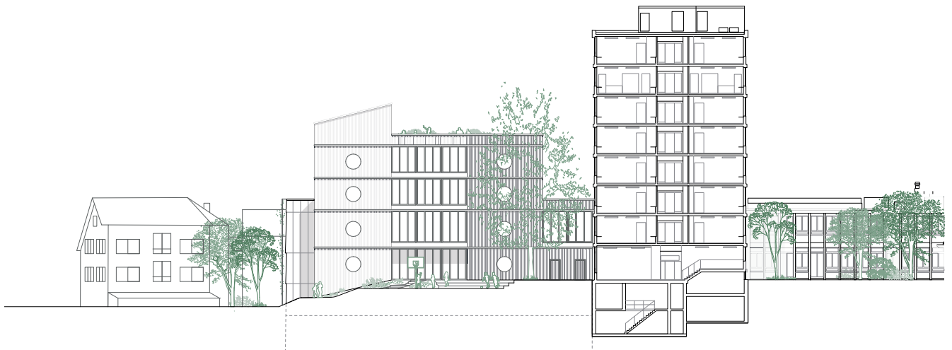
Ansicht West 1:600
