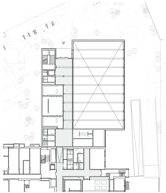
Grundriss 1. Untergeschoss 1:600
