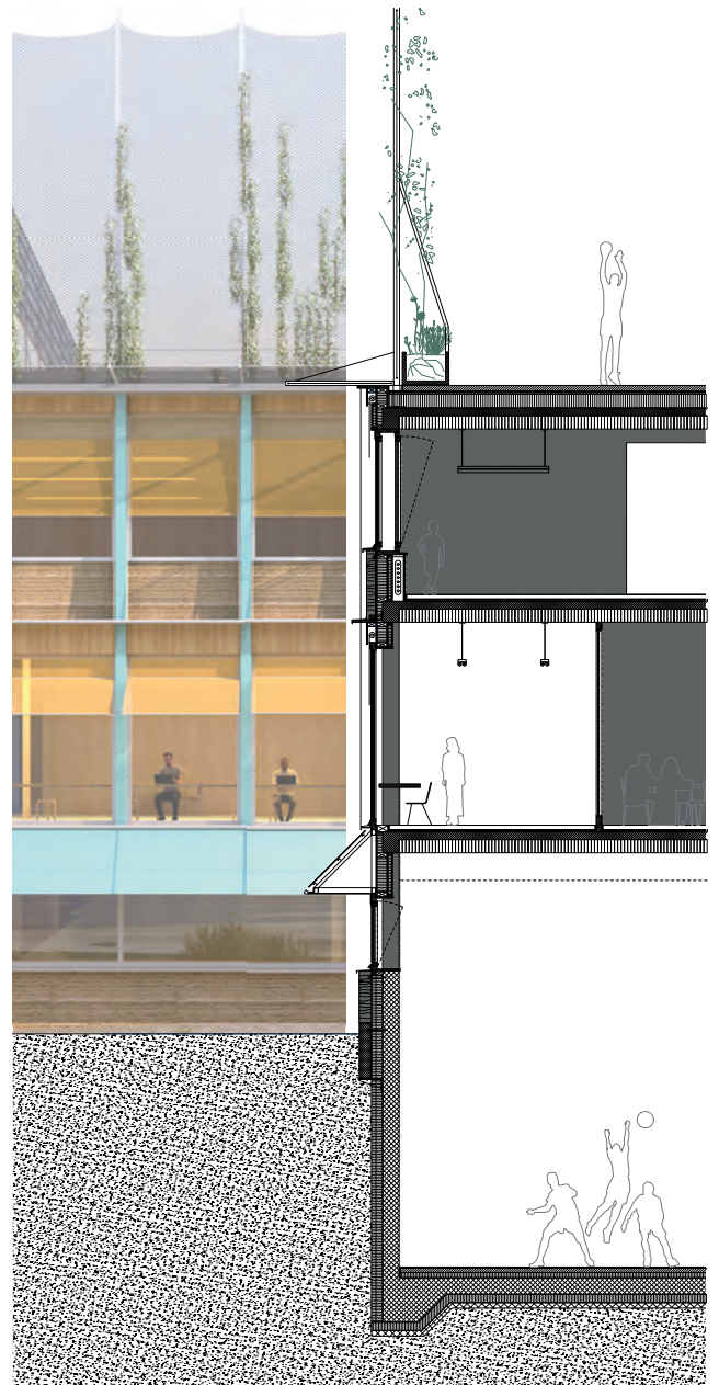
Konstruktionsschnitt und Ausschnitt Fassade 1:150
