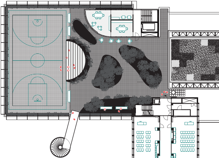
Grundriss Dachgeschoss 1:600
