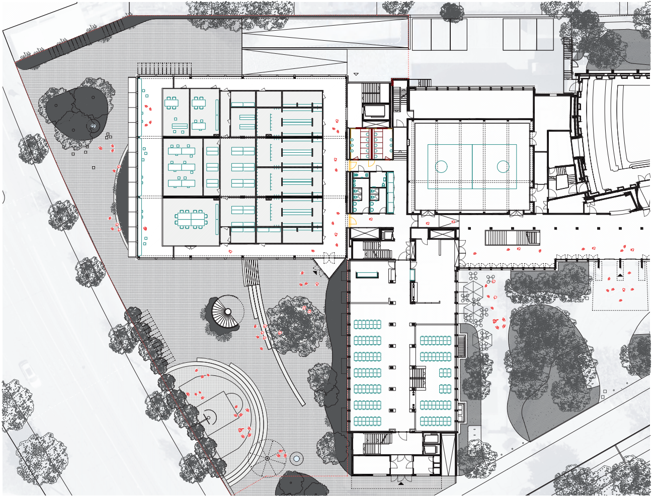
Grundriss Erdgeschoss 1:600
