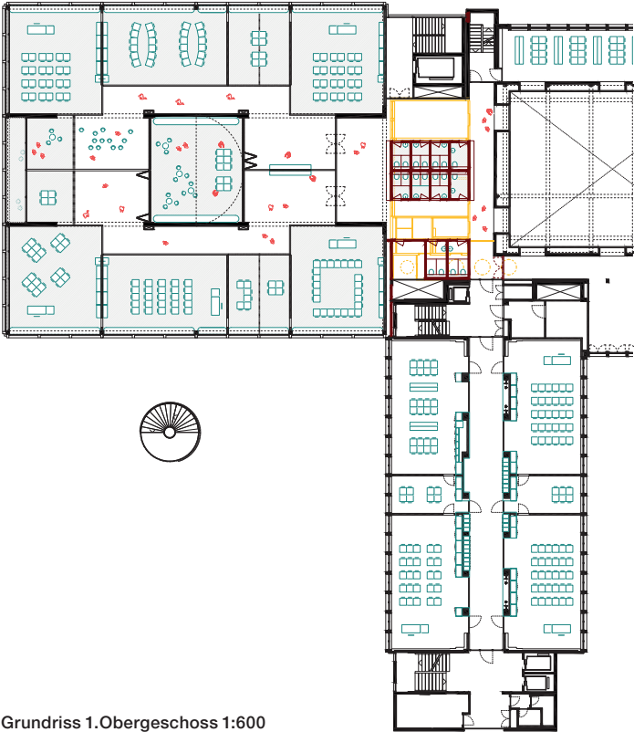
Grundriss 1. Obergeschoss 1:600
