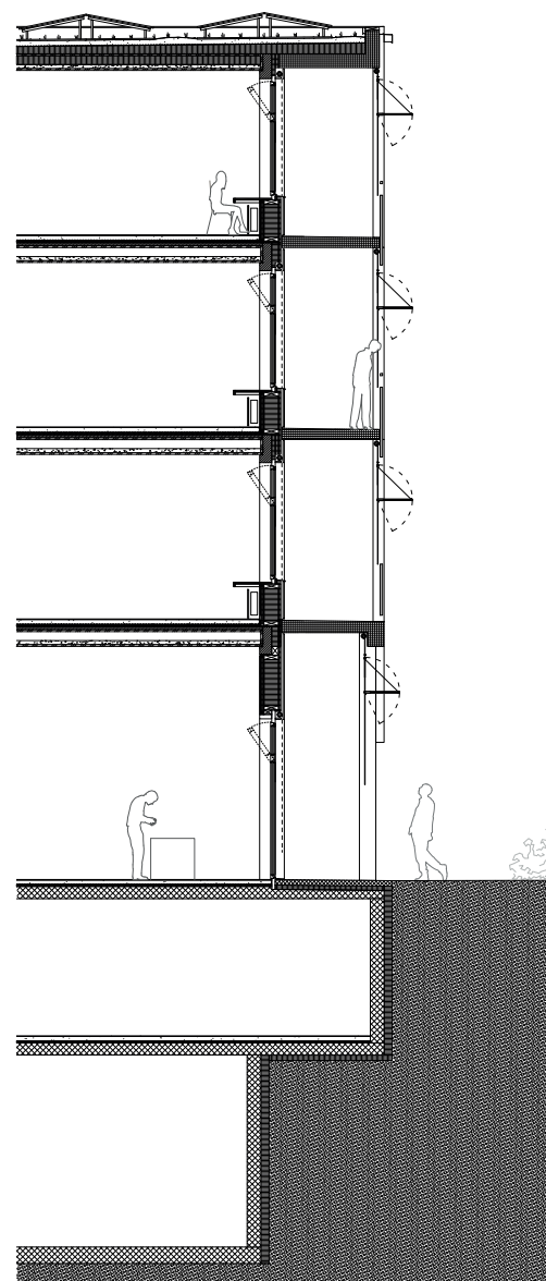
Konstruktionsschnitt und Ausschnitt Fassade 1:150
