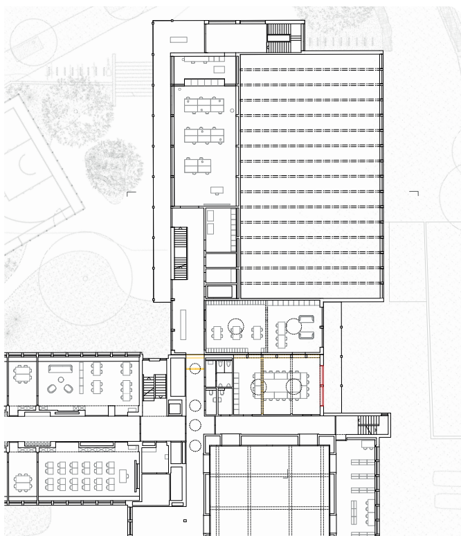
Grundriss 1. Obergeschoss 1:600
