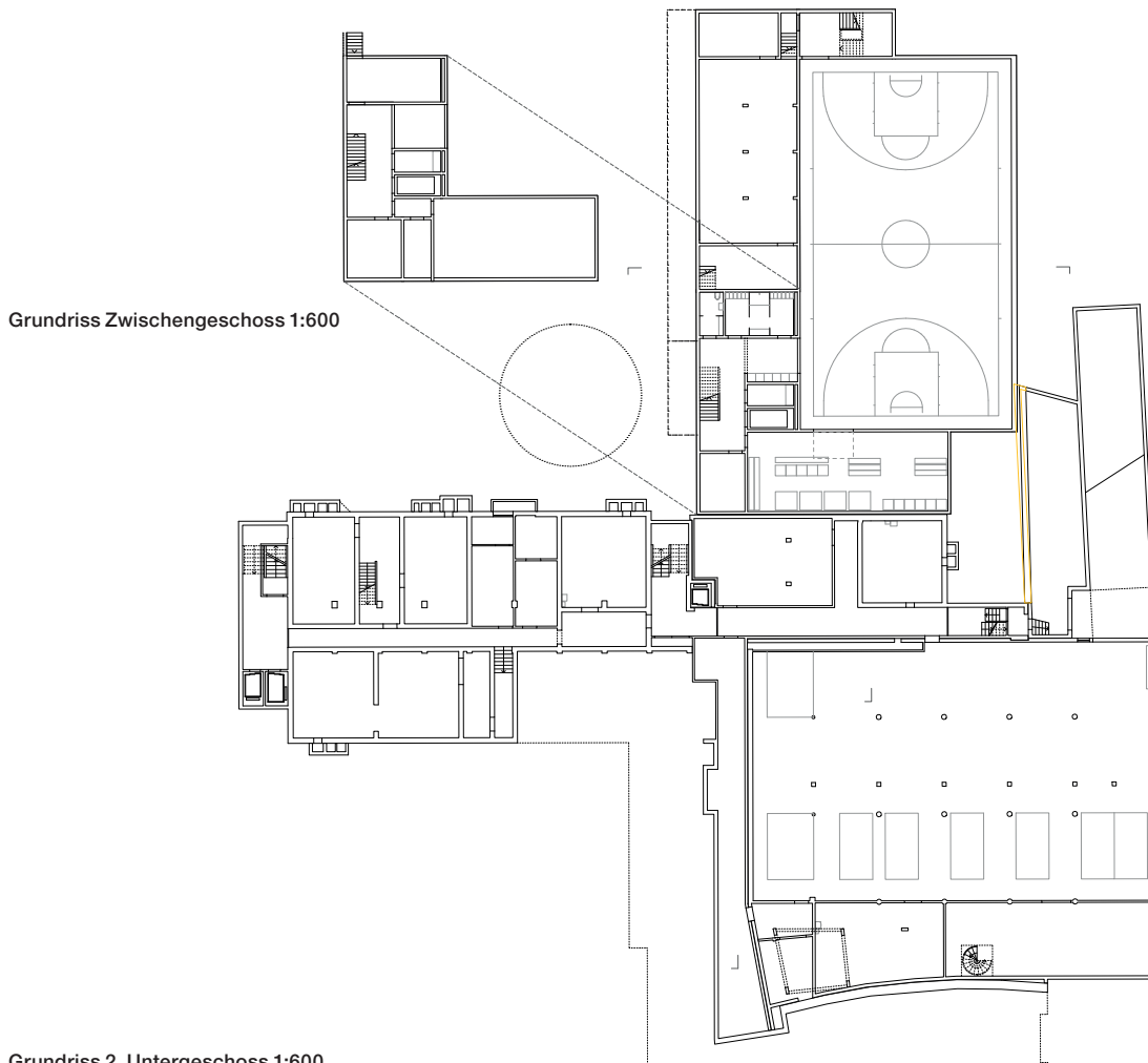
Grundriss 2. Untergeschoss 1:600
