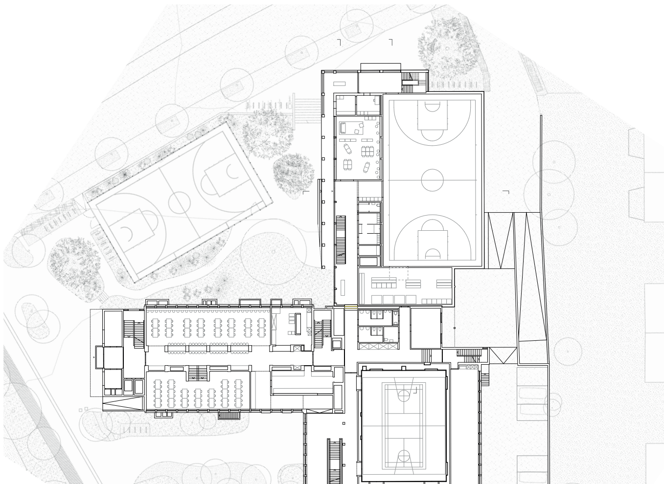
Grundriss Erdgeschoss 1:600
