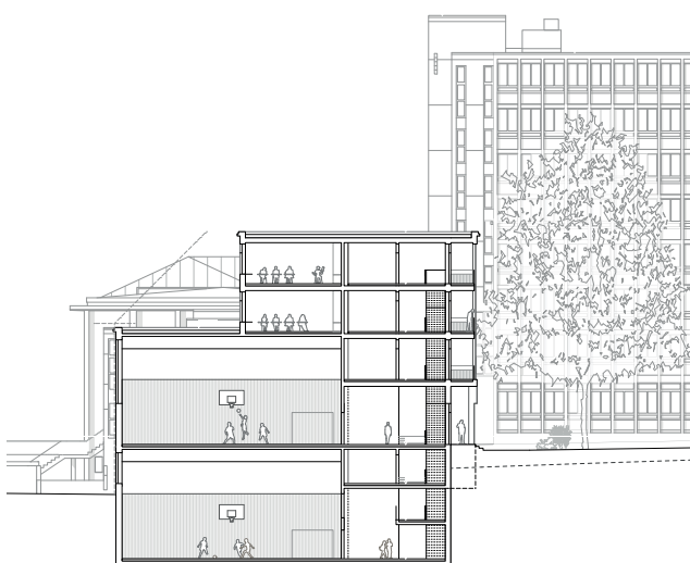
Querschnitt 1:600
