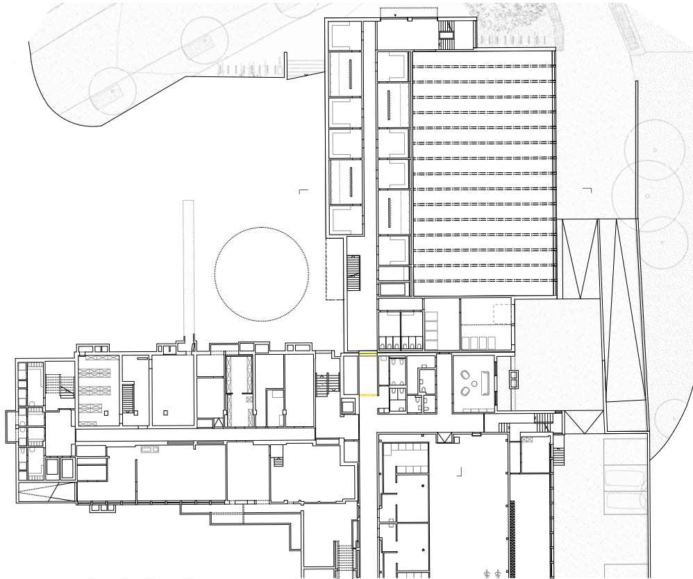
Grundriss 1. Untergeschoss 1:600
