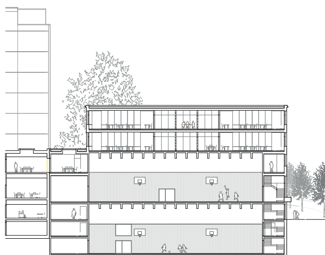
Längsschnitt 1:600
