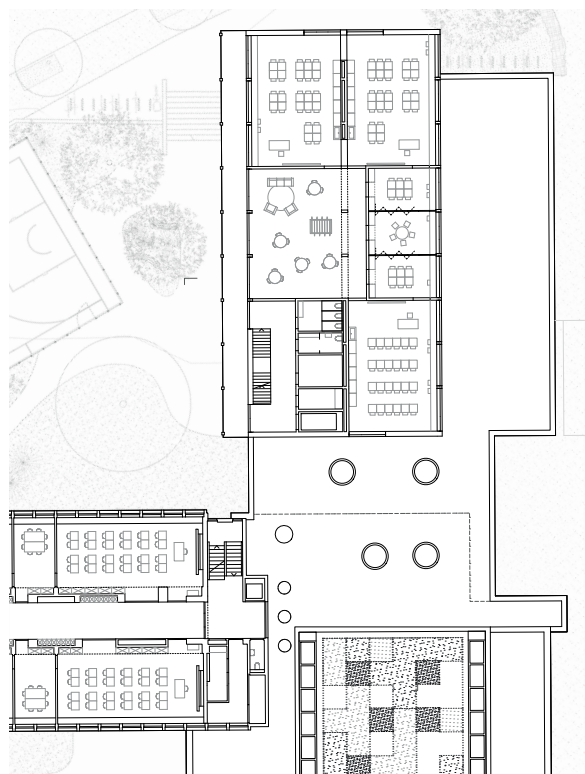
Grundriss 2. und 3. Obergeschoss 1:600
