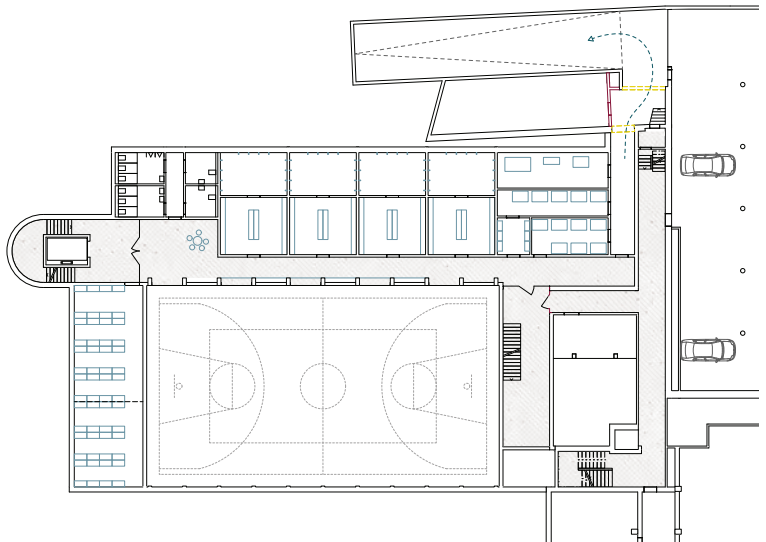
Grundriss 1. Untergeschoss 1:600
