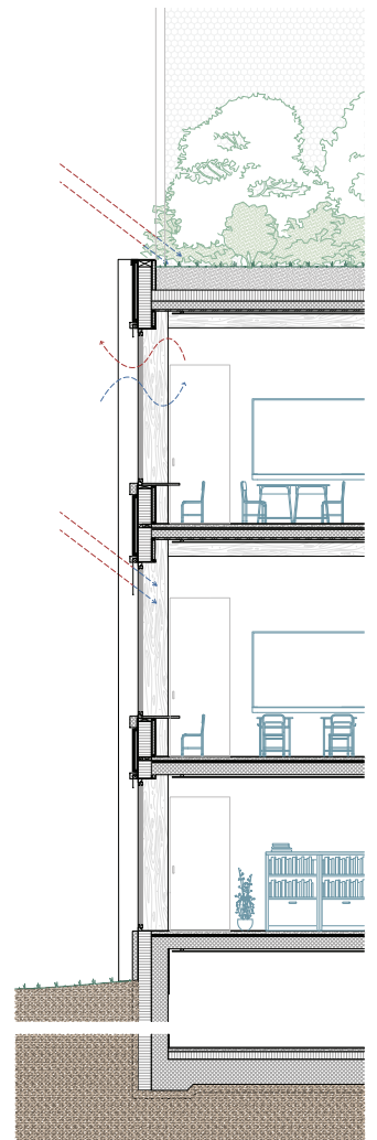
Konstruktionsschnitt 1:150
