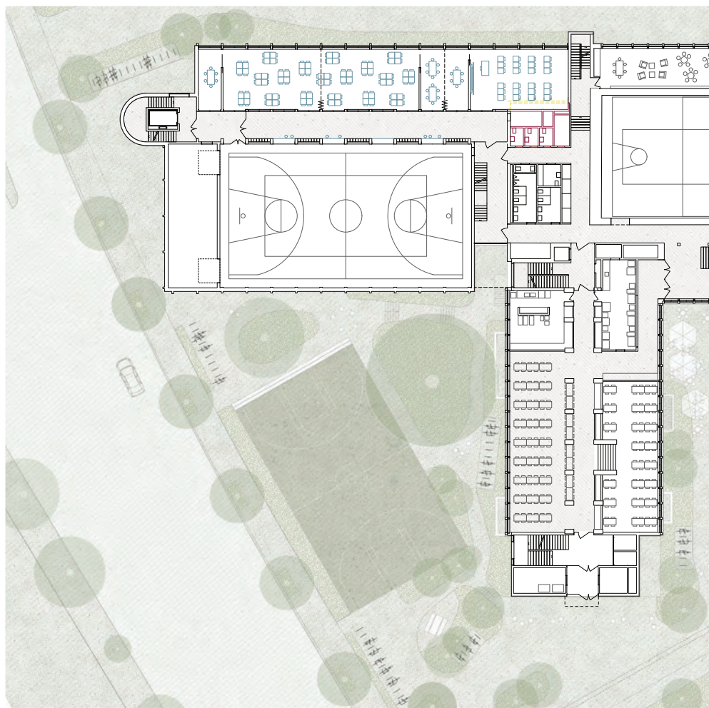
Grundriss 1. Obergeschoss mit Umgebung 1:600
