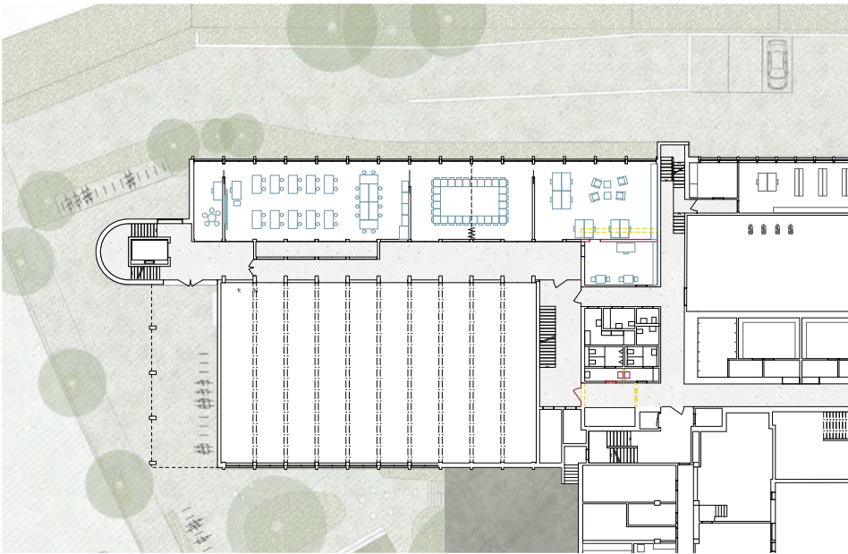
Grundriss Erdgeschoss 1:600
