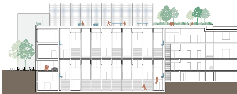
Längsschnitt 1:600
