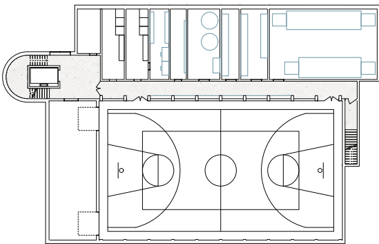
Grundriss 2. Untergeschoss 1:600
