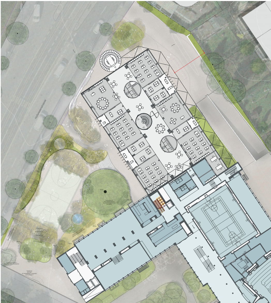
Grundriss 1. Obergeschoss 1:600
