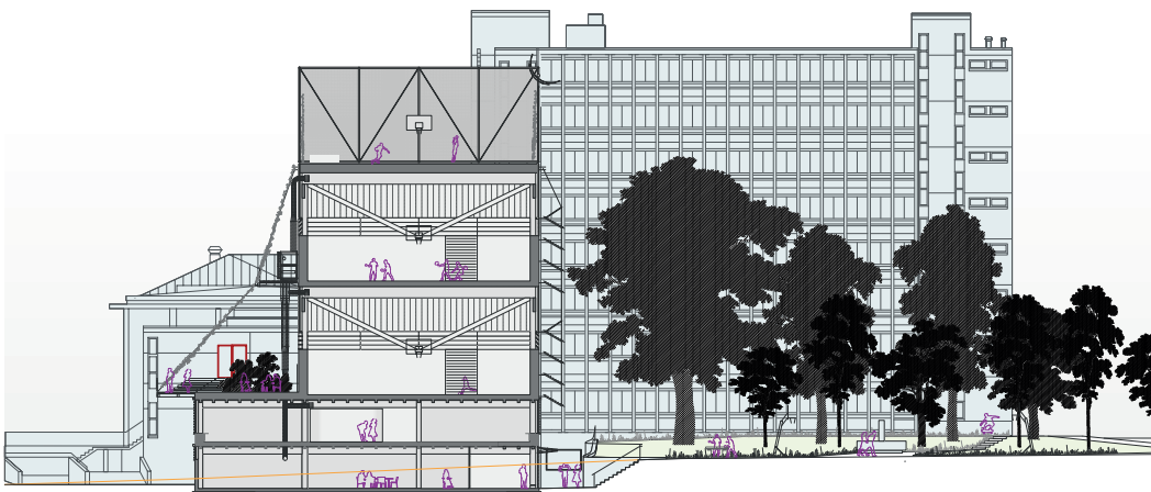
Querschnitt 1:600
