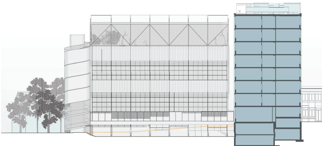
Ansicht Südwest 1:600
