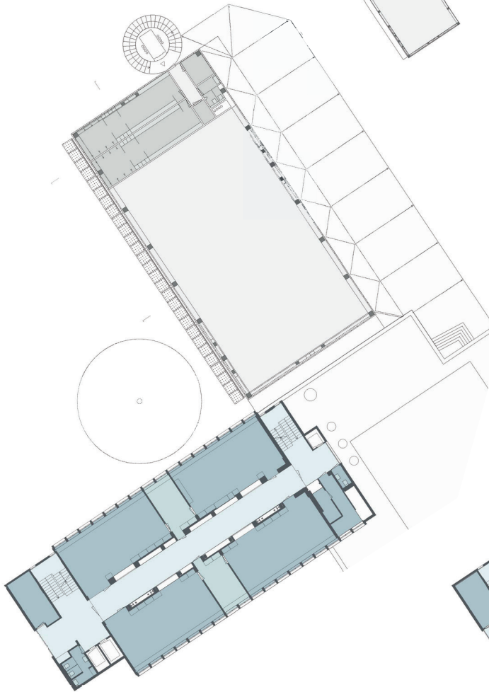
Grundriss 3. Obergeschoss 1:600
