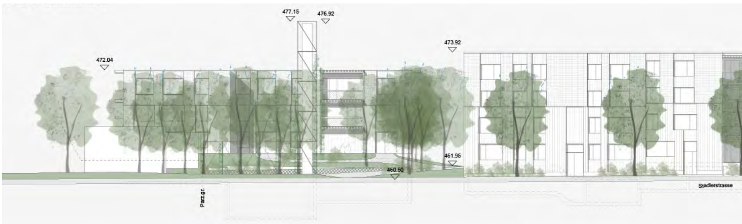
Baubereich N: Ansicht Westfassade / Grabenackerstrasse, 1:200 (verkleinerte Darstellung)
