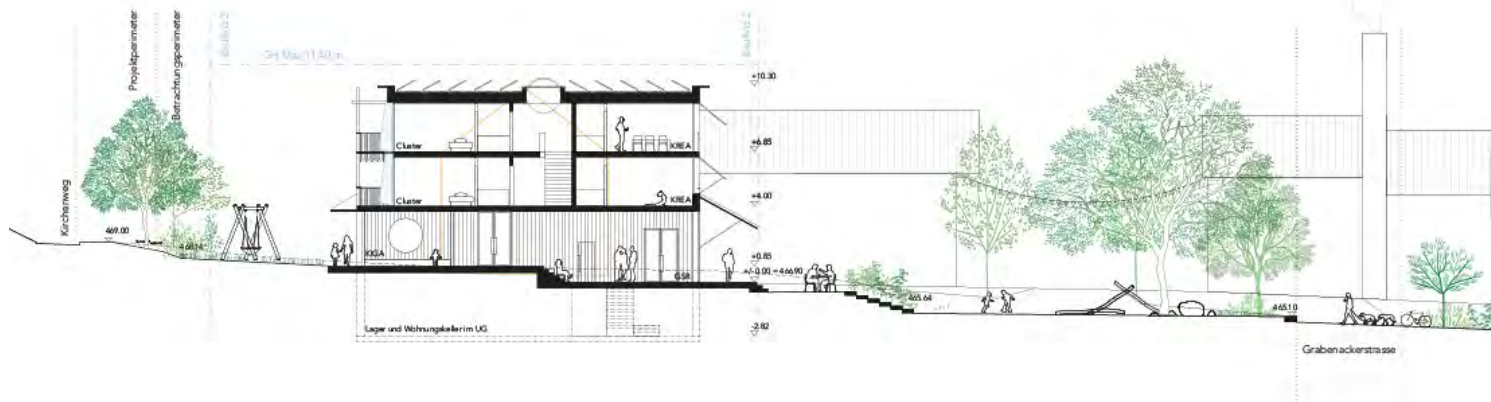
Baubereich Z und S1: Querschnitt West-Ost, 1:200 (verkleinerte Darstellung)
