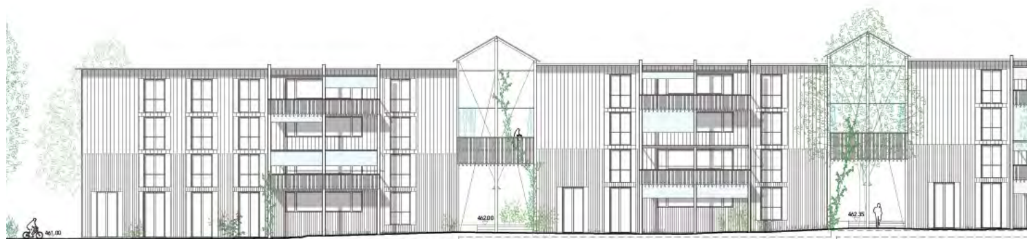
Baubereich S1: Ansicht Ostfassade / Stadlerstrasse, 1:200 (verkleinerte Darstellung)
