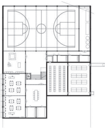
1. Untergeschoss
