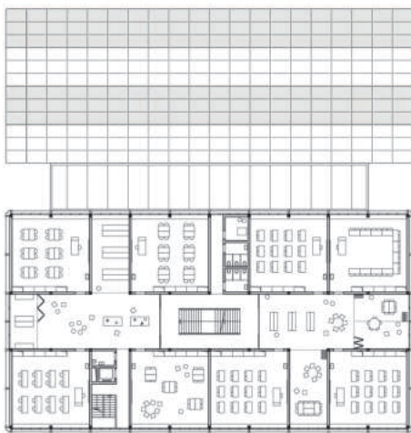
1. Obergeschoss
