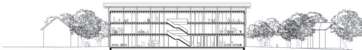
Schnitt A
