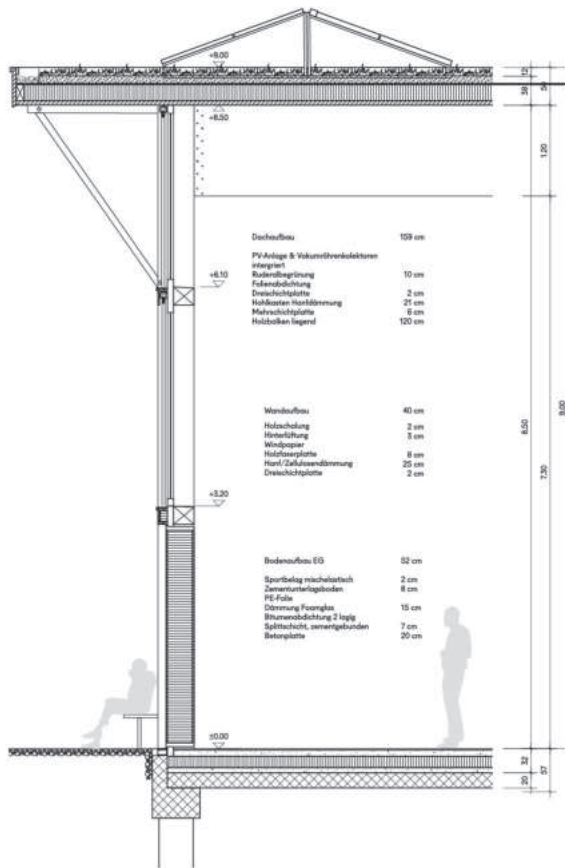
Fassade Sporthalle
