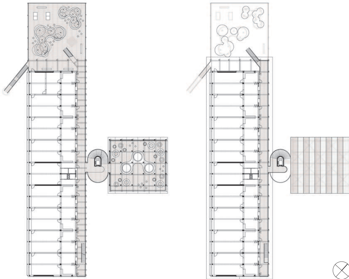
1. Obergeschoss
