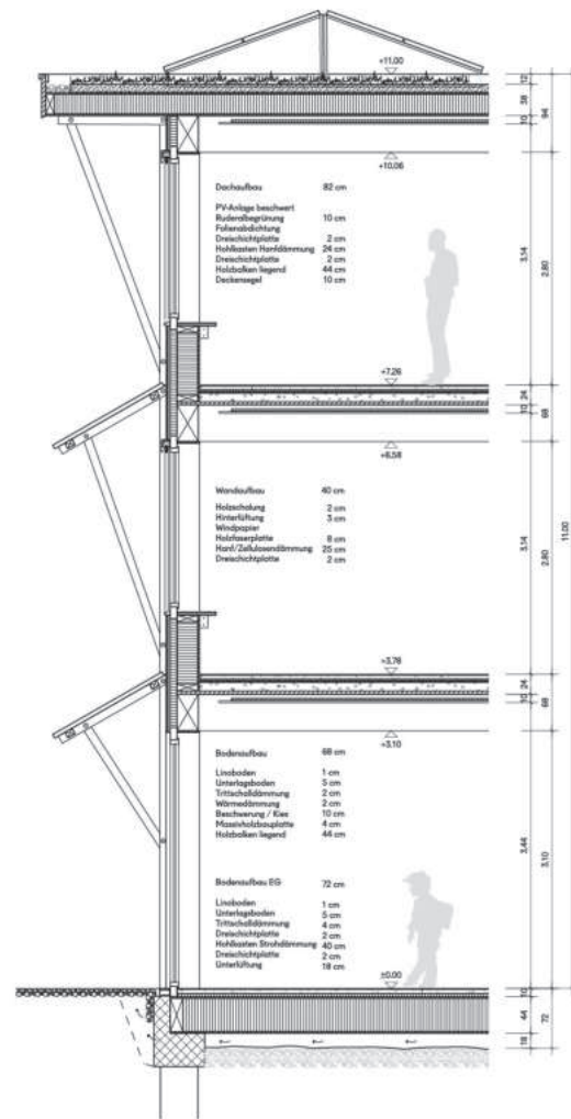
Fassade Schulhaus
