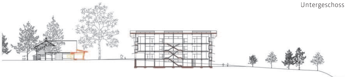
Längsschnitt Schulhaus
